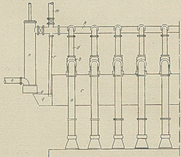
Abb. 2. Füllgasabsaugvorrichtung.
