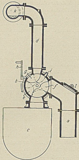
Abb. 1. Schnitt durch das Gaswechselventil.
