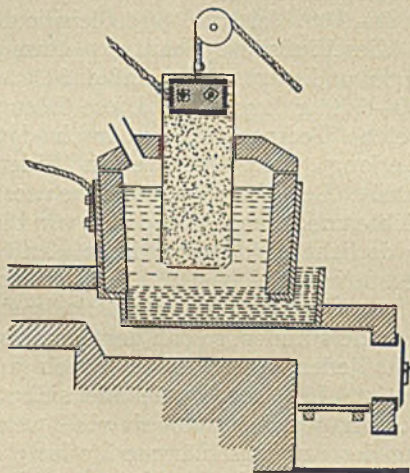
Abb. 1. Elektrischer Bleiofen von Kern.
