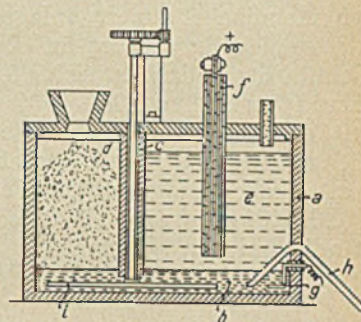
Abb. 2. Elektrischer Bleiofen von Auerbach.
