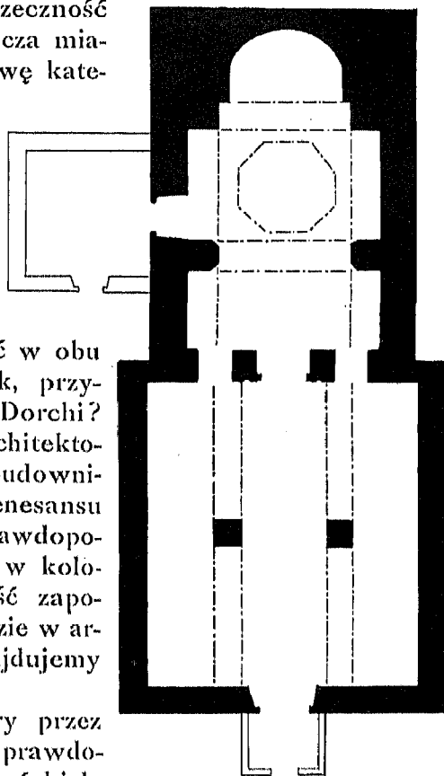
17. Kaffa, kościół ormiański św. Jana Chrzciciela. Rzut poziomy. Zdjęcie N. S. Barsamowa w Teodozji.
