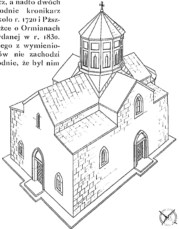
11. Lwów, katedra ormiańska. Odtworzenie pierwotnego widoku. Zdjęcie Inst. Archit. Polsk. Polít. Lwowsk.
