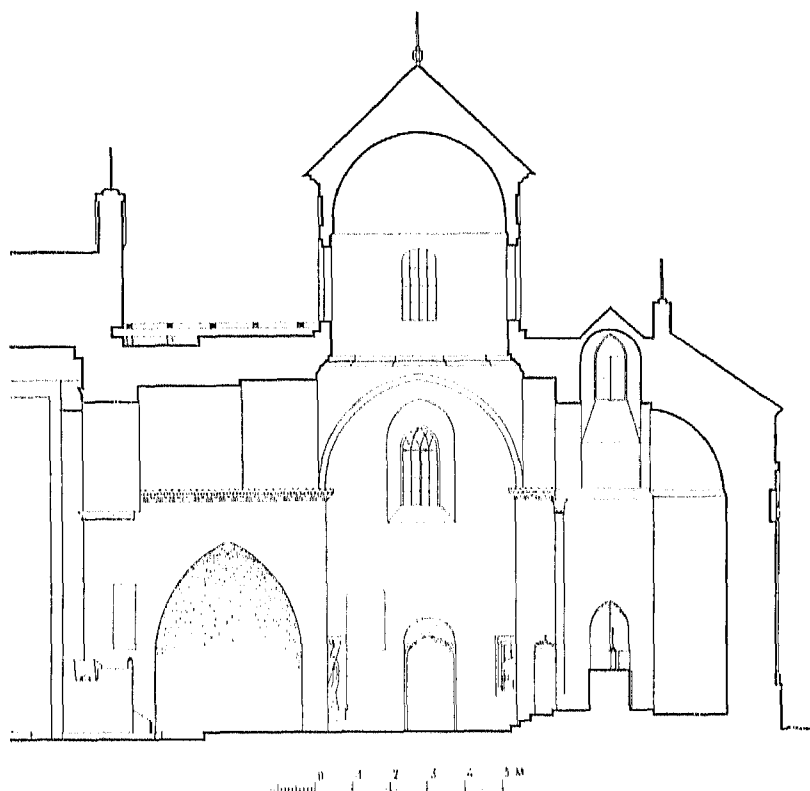
9. Lwów, katedra ormiańska. Przekrój podłużny.
