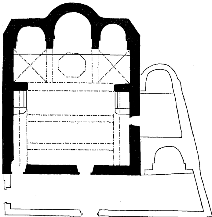
21. Kaffa, kościół ormiański śś. Gabrjela i Michała. Rzut poziomy. Zdjęcie N. S. Barsamowa w Teodozji.
