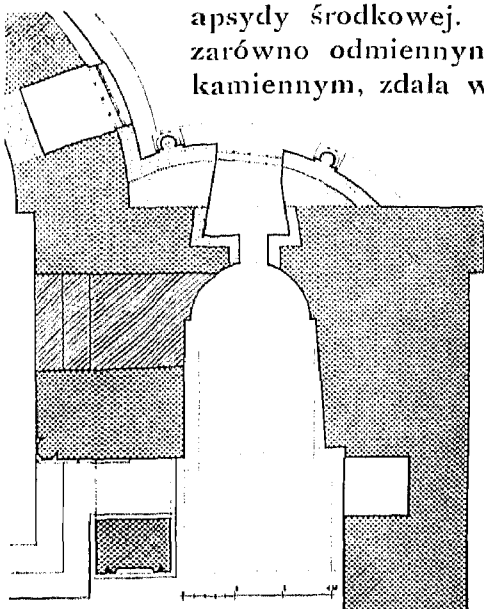
8. Lwów, katedra ormiańska. Rzut poziomy murów bocznej apsydy. Zdjęcie Inst. Archit. Polsk. Polít. Lwów.
