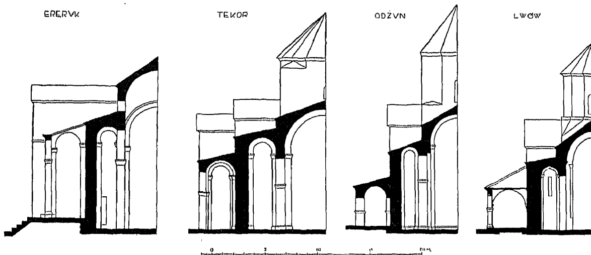
22. Przekroje poprzeczne kościołów ormiańskich w Erewan, Tekor, Odzun i Lwowie.
