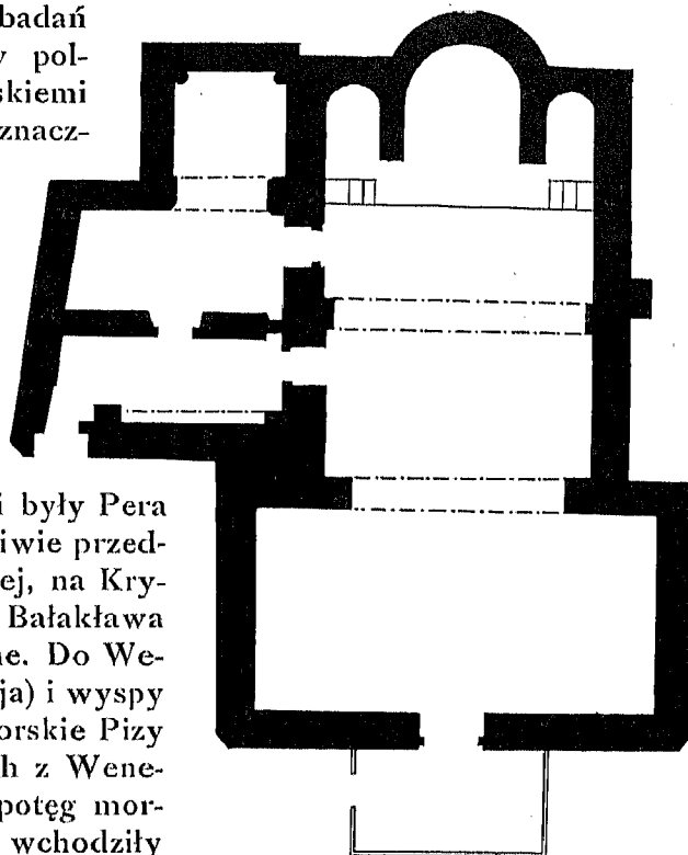
19. Kaffa, Kościół ormiański św. Sergjusza. Rzut poziomy. Zdjęcie N. S. Barsamowa w Teodozji.
