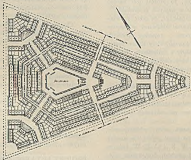
J. J. P. OUD. FRAGMENT DZIELNICY TANICH MIESZKAŃ W ROTTERDAMIE.
