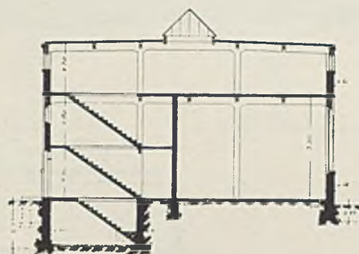
Przekrój C — D.
