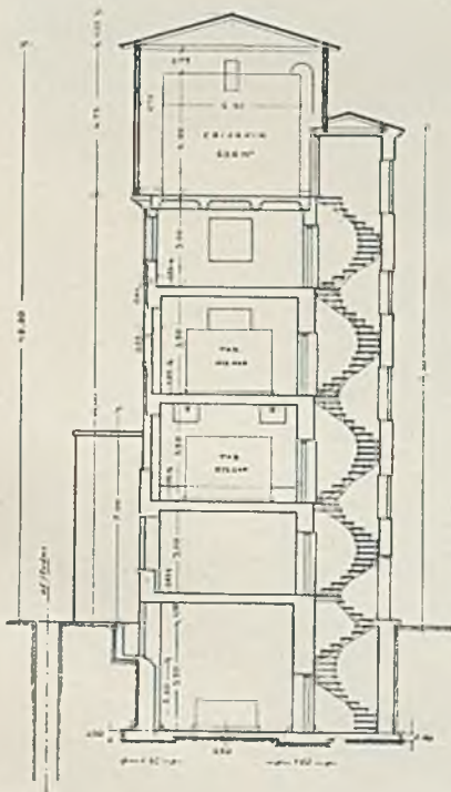
Przekrój A—B.
