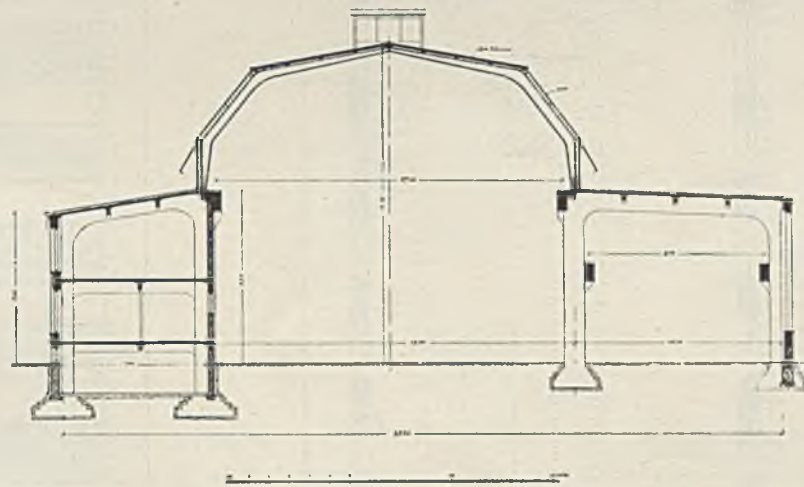
Przekrój poprzeczny.
