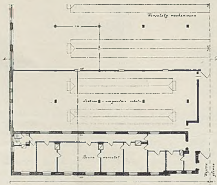
Rzut poziomy.
