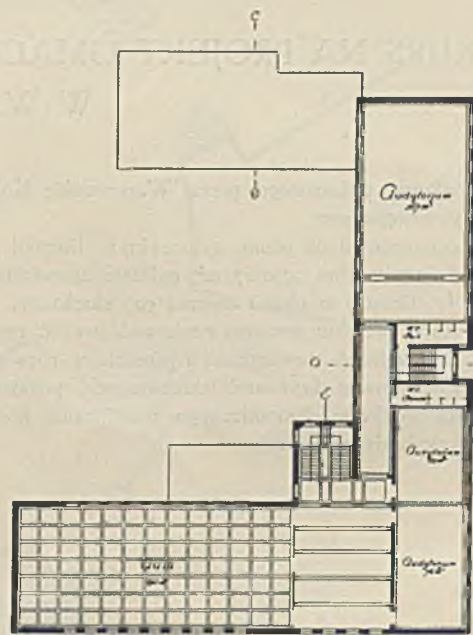
Plan 2 ty piętra
