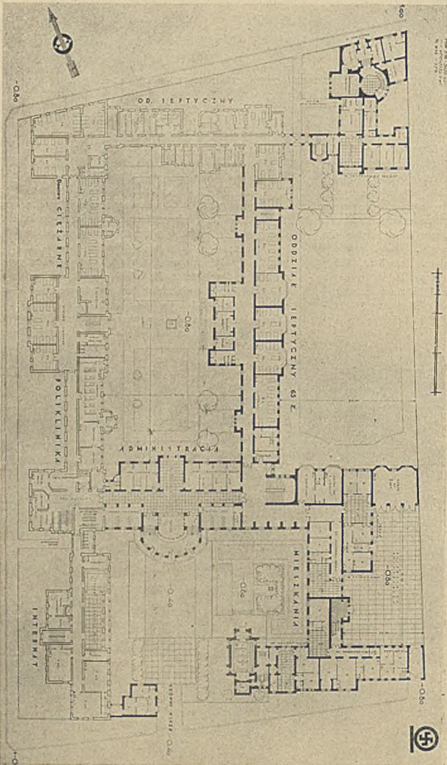
Rzut parteru.
