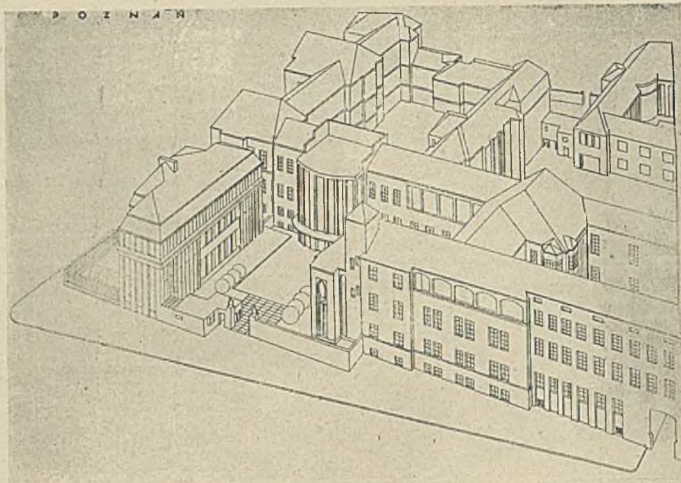
ARCH. CZESŁAW PRZYBYLSKI (WARSZAWA). PROJEKT ROZBUDOWY KRAJOWEJ KLINIKI POŁOŻNYCH W POZNANIU. Widok z lotu ptaka.
