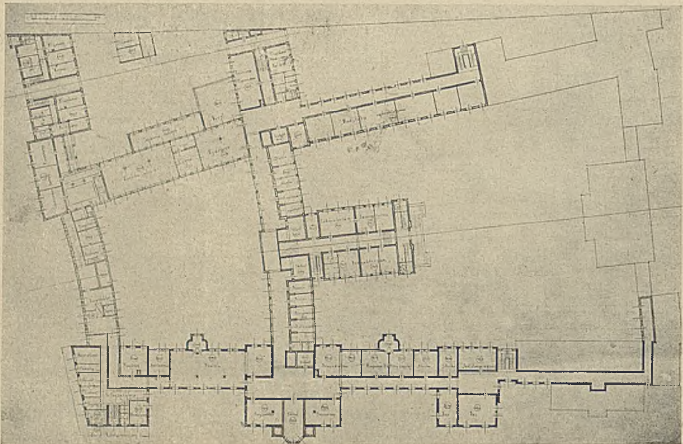
Rzut suteren.
