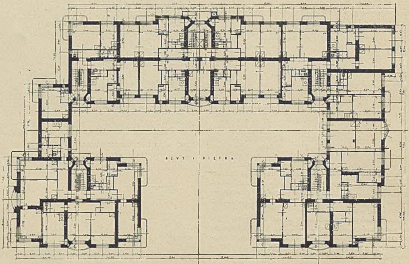
Rzut I piętra w skali 1:400.
