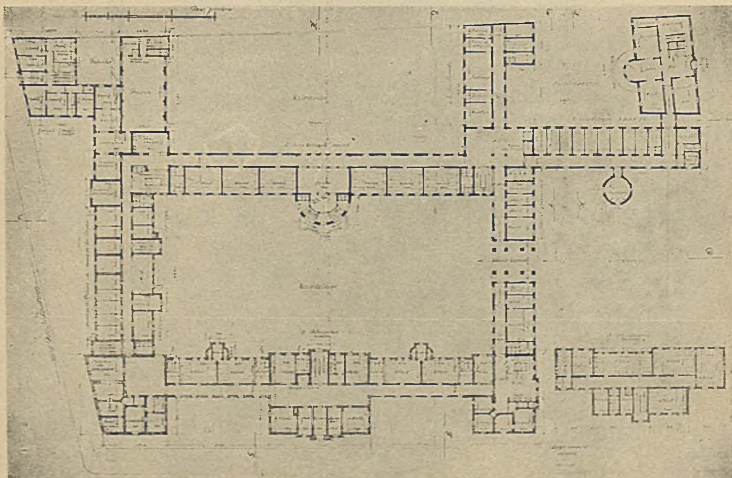
Rzut parteru.
