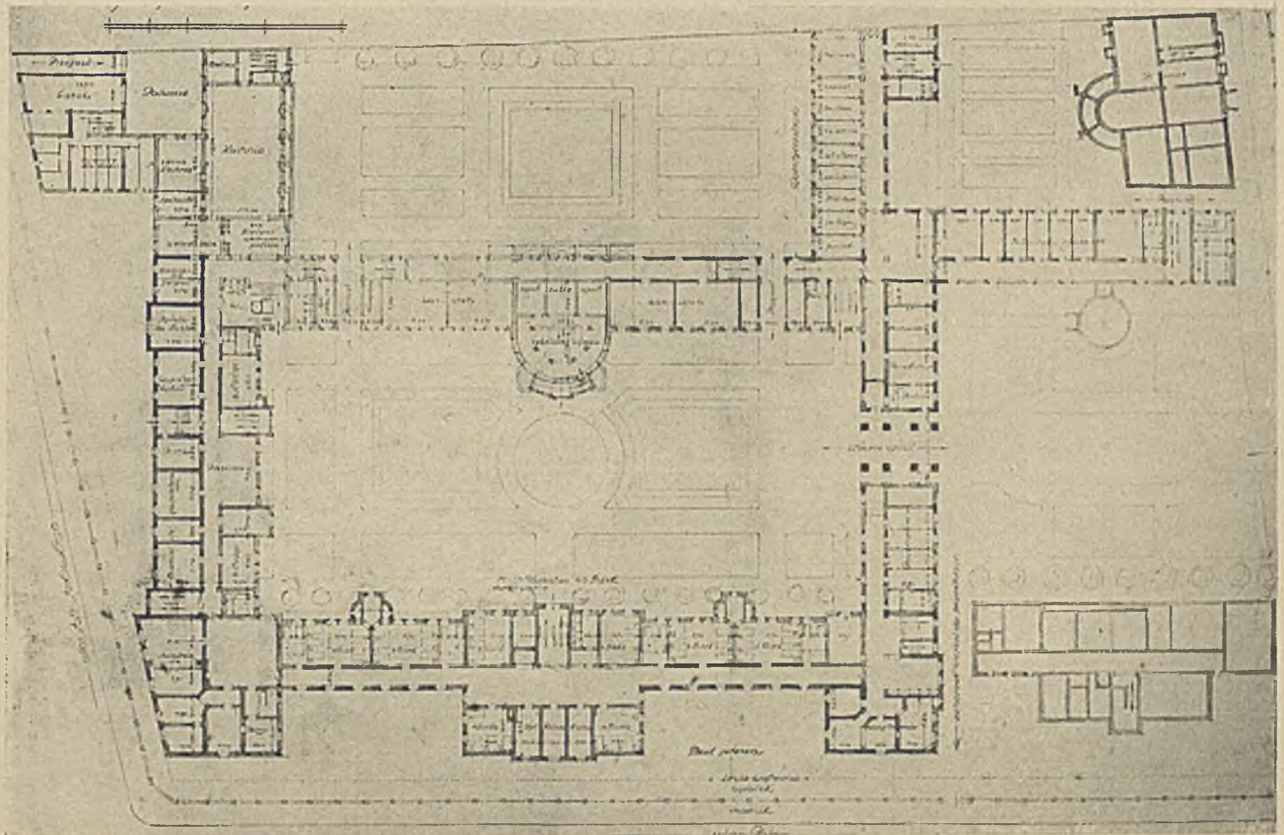
Rzut suteren.
