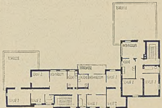
ARCH. JÓZEF FRANK (WIENIĘ). DOM DLA 2-CH RODZIN W OSIEDLU WEISSENHOF W STUTTGARCI.
