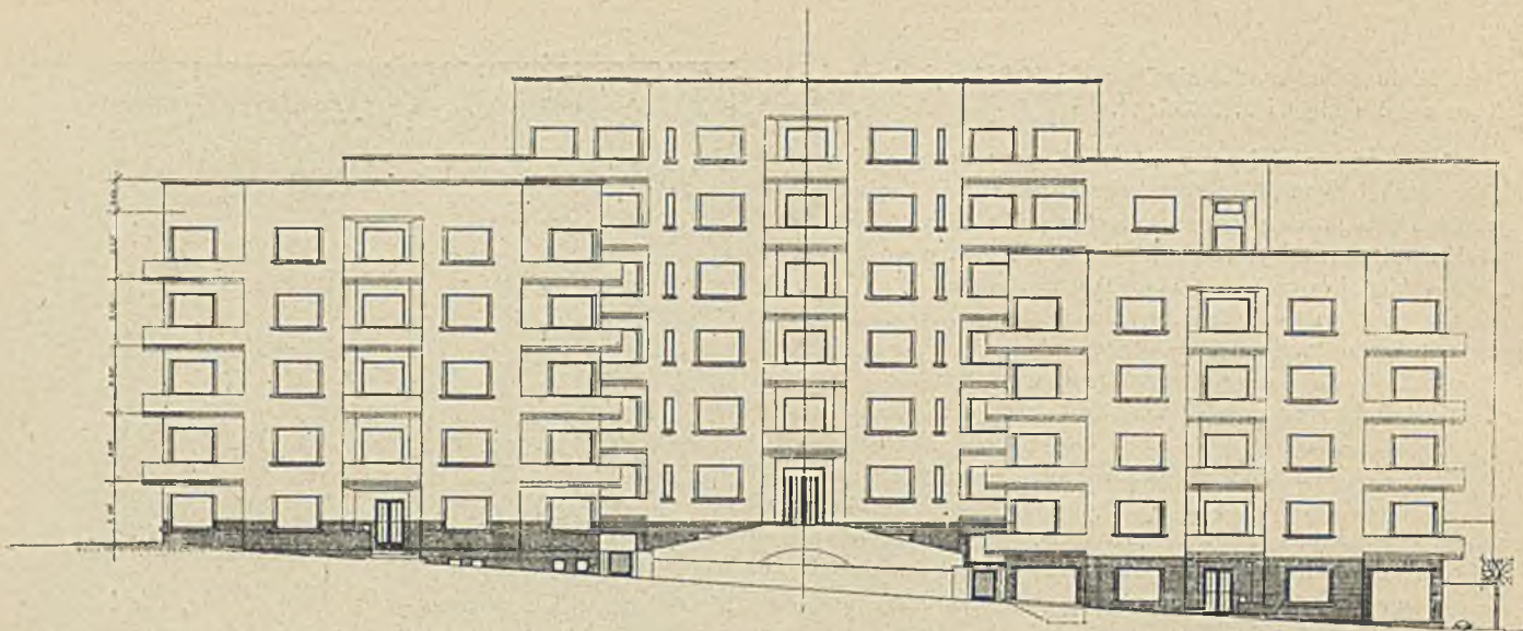
Elewacja od ul. Stryjskiej.
