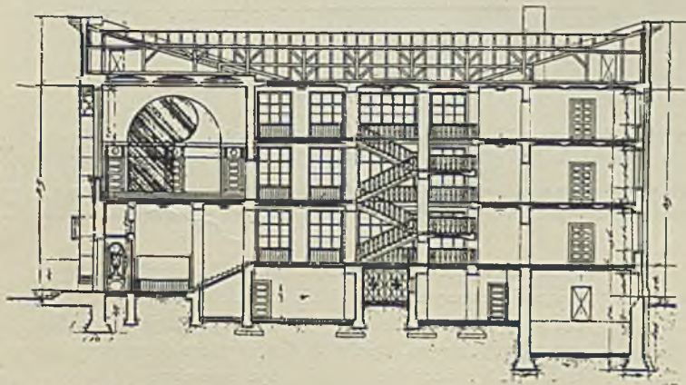
Przekrój A—B.
