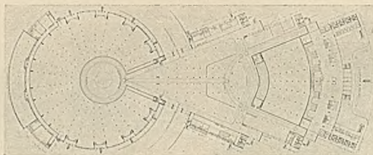
Rzut poziomu I.
