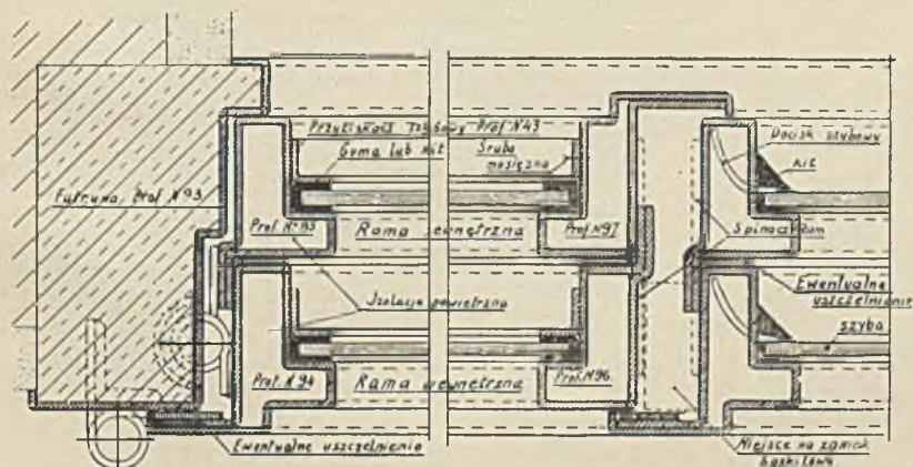
Przekrój poziomy okna szwedzkiego „HAZET-STALOSZWED”
