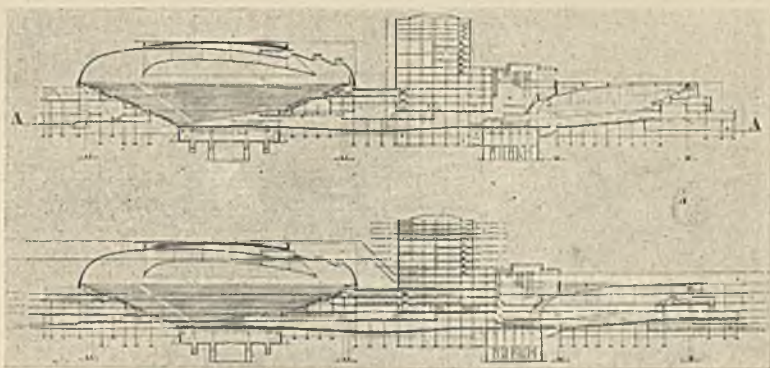
Przekrój podłużny.
