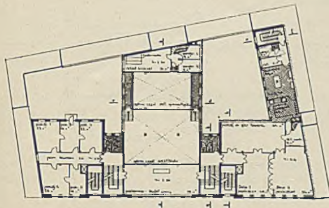
Rzut parteru.
