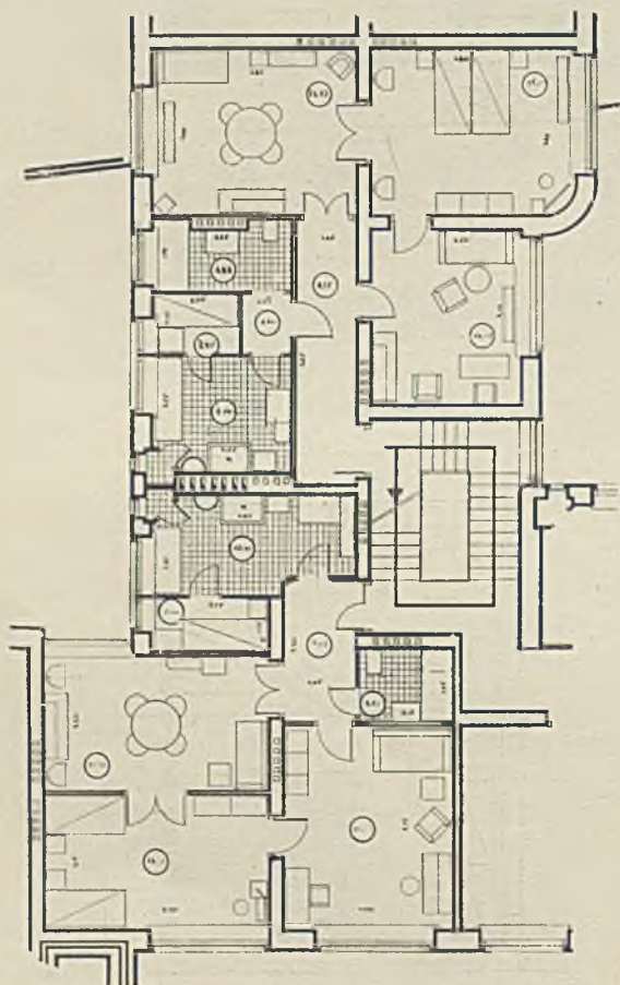
Mieszkanie 3-pokojowe.
