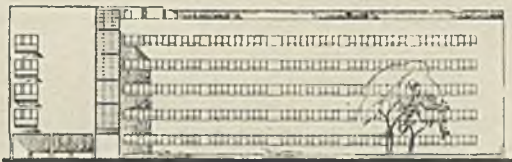
Elewacja południowa.
