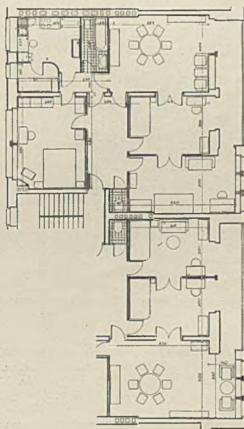
Mieszkanie 4-pokojowe. 1:200
