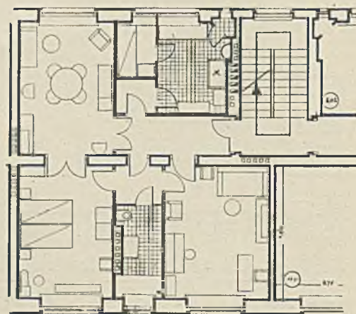
Mieszkanie 3-pokojowe.
