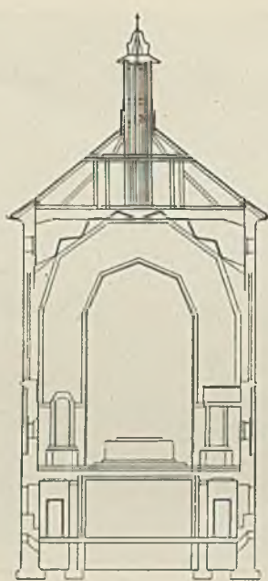
Przekrój poprzeczny
