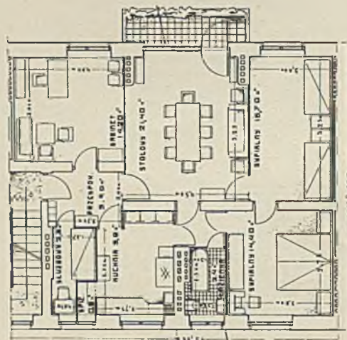
Mieszkanie 4-pokojowe.
