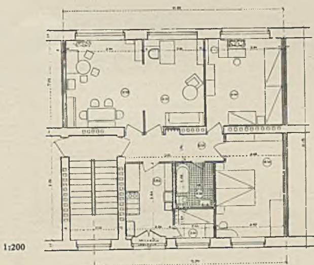
Mieszkanie 4-pokojowe.
