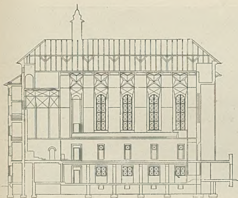
Przekrój podłużny.
