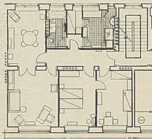
Mieszkanie 4-pokojowe.
