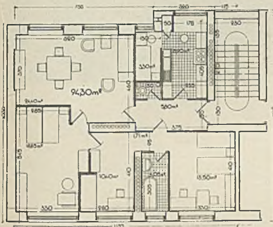
Mieszkanie 4-pokojowe.
