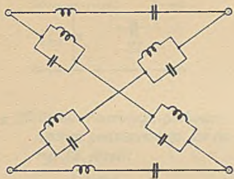
Rys. 16. Przykład filtra kratowego.
