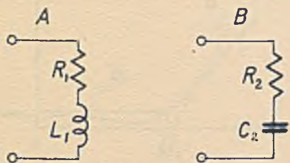
Rys. 5. Dwojniki A i B są sprzężone dla częstotliwości f = \frac{1}{2\pi\sqrt{L_1 C_2}} , gdy R_1 = R_2 .
