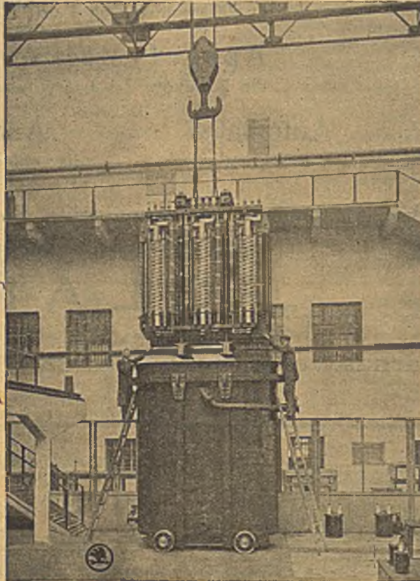
Transformator 17. 500 KVA, 6.300/22.000 volt, 50 okresów, dostarczony do Elektrowni Miejskiej w Pradze Czeskiej.
