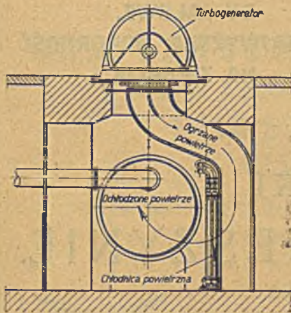
Chłodnica powietrzna typu G e a
