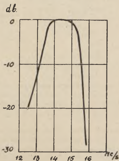
Rys. 7. Rezonansowa charakterystyka anteny
