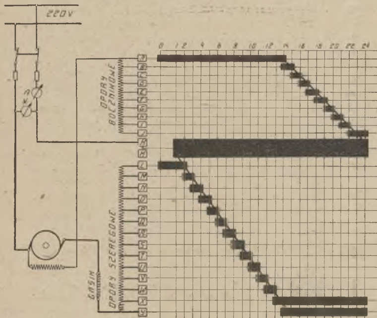
Rys. 2. Plan połączeń silnika bocznikowego z regulacją obrotów przez włączanie oporów i osłabianie pola magnetycznego.
