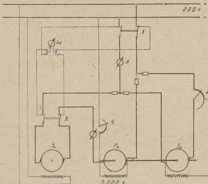
Rys. 3. Regulacja obrotów silnika przez połączenie posobno i przeciw sobne.
