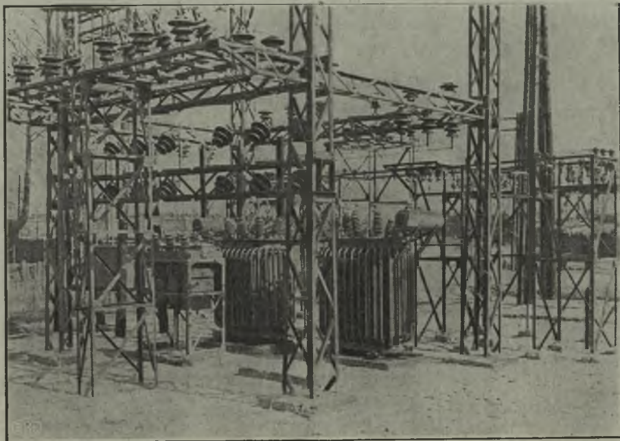
Transformatory 320 kVA 31,5/6,3/0,4 kV. w podstacji napowietrznej (Zjedn. Elektr. Okr. Rad.-Kiel. S. A.)
