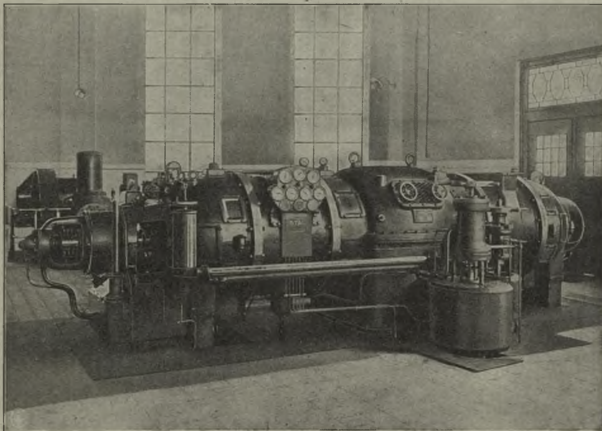
TURBINA PRZECIWPREŻNA STAL O MOCY 2 100 kW.
