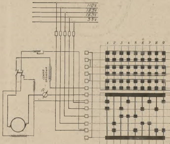
Rys. 8. Plan połączeń silnika bocznikowego prądu stałego przy systemie pięcioprzewodowym.
