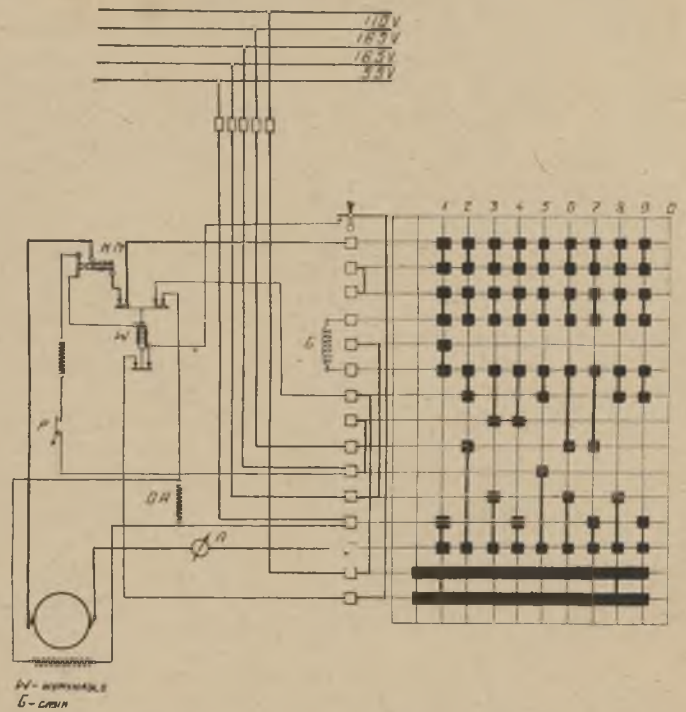
Rys. 9. Plan połączeń silnika bocznikowego z łącznikiem samoczynnym nadmiarowym przy sieci pięcioprzewodowej.
