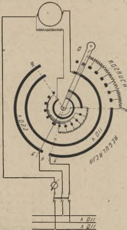
Rys. 4. Regulacja obrotów silnika bocznikowego przez włączanie twornika na dwa napięcia.
