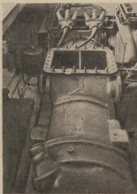
Rys. 2. Tenże skraplacz po naprawie własnymi siłami (wyprostowano płaszcz i wstawiono łąty)
