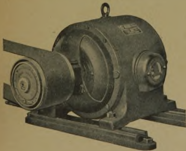
Rys. 5. Silnik krótkozwarty z odśrodkowym sprzęgłem rozruchowym „Skoda - Götz” o mocy 35 kW, 1460 obr., 380/220 V. (Skoda).
