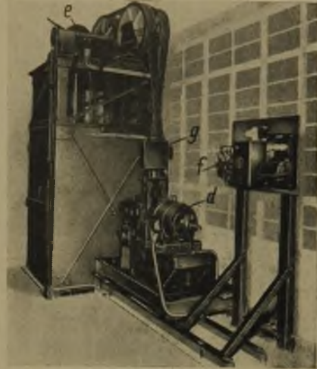
Rys. 4. Dźwig ze sterowaniem mechanicznym; d — silnik, e — rozrusznik, f — wyłącznik pomocniczy, g — elektromagnes.
