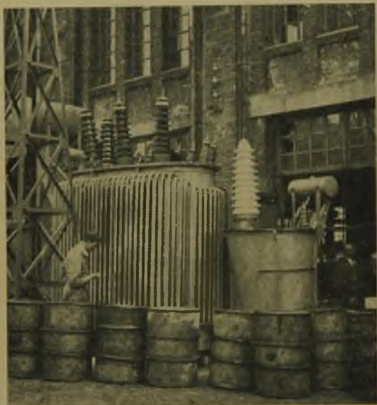
Rys. 1. Transformator trójzwojowy 3 000 kVA, 60 000/15 500/6 400 V w czasie próby napięciowej (Elektrobudowa).
