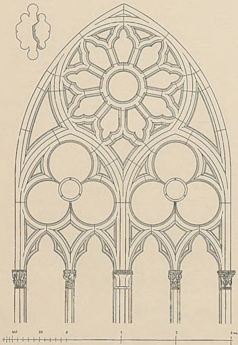
15. Ostfenster des Domes in Breslau. 1 : 40.
