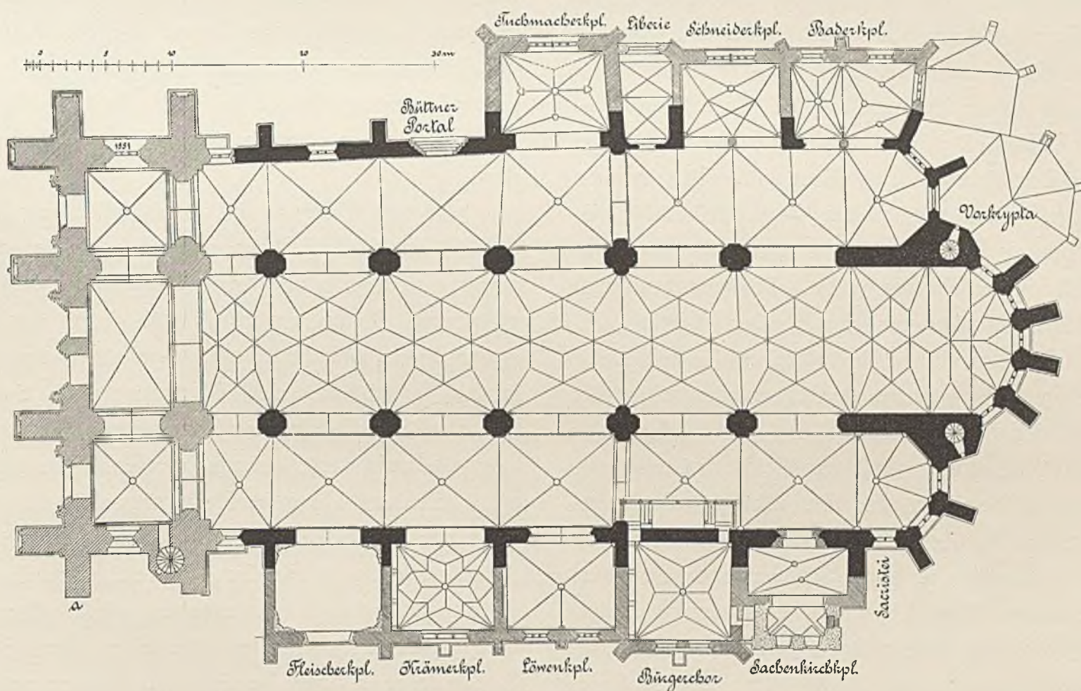
21. Grundriss der Katholischen Pfarrkirche in Schweidnitz.
