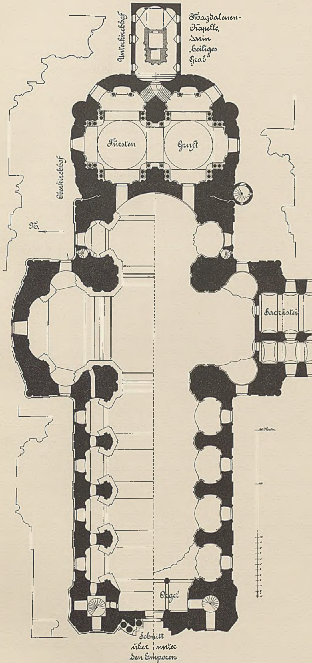
67. Grundriss und Profile der Klosterkirche in Grüssau.
