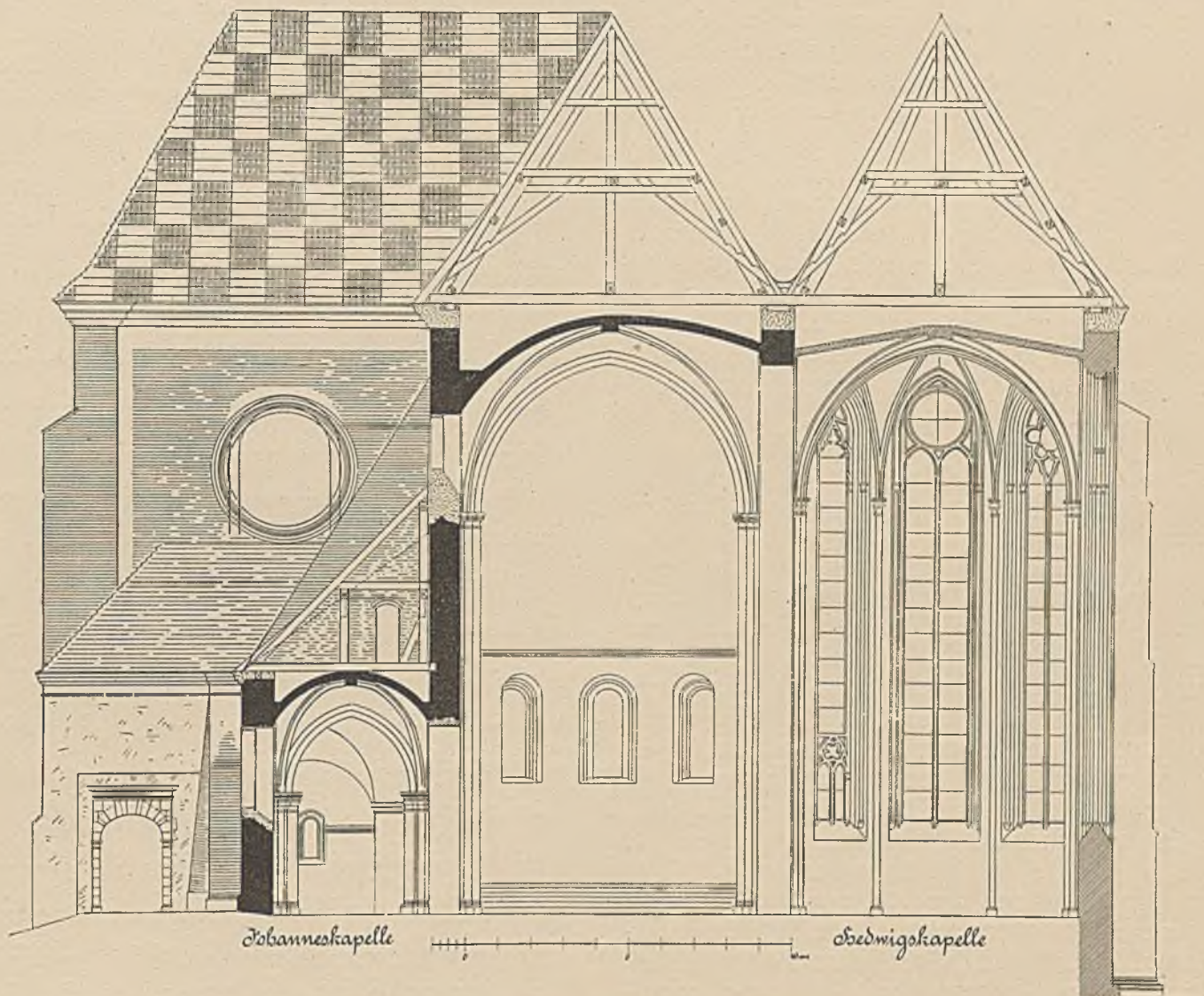
2. Idealschnitt durch die Klosterkirche in Trebnitz und die Hedwigskapelle.
