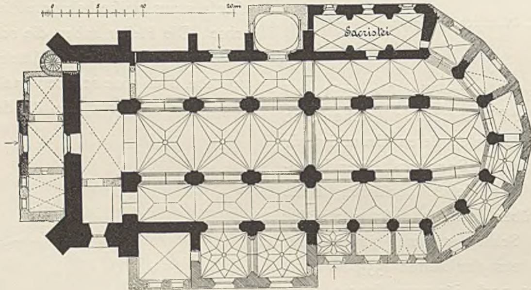
28. Grundriss der k. Pfarrkirche in Guhrau.
