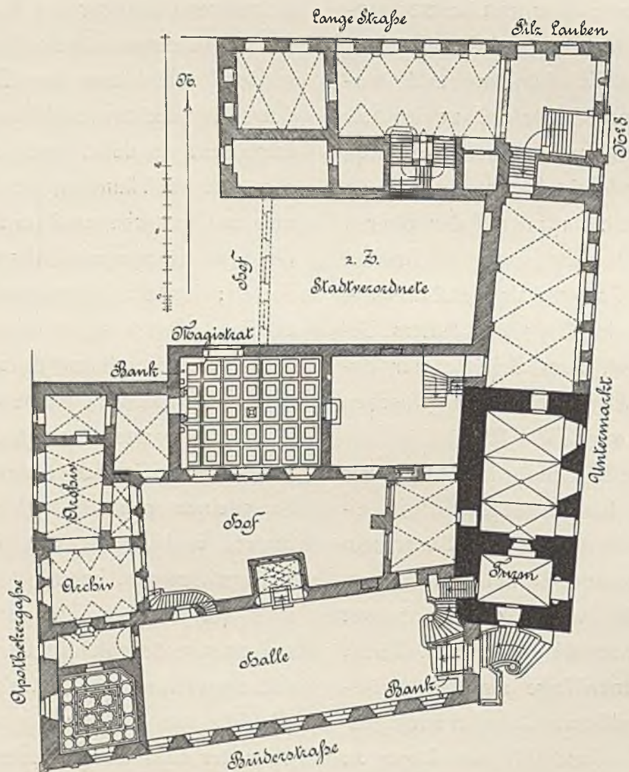
46. Grundriss des Hauptgeschosses des Rathauses in Görlitz.
