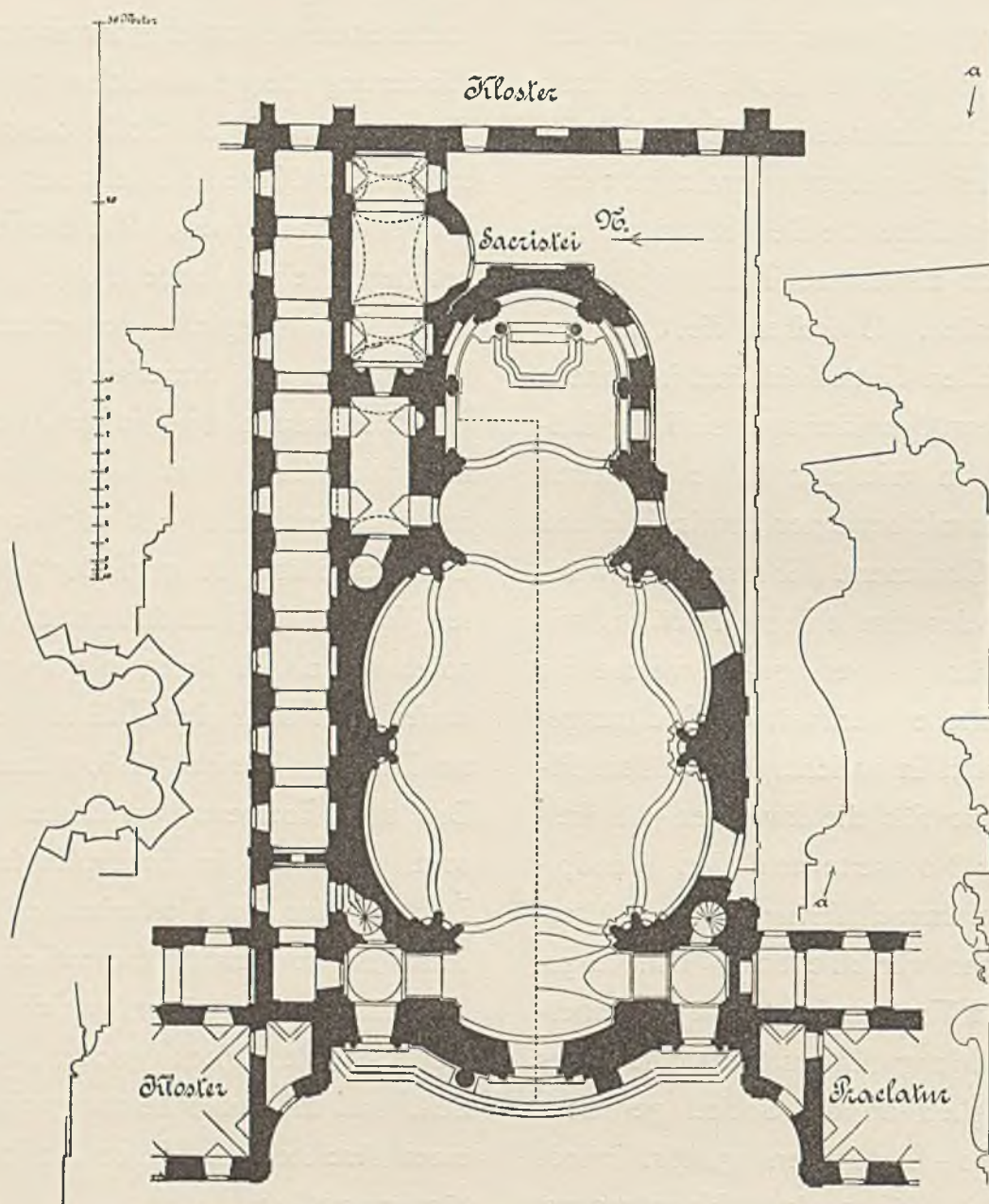
66. Grundriss und Profile der Klosterkirche in Wahlstatt.
