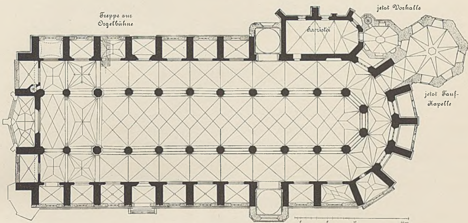
23. Grundriss der k. Pfarrkirche in Neisse.
