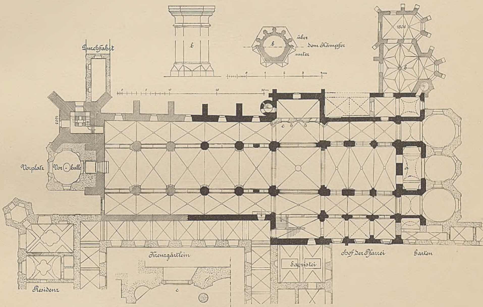
6. Grundriss der Klosterkirche in Heinrichau.
