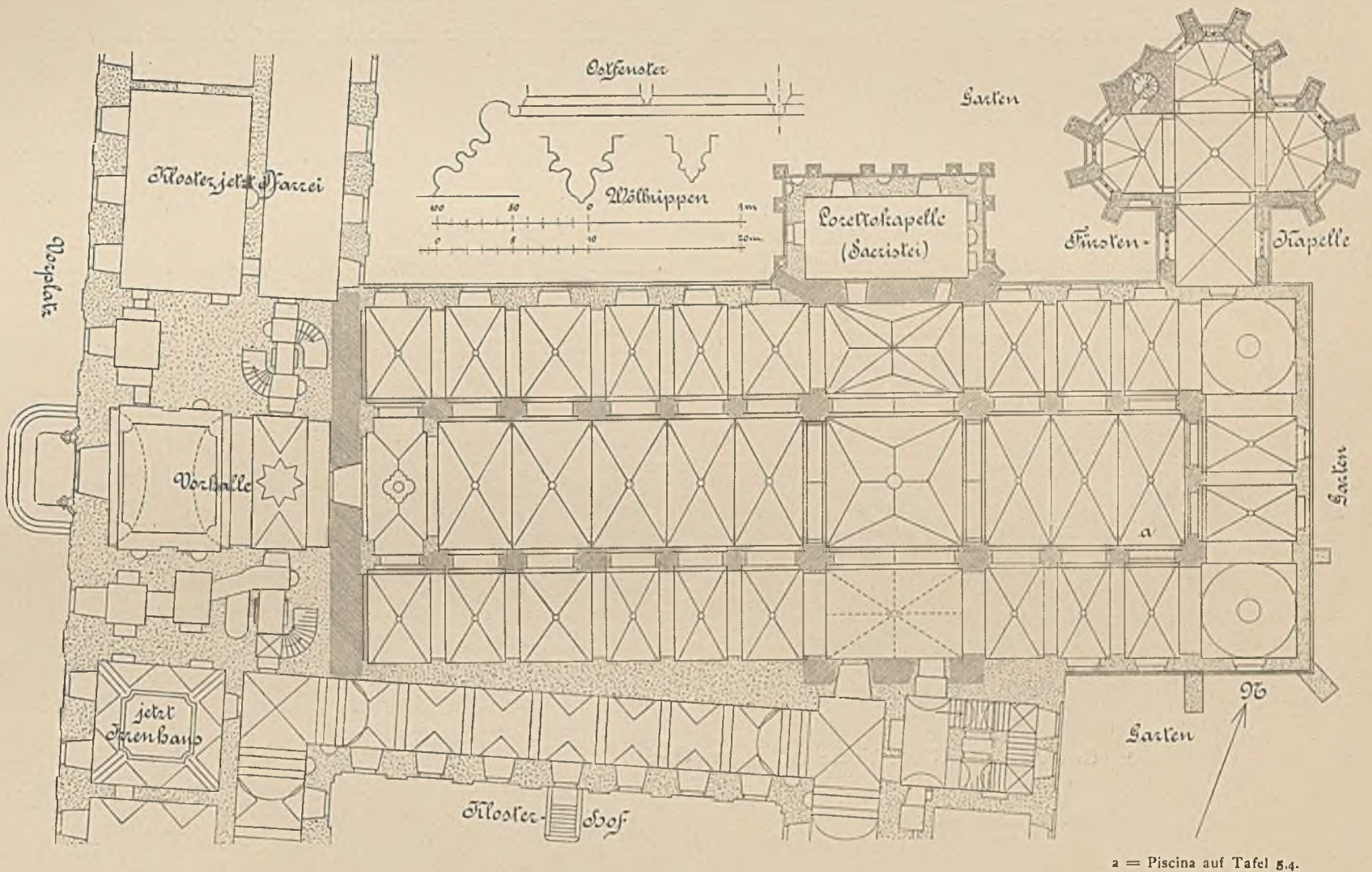
8. Grundriss der Klosterkirche in Leubus.
