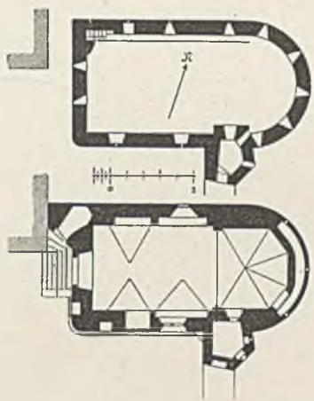
54. 55. Antoniuskapelle in Striegau. Oberer und unterer Grundriss.
