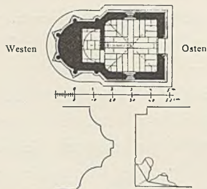
29. Heiliges Grab neben der Bergelkirche in Sagan. Grundriss nebst Fenster- und Portalprofilen.
