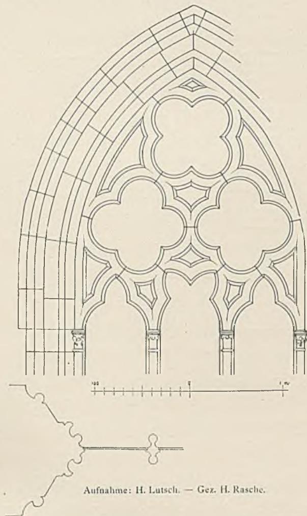
17. Fenstermaßwerk aus dem Langhause der Pfarrkirche in Goldberg.
