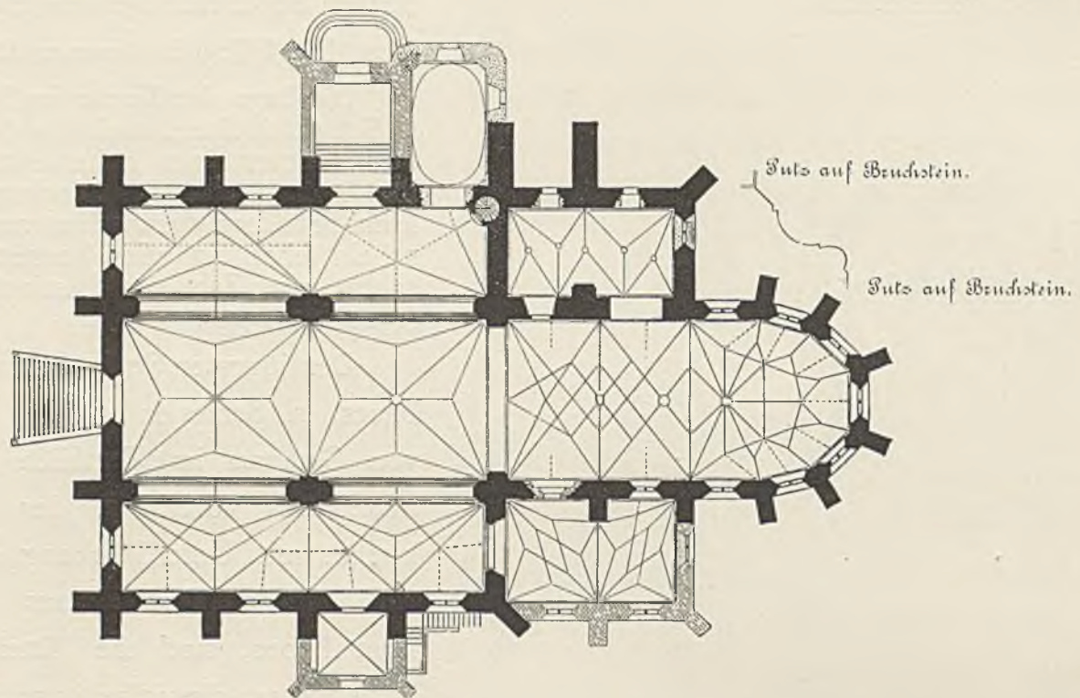
27. Grundriss und Sockelprofil der k. Pfarrkirche in Patschkau.
