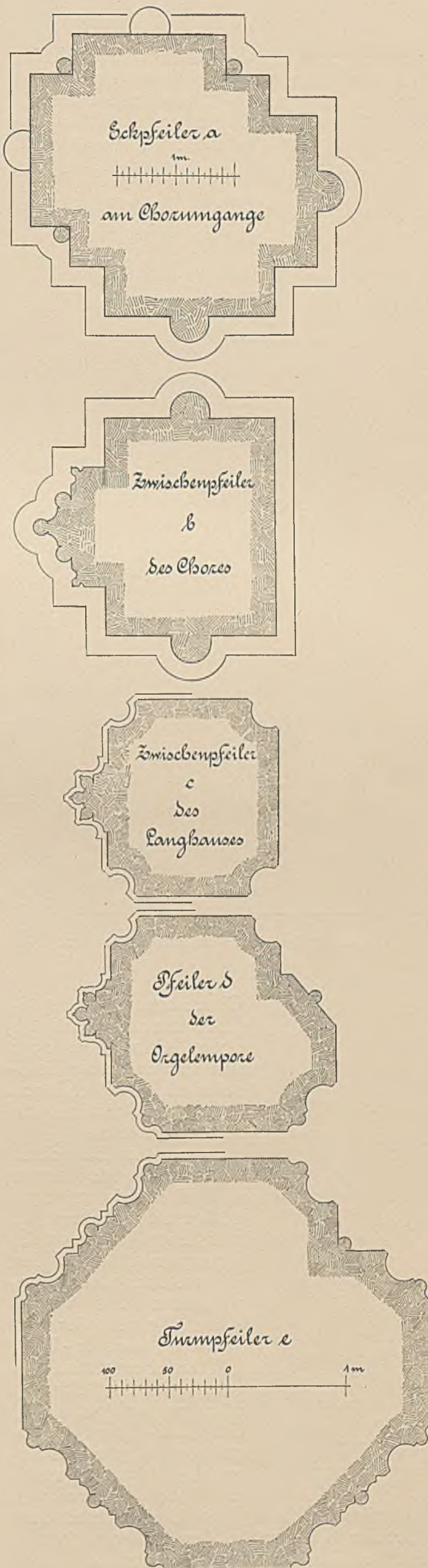
10 bis 14. Einzelheiten der Pfeiler des Doms in Breslau. Zu Tafel 11, 4.
