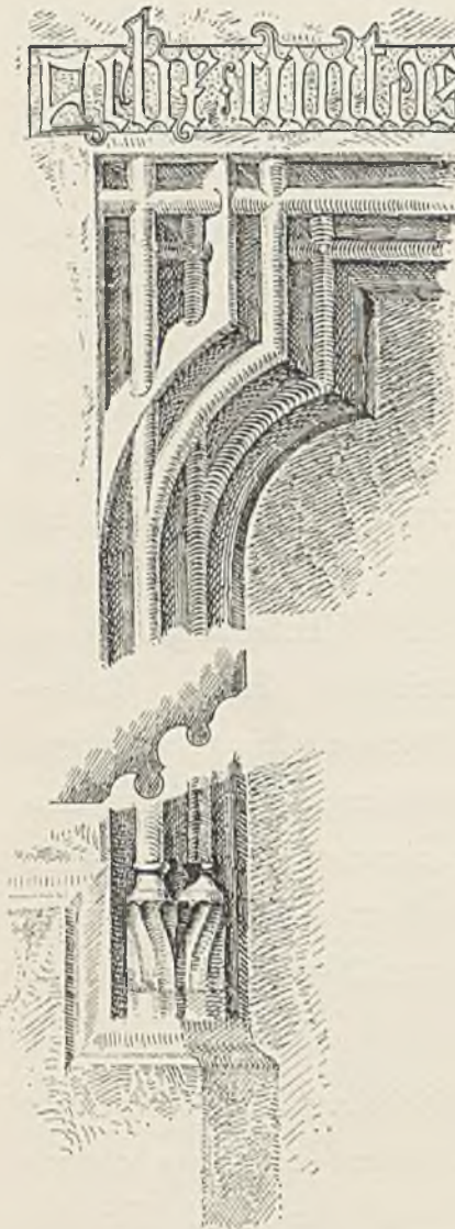
37. Portalgewände aus dem Rathause in Schweidnitz.
