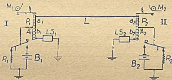
Rys. 33. SCHEMAT UKŁADU PRZECIWSOBNEGO (DUPLIX) DO PRZESYŁANIA PO JEDNYM PRZEWODZIE DWÓCH DEPEZ W PRZECIWNYM KIERUNKACH
