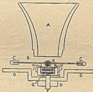
Rys. 43. MIKROFON TELEFONICZNY WSPÓŁCZESNY A — tuba, B — membrana, E — czasza miedziana, H — krążek miki, M — krążek węglowy
