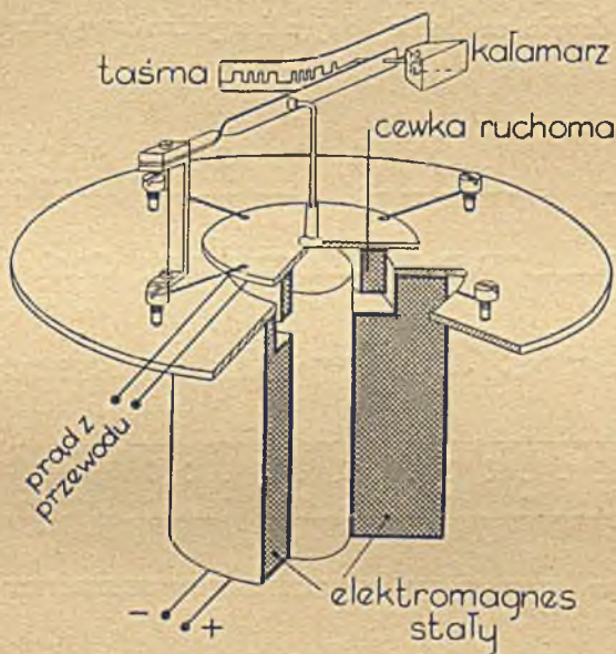
Rys. 31. ZAPISYWACZ SYFONOWY KELVINA (siphon recorder)
