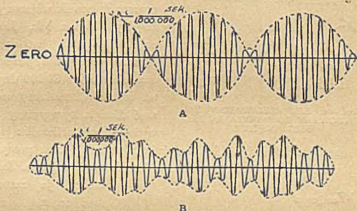
Rys. 68. ZMIANY NATĘŻENIA PRĄDU NOSNEGO POD WPEŁYWEM MIKROFONU A odpowiada pojedynczej gwizdanej nucie, B — mowie. Częstotliwość prądu nośnego: 1 000 000 drgań na sekundę.
