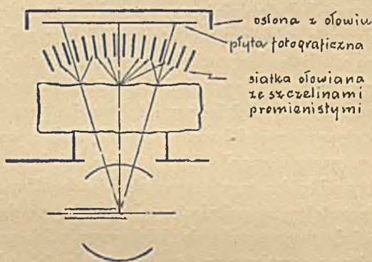
Rys. 83. PRZESŁONA POTTERA-BUCKYEGO
