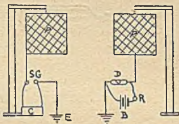
rys. 61. JEDEN Z PIERWSZYCH UKŁADÓW NADAWCZO-ODBIORCZYCH MARCONIEGO
