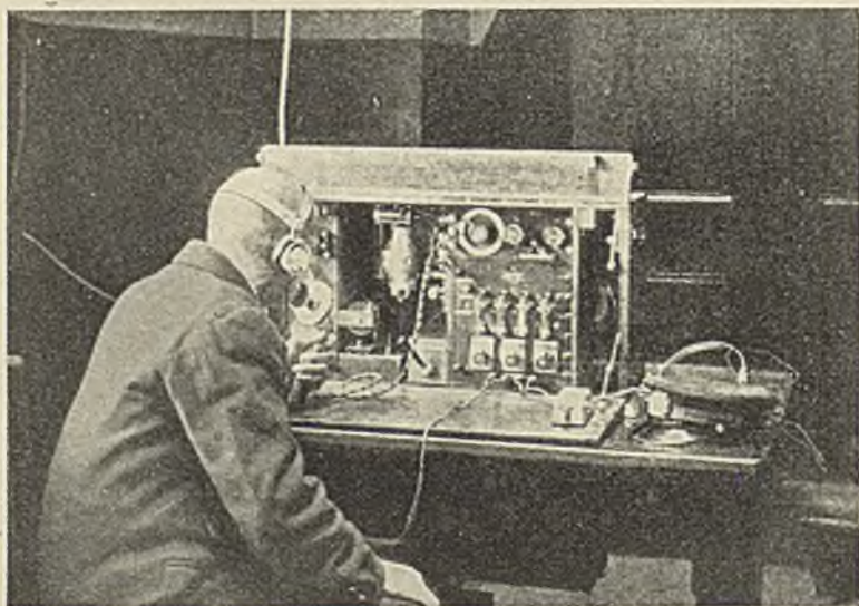
B. JEDNO Z PIERWSZYCH ROBOCZYCH URZĄDZEŃ RADIO-TELEFONICZNYCH Stosowane do komunikacji z okrętem-laternią
