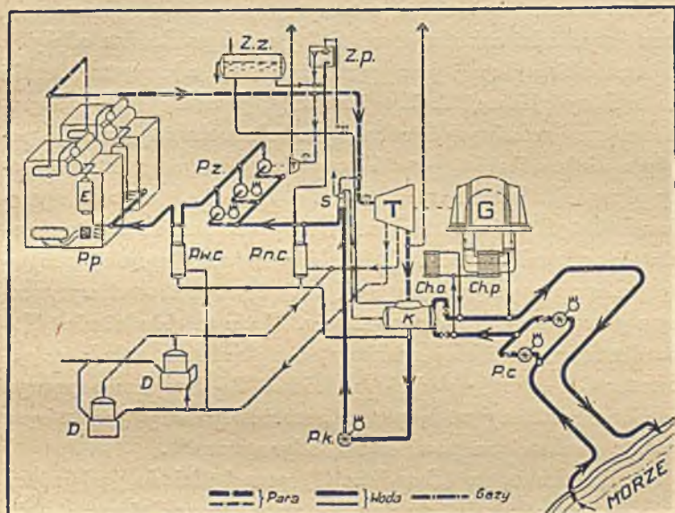
Rys. 21. SCHEMAT OBIEGU CIEPLNEGO ELEKTROWNI PAROWEJ „GRÓDKA” W PORCIE GDYŃSKIM
