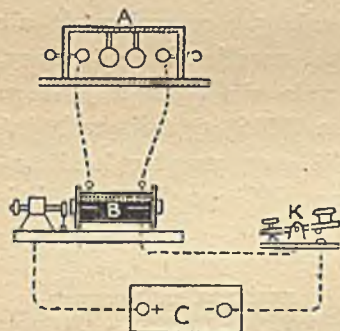
Rys. 60. JEDEN Z PIERWSZYCH SCHEMATÓW NADAWCZYCH MARCONIEGO
