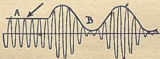
Rys. 40. PRĄD NOŚNY SINUSOIDALNY (A) I MODULOWANY (B)
