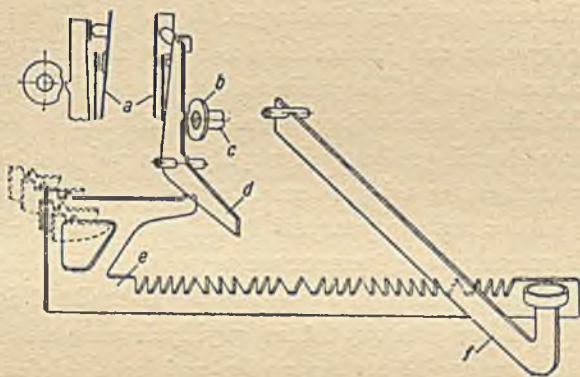
Rys. 39. SZYNA WYBIERAKOWA DALEKOPISU „MECHANICZNEGO „SIEMENS-HALSKE“
