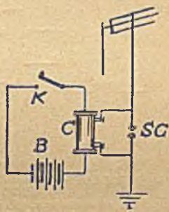
Rys. 63. PIERWSZY UKŁAD MARCONIEGO Z ANTENĄ SG — iskiernik, C — cewka indukcyjna, K — klucz Morse'a, B — bateria miejscowa
