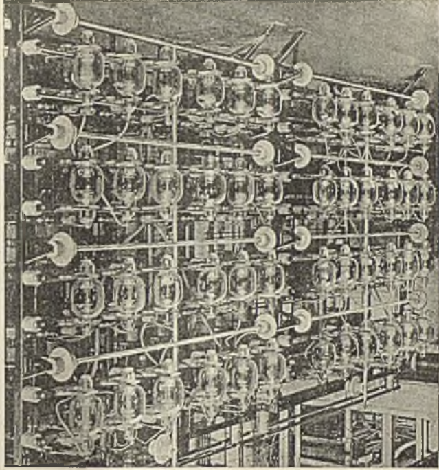
A. NAJWIĘKSZY UKŁAD LAMP NA ŚWIECIE 48 lamp nadawczych na stacji Marconi'ego w Caernarvon
