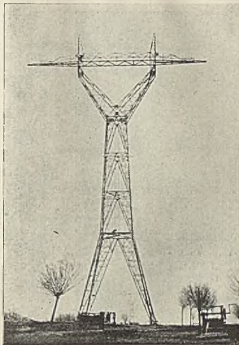
B. SŁUP SPECJALNY LINII PRZESYŁOWEJ MOŚCI-CE-STARACHOWICE O NAPIĘCIU 150 000 WOLTÓW
