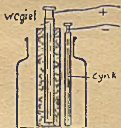
Rys. 9. OGNIWO LECLANCHÉGO
