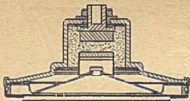
Rys. 44. NAJNOWSZA POSTAĆ MIKROFONU TELEFONICZNEGO Obie elektrody całkowicie zanurzone w proszku
