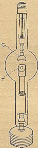
Rys. 78. WSPÓL- CZESNA RURA RENTGENOWSKA (COOLIDGE'A) T — tarcza, C — ka- toda rozżarzona
