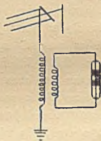
Rys. 65. SCHEMAT ODBIORCZY STRO- JONY DO NADAJ- NIKA NA RYS. 64.
