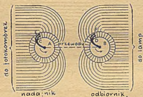
Rys. 98. PRZEŁĄCZNIK, KTÓRY MOŻNABY ZASTOSOWAĆ PRZY TELEWIZJI SYSTEMEM RUHMERA
