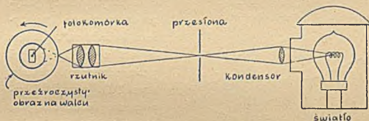
Rys. 91. SCHEMAT NADAJNIKA FOTOTELEGRAFICZNEGO SYSTEMU IVESA
