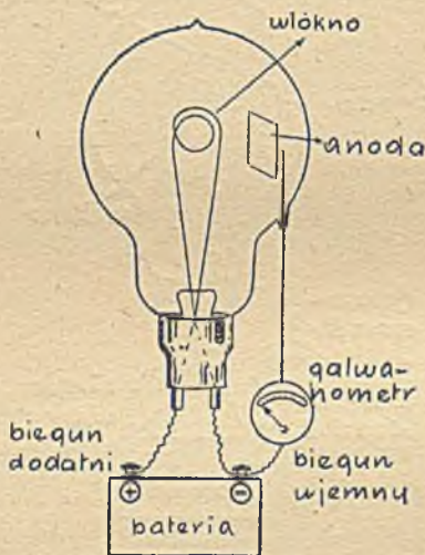
Rys. 72. GDY W UKŁADZIE EDISONA ANODA JEST POŁĄCZONA Z UJEMNYM BIEGUNEM BATERII, NIE MA PRĄDU. (Por. rys. 71).
