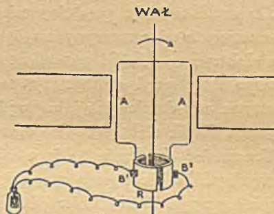
Rys. 19. ZASADA PRĄDNICY PRĄDU STAŁEGO
