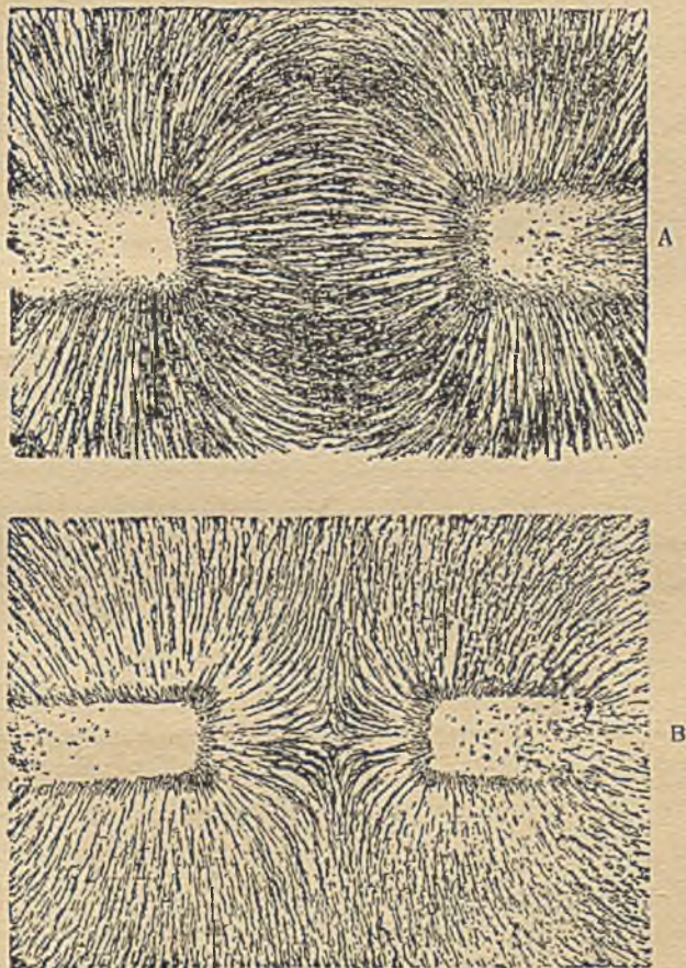
Rys. 2. LINIE SIŁ POLA MAGNETYCZNEGO Opilki żelazne rozsypane na arkuszu papieru, pod którym znajdują się dwa magnesy liniowe. A — bieguny różnoimienne, B — bieguny jednoimienne
