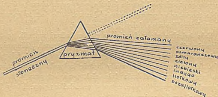
Rys. 80. WIDMO ŚWIATŁA BIAŁEGO
