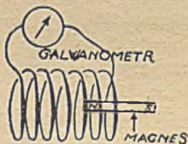
Rys. 16. MAGNES PORUSZAJĄCY SIĘ WEWNĄTRZ CEWKI WYWÓLUJE W NIEJ PRĄD ELEKTRYCZNY
