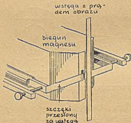
Rys. 92. WENTYL ŚWIETLNY SYSTEMU IVESA
