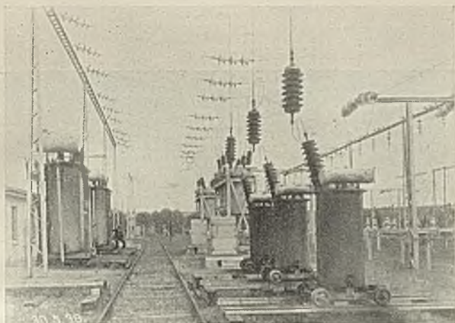
A. TROZDZIELNIA 60 000 V W ŻURZE POD GOŁYM NIEBEM
