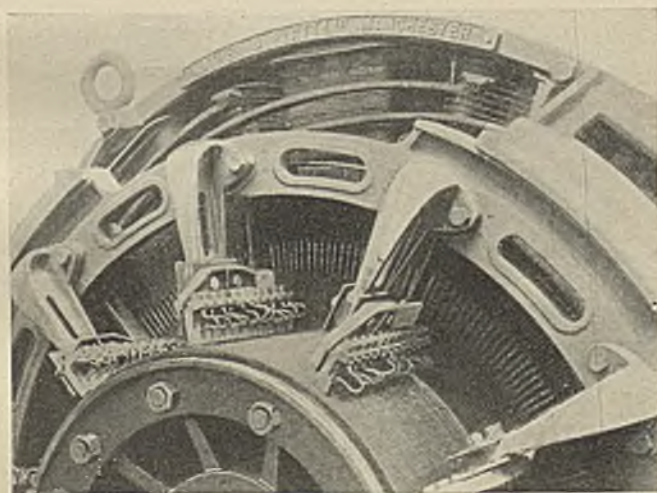
B. CZĘŚĆ TEJŻE PRĄDNICY. WIDĄC SZCZOTKI WĘGLOWE PRZYCIŚNIĘTE DO MIEDZIANYCH WYCINKÓW KOMUTATORA U góry widać magnesy pola i ich uzwojenie.
