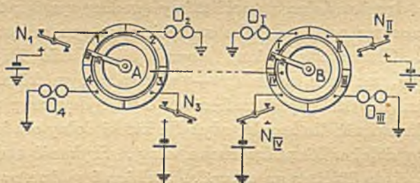
Rys. 37. SCHEMAT TELEGRAFU POSPIESZNEGO WIELOKROTNEGO (CZTERY DEPEZYE PO JEDNYM PRZEWODZIE) N — aparaty nadające, O — aparaty odbierające
