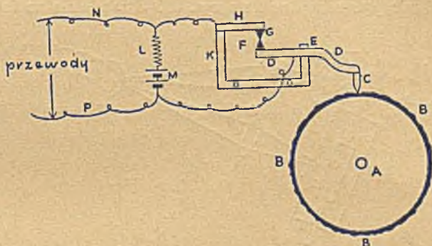
Rys. 88. SCHEMAT NADAJNIKA TELEAUTOGRAFIKZNEGO SYSTEMU BELINA
