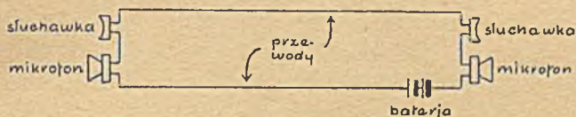
Rys. 45. NAJPROSTSZY OBWÓD TELEFONICZNY
