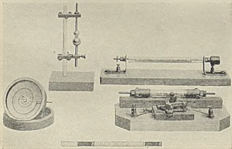
B. (Na lewo) KOHERER SPRĘŻYNOWY LODGE'A (1894), KOHERER Z PRZERWĄ SPRĘŻYNOWĄ (1889), (Na prawo) DWA KOHERERY BRANLY-LODGE'A, DOLNY ZE WSTRZĄSACZEM. U dołu skala w calach.
