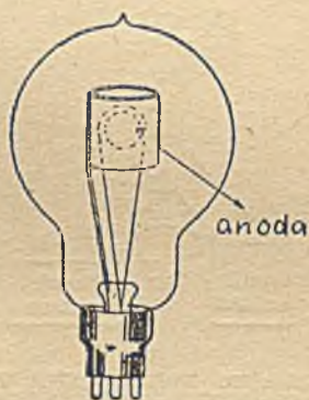
Rys. 73. ANODA CYLINDRYCZNA DOKOŁA WŁÓKNA WPROWADZONA PRZEZ FLEMINGA
