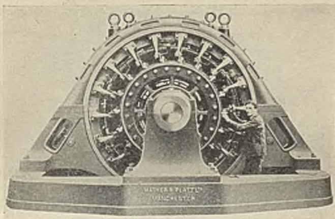
A. WIELKA PRĄDNICĄ PRĄDU STAŁEGO DO PRODUKCJI CHEMIKALÓW ZA POMOCĄ PRĄDU ELEKTRYCZNEGO
