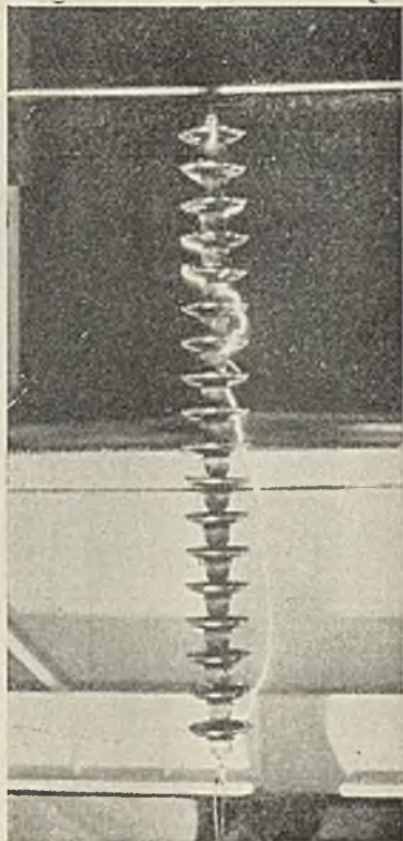
A. DZIAŁANIE BŁYSKAWICY NA NIEZABEZPIECZONY IZOLATOR
