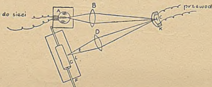
Rys. 89. SCHEMAT ODBIORNIKA TELEAUTOGRAFICZNEGO SYSTEMU BELINA
