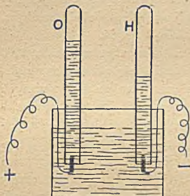
Rys. 11. ELEKTROLIZA WODY
