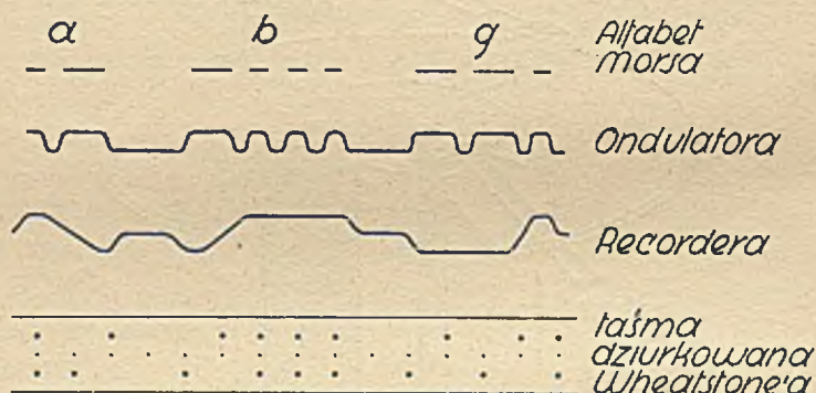
Rys. 32. ZESTAWIENIE KILKU ALFABETÓW TELEGRAFICZNYCH
