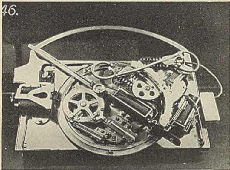
A. WYBIERAK PŁASKI ERICSSONA Ramie jego ma dwa ruchy: promieniowy i obrotowy
