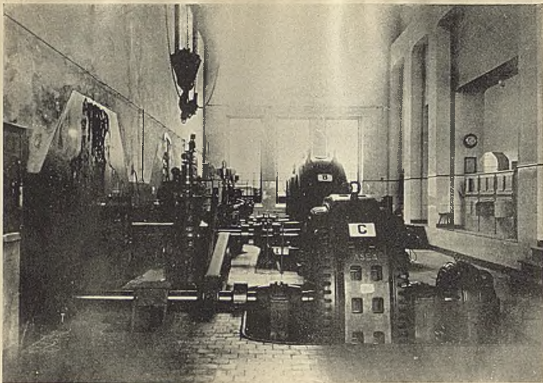
WNĘTRZE MASZYNOWNI ZAKŁADU WODNO-ELEKTRYCZNEGO W GRÓDKU Turbozespoły poziome
