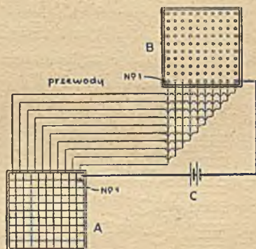
Rys. 97. UKŁAD RUHMER DO TELEWIZJI
