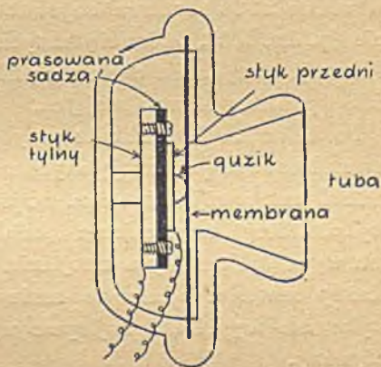
Rys. 12. MIKROFON Z MASĄ WĘGLOWĄ EDISONA
