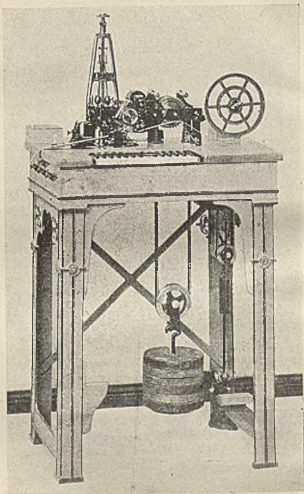
APARAT TELEGRAFICZNY DRUKUJĄCY, NADAWCZO-ODBIORCZY HUGHESA (JUŻ)
