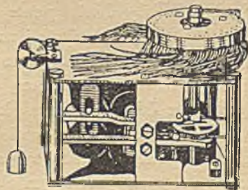
Rys. 51. WCZESNA POSTAĆ TELEFONU AUTOMATYCZNEGO
