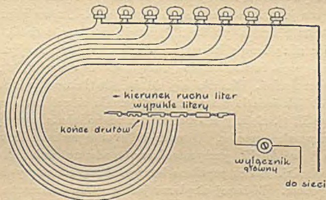
Rys. 29. SCHEMAT POŁĄCZEŃ DLA OSMIU LAMP JEDNEGO RZĘDU W „KURIERZE ŚWIETLNYM“
