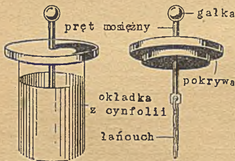
Rys. 5. BUTELKA LEJDEJSKA
