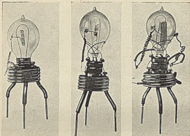
A. PIERWSZE LAMPY FLEMINGA (1904) STOSOWANE PRZEZEŃ JAKO DETEKTORY RADIOWE
