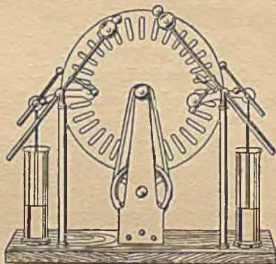
Rys. 4. MASZYNA WIMSIIURSTA do wytwarzania elektryczności przez tarcie
