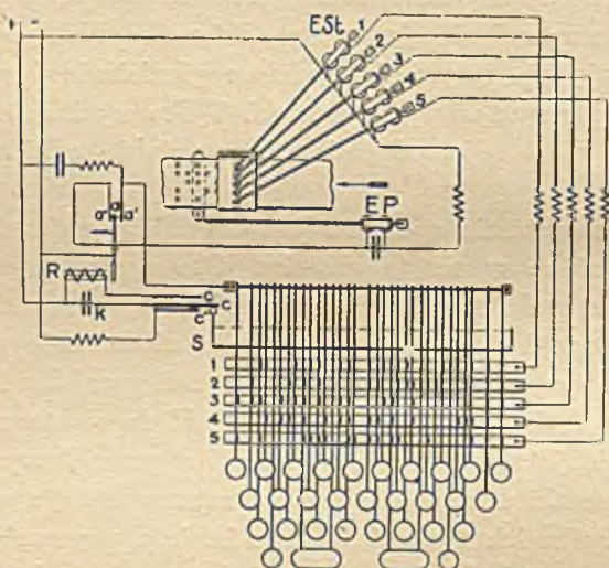
Rys. 39. SCHEMAT DZIURKARKI TELEGRAFU POŚPIESZNEGO SYSTEMU SIEMENSA
