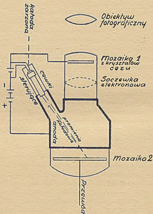
Rys. 100. IKONOSKOP ZWORYKINA w ostatnim wykonaniu
