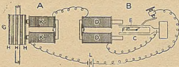
Rys. 87. BĘBEN FONICZNY I PRZERYWACZ WIDEŁKOWY DO SYNCHRONIZACJI W SYSTEMIE RANGERA (WG MIHALYEGO).
