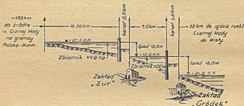
Rys. 23. SCHEMATYCZNY PROFIL ZBIORNIKÓW WODNYCH I SPADÓW ZAKŁADÓW WODNO-ELEKTRYCZNYCH W ŻURZE I GRÓDKU
