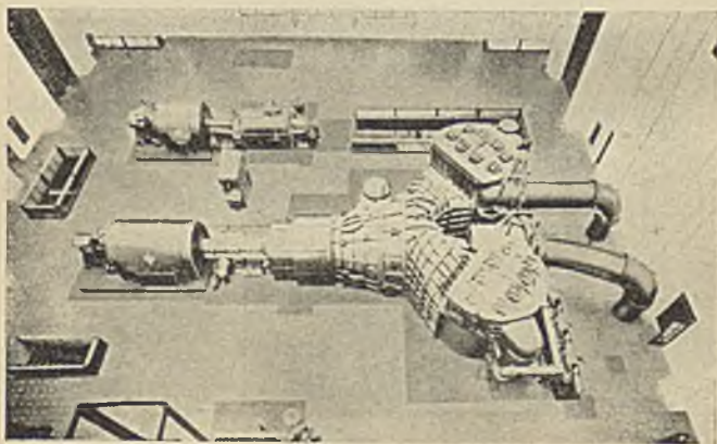
B. TURBOZESPÓŁ PARSONSA O MOCY 50 000 kW ustawiony w Chicago
