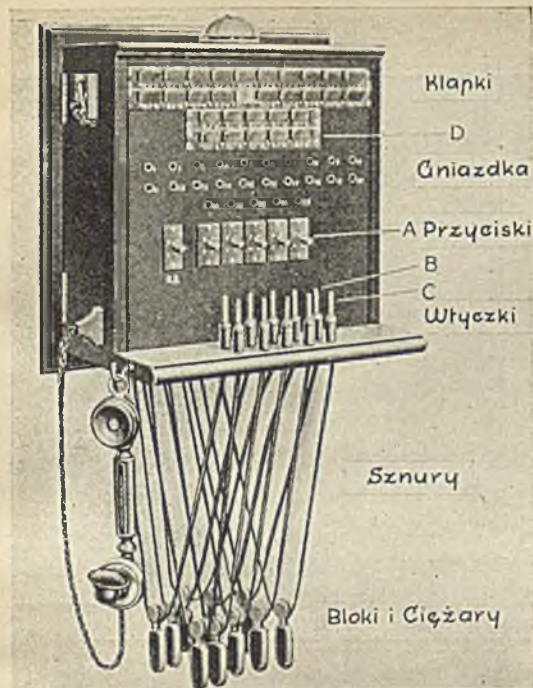
MAŁA ŁĄCZNICA TELEFONICZNA RĘCZ- NA NA 25 ABO- MENTÓW
