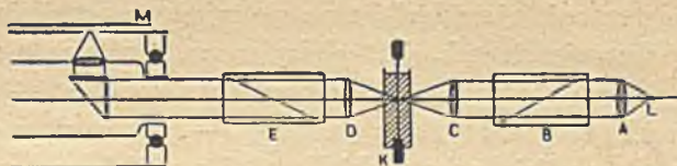
Rys. 96. UKŁAD OPTYCZNY ODBIORNIKA FOTOTELEGRAFICZNEGO MARCONI-WRIGHTA
