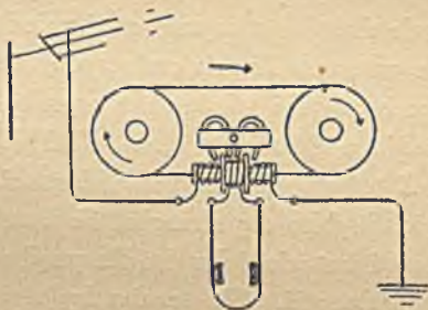
Rys. 66. DETEKTOR MAGNETYCZNY MARCONIEGO
