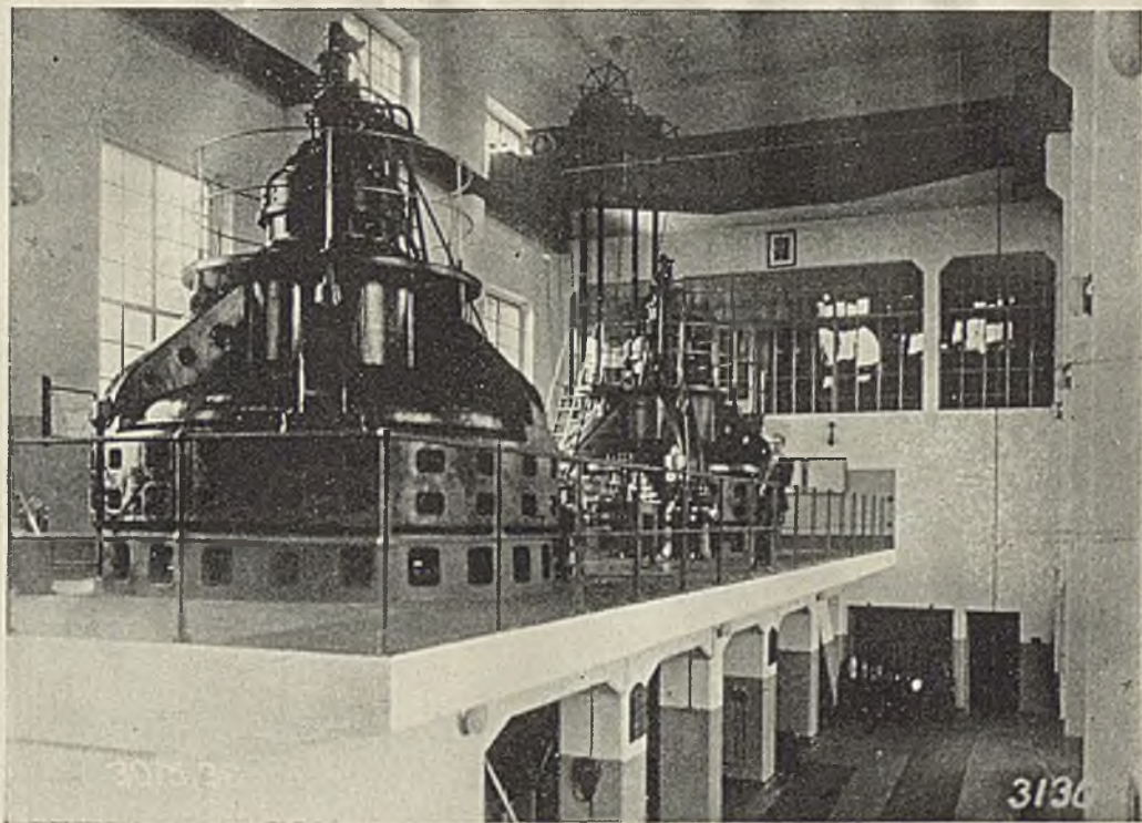
WNĘTRZE MASZYNOWNI ZAKŁADU WODNO-ELEKTRYCZNEGO W ŻURZE Turbozespoły pionowe. Widoczne turbiny.
