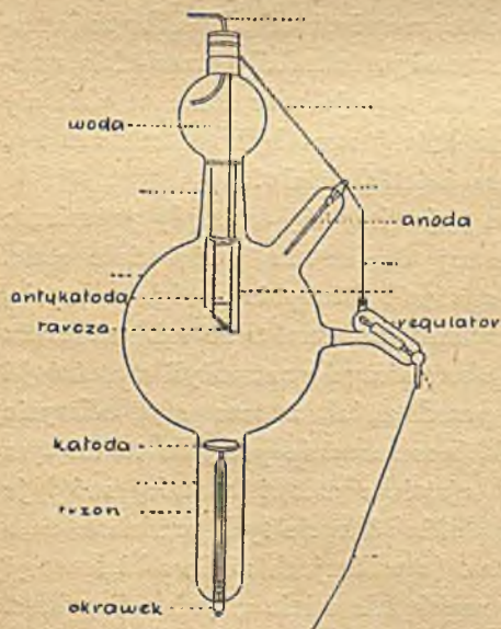
Rys. 77. POSTAĆ RURY RENTGENOWSKIEJ, UŻYWANEJ DO NIEDAWNA
