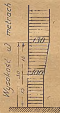
Parcie wiatru w kg/m 2
