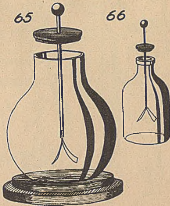
Elektroskop
