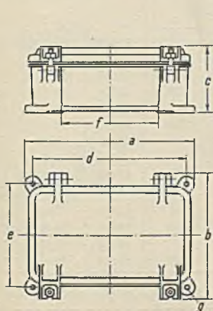
Maßbild für Listen-Nr. 93001 bis 93004.
