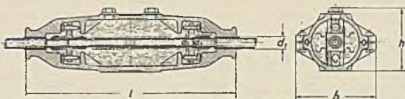
Abmessungen siehe Maßtabelle.
