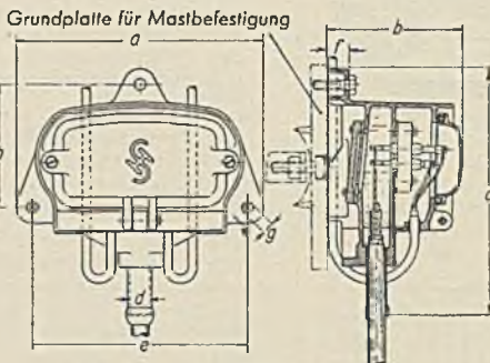
Abmessungen siehe Maßtabelle.
