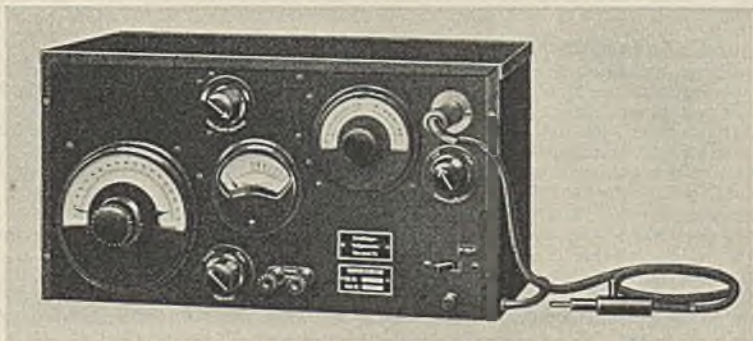
Empfänger-Prüfgenerator.
