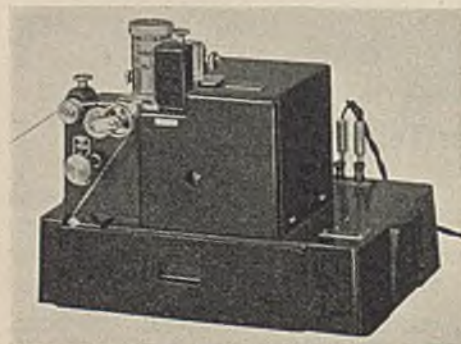
Drehspulnschnellschreiber.
