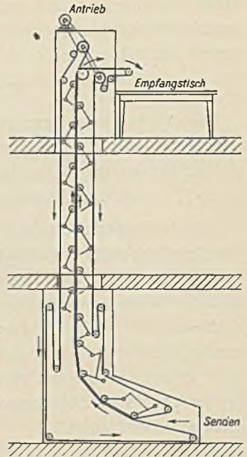
Schema eines Bandaufzuges.
