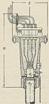
Abmessungen siehe Maßtabelle.
