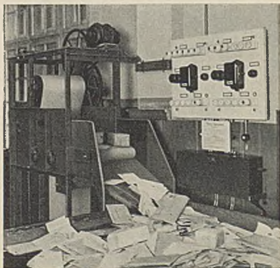
Endstelle einer Briefkastenleerungs-Anlage mit Bandaufzug.
