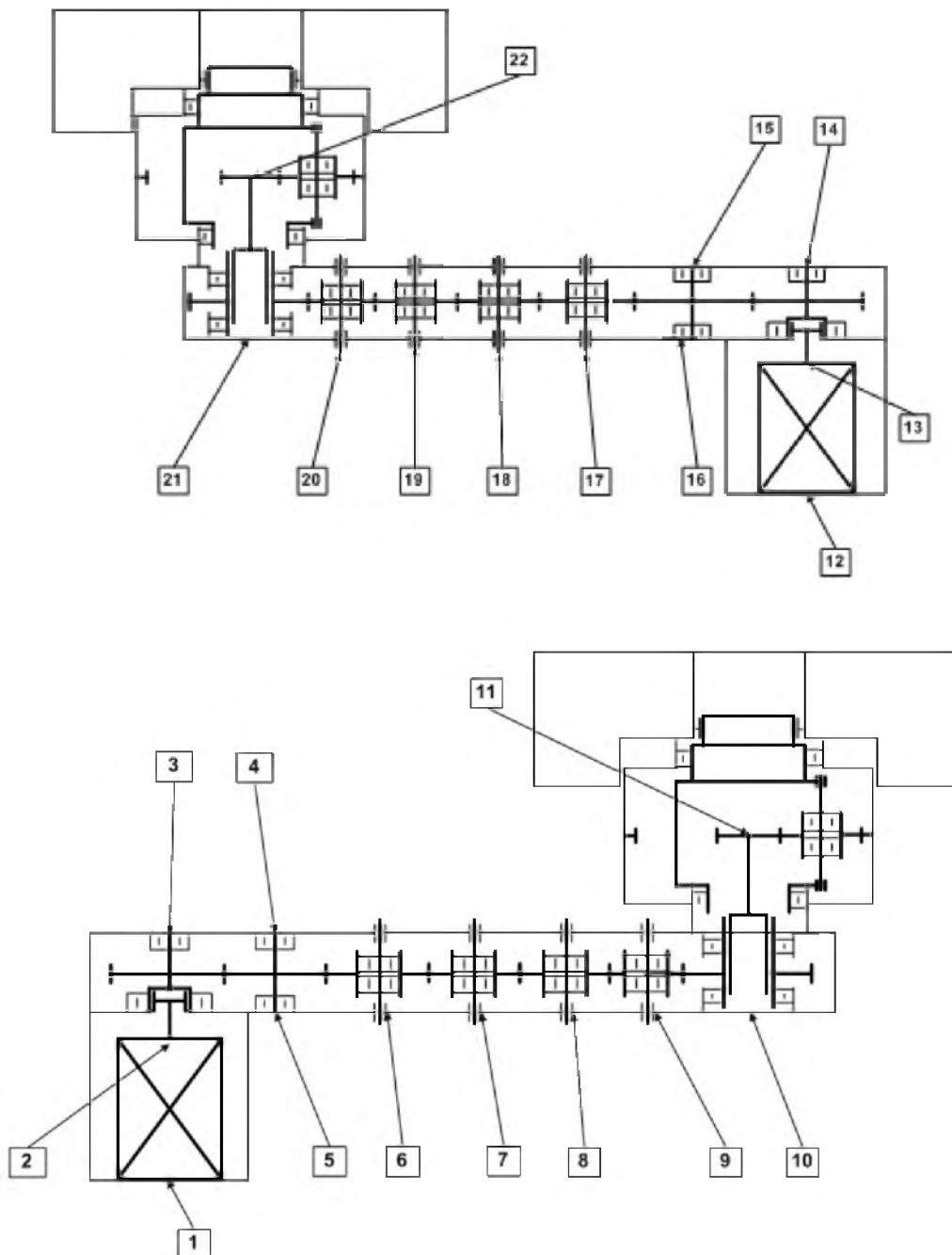
Rys. 4.8 Schematy kinematyczne ramion kombajnu ściany Eickhoff SI-300, z zaznaczonymi punktami pomiarowymi
