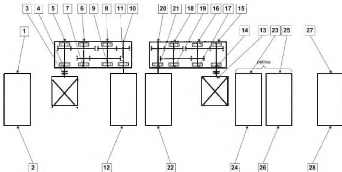
Rys. 4.9 Schemat kinematyczny z zaznaczonymi punktami pomiarowymi przenośnika taśmowego Gwarek
