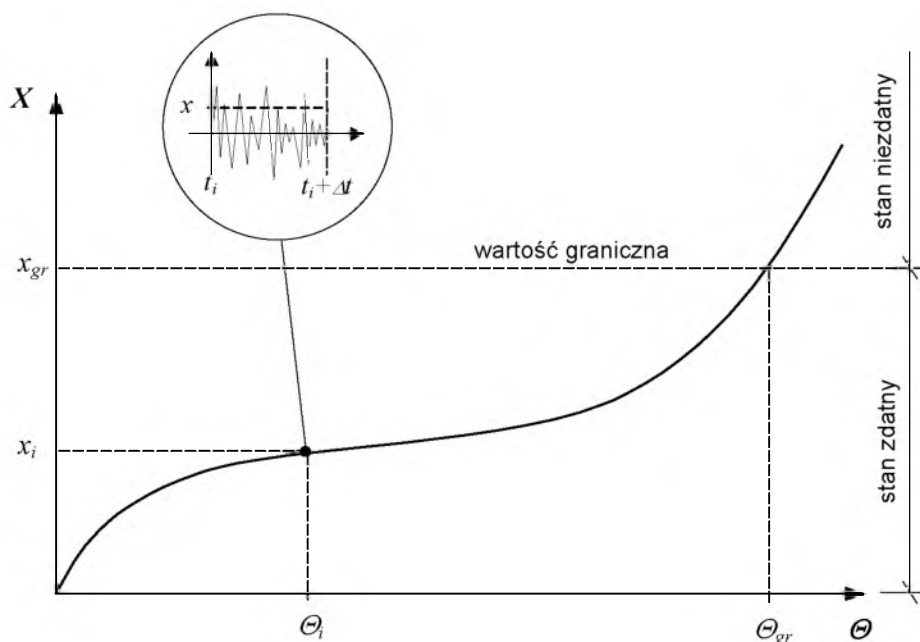
Rys. 4.1 Idea obserwacji przebiegu wartości symptomu stanu w czasie:
