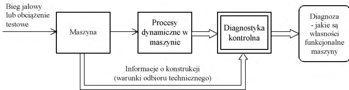
Rys. 4.5 Schemat współzależności w przypadku wibroakustycznej diagnostyki kontrolnej maszyn
