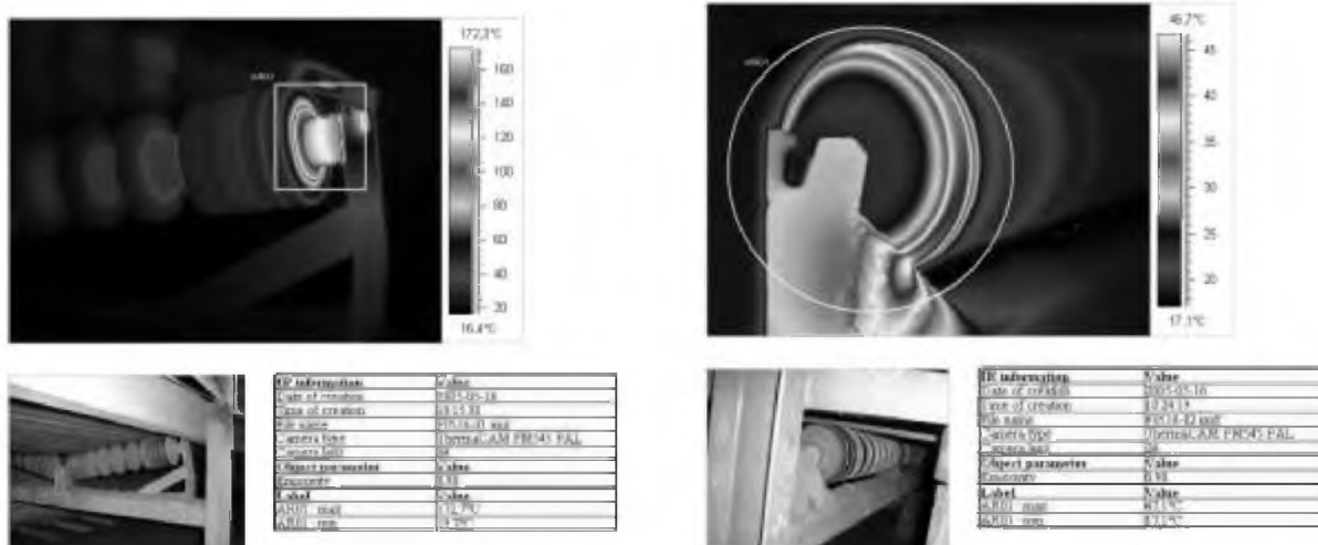
Rys.4.4 Termogramy krążnika zabudowanego na powrocie taśmy
