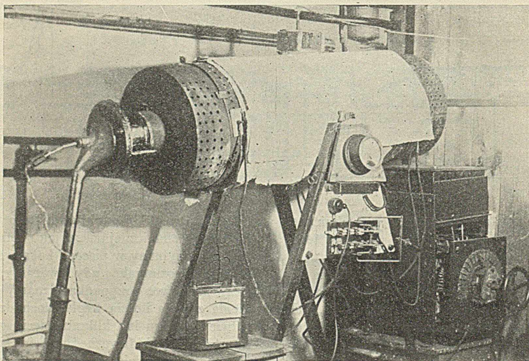
Rycina 2. Fotografia pieca Wölblinga po przeróbce.
