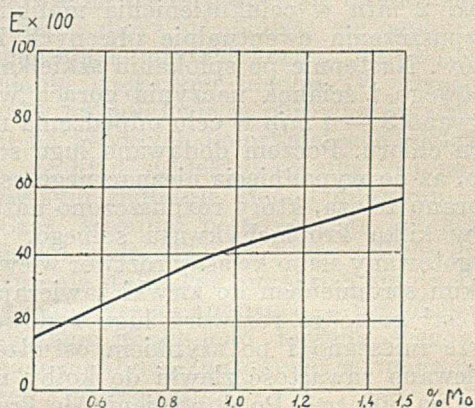
Rycina 6. Krzywa zawartości molibdenu od 0,5 do 1,5%. Filtr S 50. Długość warstwy 50 mm. 1 g naważki -500\text{ cm}^3 \rightarrow 10\text{ cm}^3 = 0,02\text{ g} .
