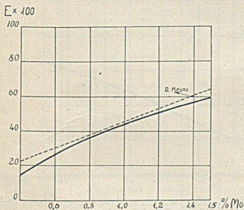
Rycina 4. Krzywa zawartości molibdenu od 0,5 do 1,5%. Filtr S 436 Hg. Długość warstwy 50 mm. 1 g naważki -500\text{ cm}^3 \rightarrow 10\text{ cm}^3 = 0,02\text{ g} .
