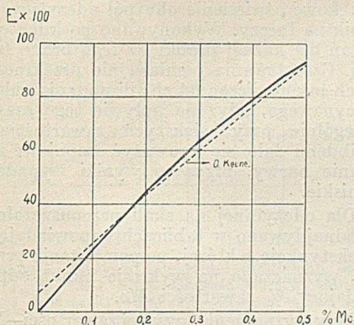
Rycina 3. Krzywa zawartości molibdenu od 0 do 0,5%. Filtr S 436 Hg. Długość warstwy 50 mm 1 g naważki -500\text{ cm}^3 \rightarrow 50\text{ cm}^3 = 0,1\text{ g} .
