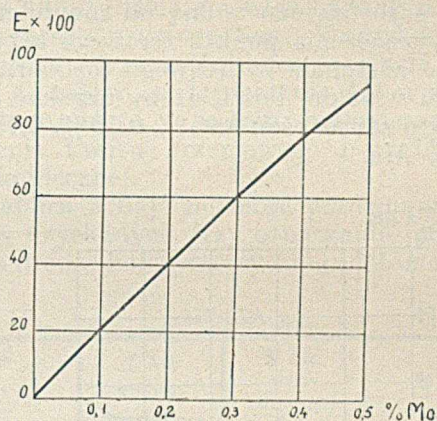
Rycina 5. Krzywa zawartości molibdenu od 0 do 0,5%. Filtr S 50. Długość warstwy 50 mm. 1 g naważki -500\text{ cm}^3 \rightarrow 50\text{ cm}^3 = 0,1\text{ g} .
