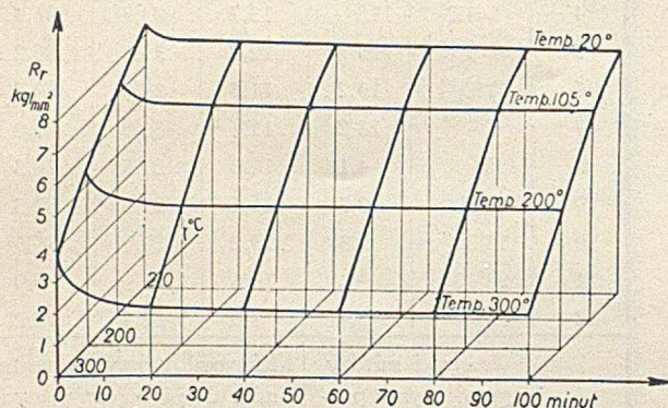
Rycina 1. Wykres przestrzenny wpływu szybkości rozciągania w wysokich temperaturach na wytrzymałość R_r aluminium. Oś pozioma przedstawia czas rozciągania próbki w minutach.
