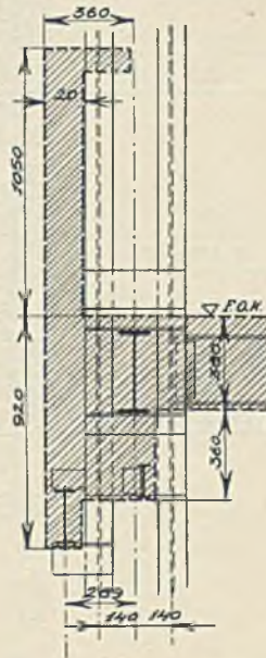
Abb. 81. Detail „A“.
