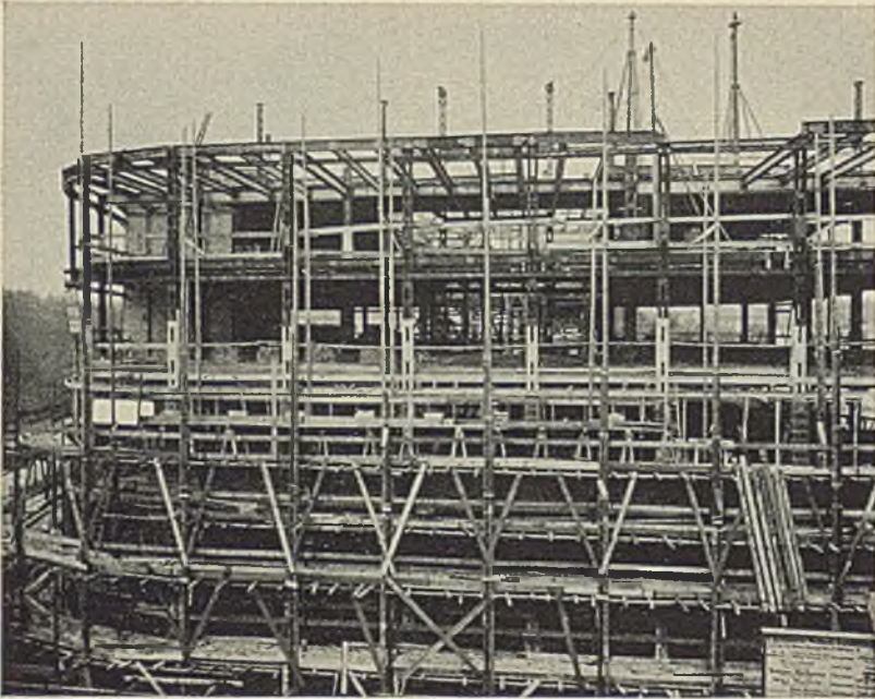
Abb. 3. Warenhaus Wertheim, Breslau. Aufstellung des Stahlgerüstes. Außenrüstung. Ausführung: Carlshütte A. G., Waldenburg-Altwasser i. Schl.
