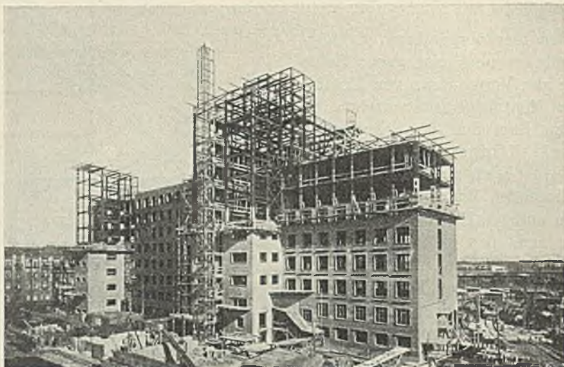
Abb. 332. Verwaltungsgebäude Wernerwerk X. Berlin-Siemensstadt. Montagebild. Teilweise Fertigstellung der Wände.
