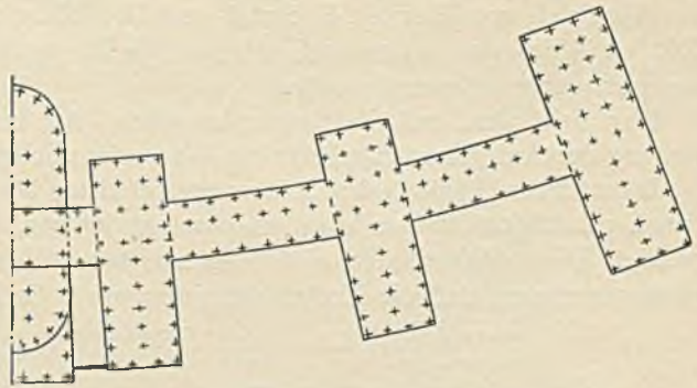
Abb. 27. Zentralverwaltungsgebäude der I. G. Farbenindustrie A. G., Frankfurt a. M. Grundriß. Nach Lackmann, H. u. H. Vierkorn: Die Brücke 1929.
