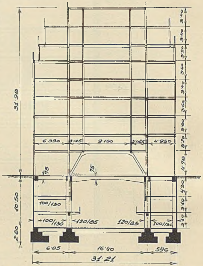
Abb. 36. Hochhaus „Berg- und Hüttenwerksges.“ in Prag. Querschnitt. Drei Kellergeschosse samt Theatersaal in Eisenbeton.
