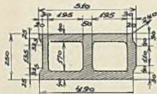
Abb. 235. Isostone-Wandstein (Prag).
