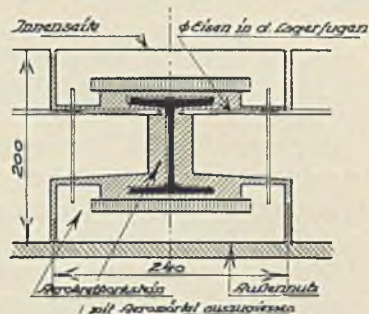
Abb. 270. Skelettbauweise „Torkret“. Stützedetail.
