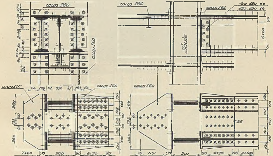
Abb. 52. Europahaus, Berlin. Trägeranschlüsse bei waagerechter Rahmenwirkung.
