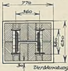
Abb. 262. Erdgeschoß.
