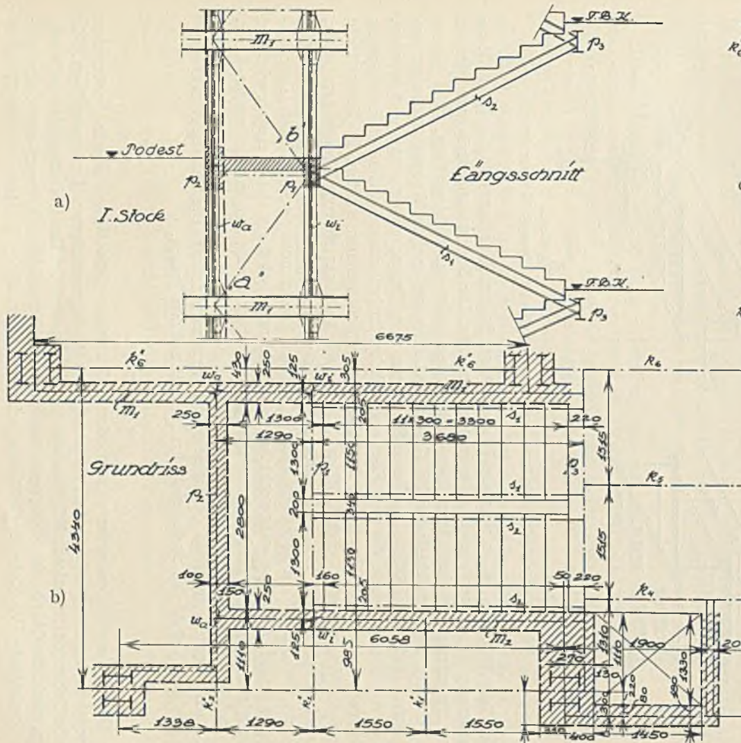
Abb. 199. Abb. 199 bis 201. Treppenkonstruktion (Nebentreppe), Hochhaus „Berg- und Hüttenwerkges.“ in Prag.
