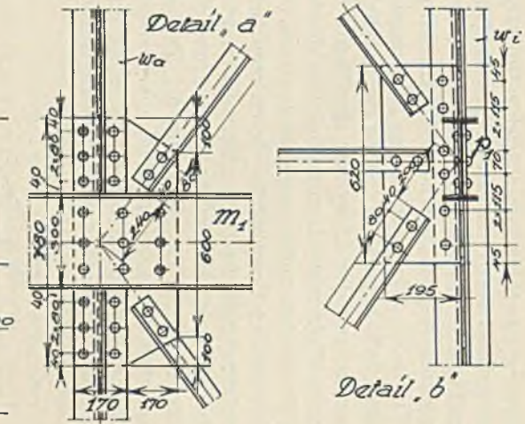
Abb. 199. Abb. 199 bis 201. Treppenkonstruktion (Nebentreppe), Hochhaus „Berg- und Hüttenwerkges.“ in Prag.
