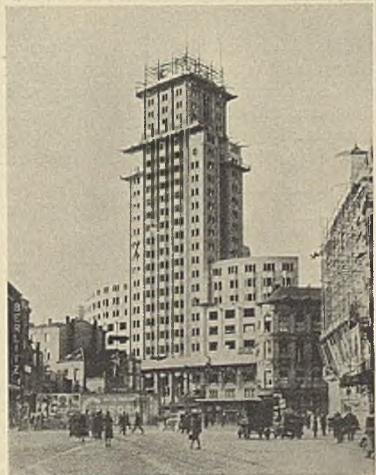
Abb. 453. Hochhaus der Allgem. Bankvereinigung in Antwerpen. Ansicht des nahezu fertigen Baues. Ausführung: DEMAG Aktienges. Duisburg.
