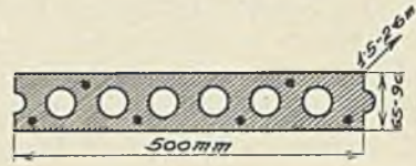
Abb. 216. Stegplatte.
