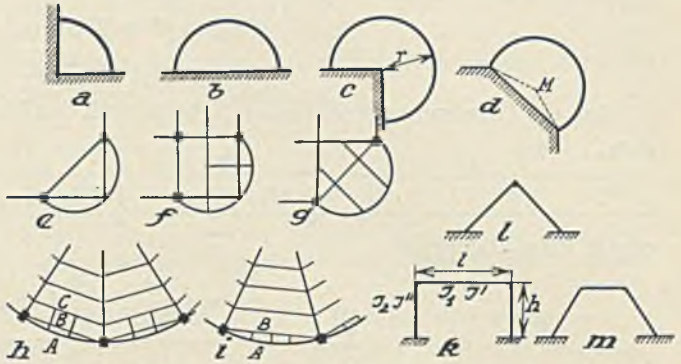
Abb. 212a bis m. Verschiedene Formen von Erkerträgern.
