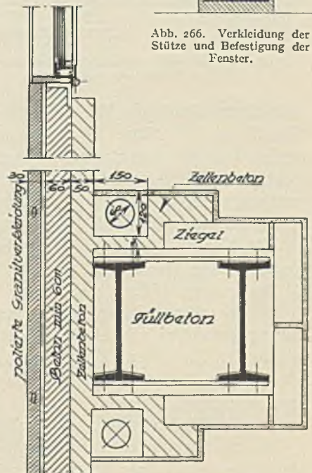
Abb. 267. Palais der Berg- u. Hüttenwerks-Gesellschaft in Prag.
