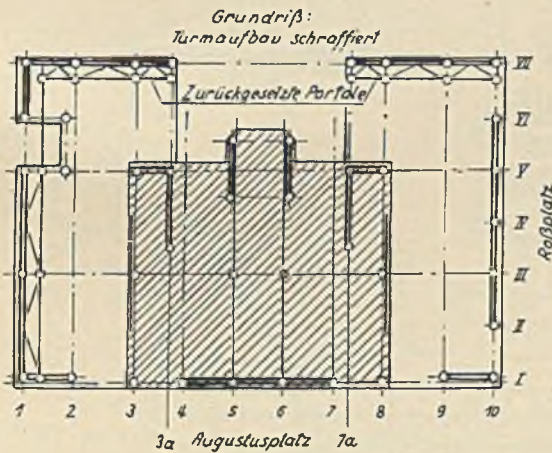
Abb. 427. Grundriß.
