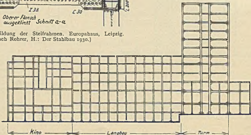
Abb. 431. Haus Grenzwacht, Aachen. Längsschnitt des Stahlskeletts. (Nach Teichmann, E.: Dt. Bauz. 1926.)
