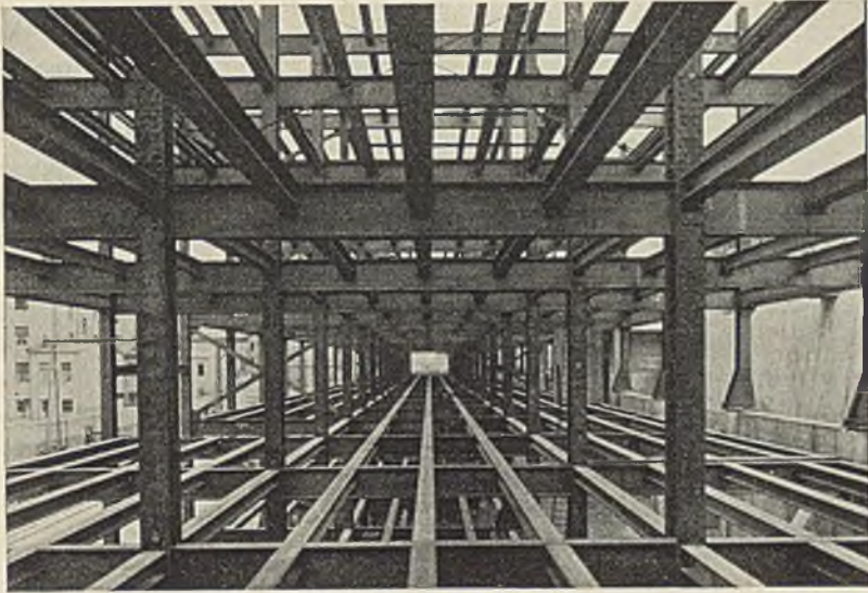
Abb. 54. Postlagergebäude in Stettin. Blick in eines der Geschosse. Ausführung: J. Gollnow & Sohn, Stettin.
