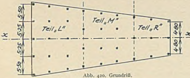
Abb. 420 bis 422. Windbeanspruchung eines Hochhauses.
