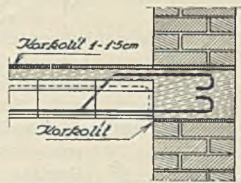
Abb. 223 b. Mauerauflager mit schalldämpfender Isolierung.
