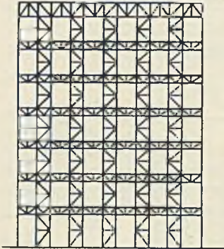
Abb. 188. Wandverbände.
