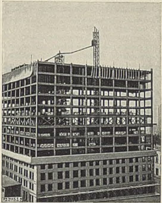
Abb. 338. Ausführung eines Stahlochhauses in Amerika. (Nach Griesel, H. Dr.: Z. V. d. I. 1929, S. 372.)
