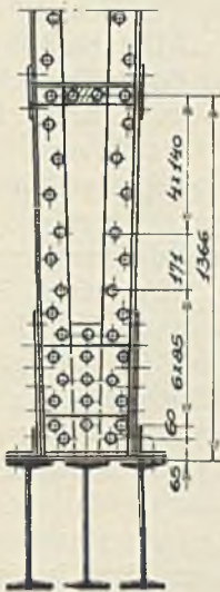
Abb. 136. Rahmenfuß.
