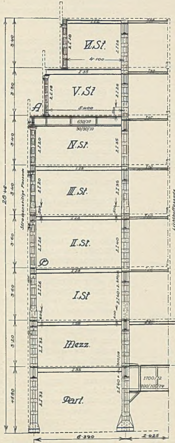
Abb. 80. Querschnitt.
