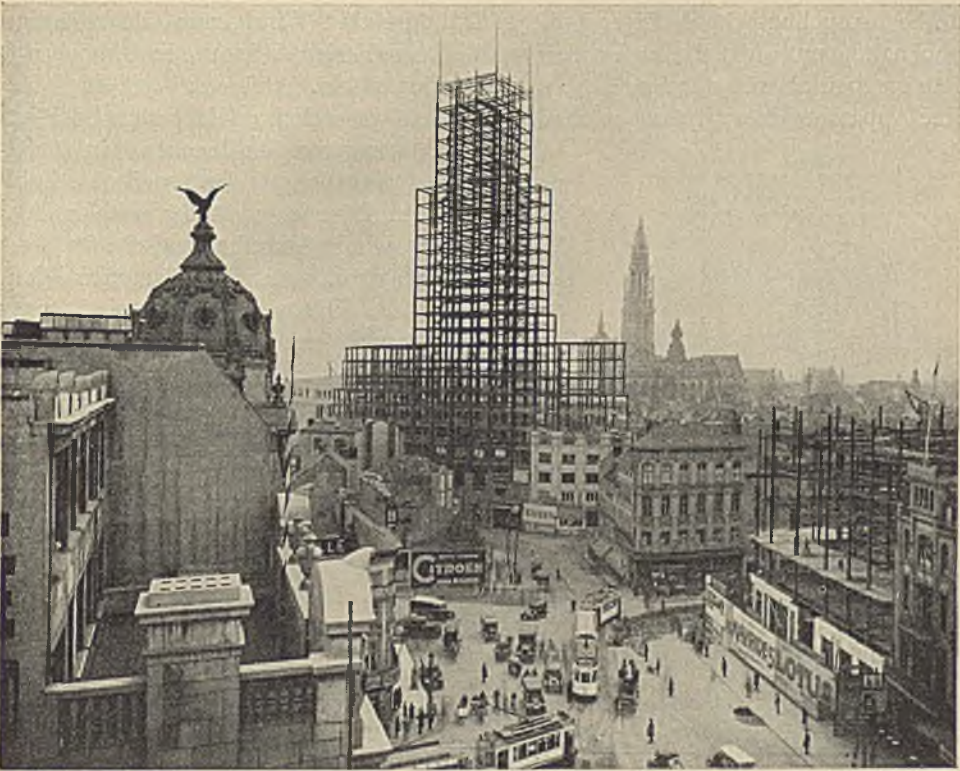
Abb. 452. Hochhaus der Allgem. Bankvereinigung in Antwerpen. Ansicht des fertigen Stahlskelettes. Ausführung: DEMAG Aktienges. Duisburg.
