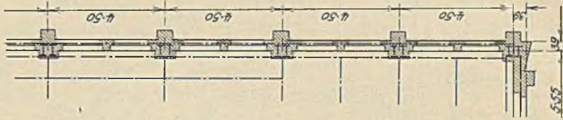
Abb. 23. Europahaus Berlin. Träger der Wandausbildung.
