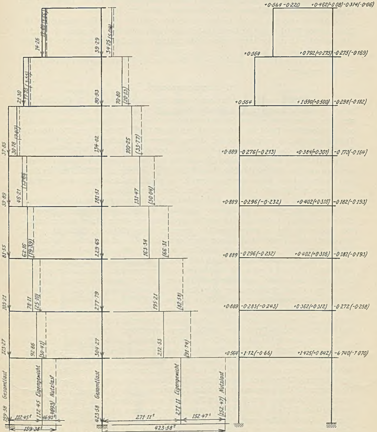
Abb. 85. Momente infolge exzentrischen Lastangriffes für Eigengewicht u. (...) Nutzlast.
