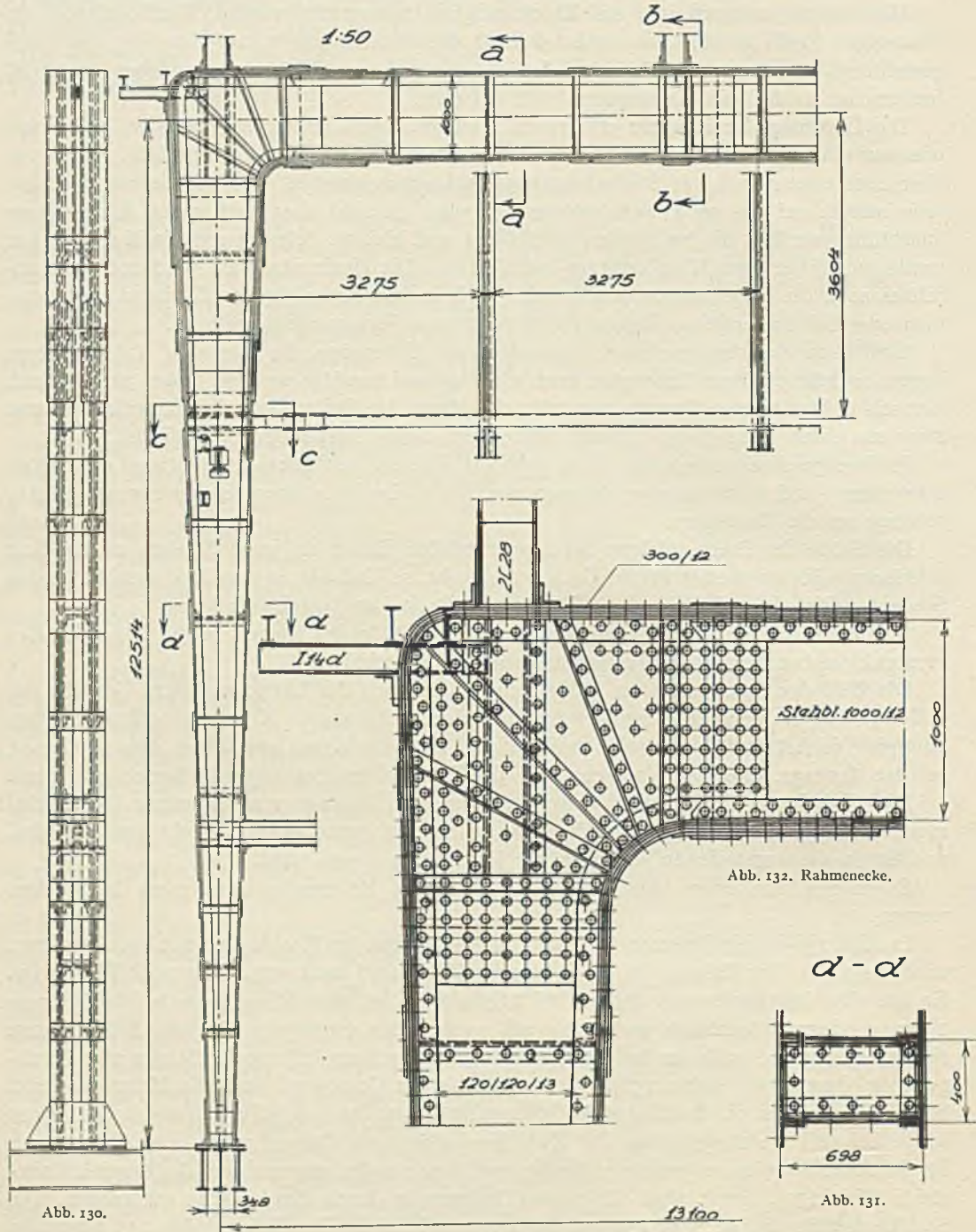
Abb. 130 bis 138, Hochhaus „Suschicky“, Prag. Rahmenträger des
