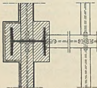
Abb. 62. Frontwandträger zentrisch gelagert (Säulenumhüllung außen vorstehend).
