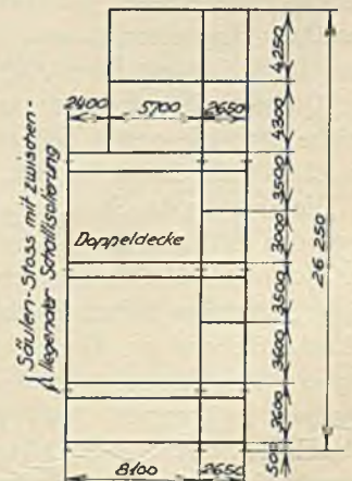
Abb. 40. Radiosendestation in Prag. Querschnitt des Gebäudeteiles „E“. Anordnung von Doppeldecken.
