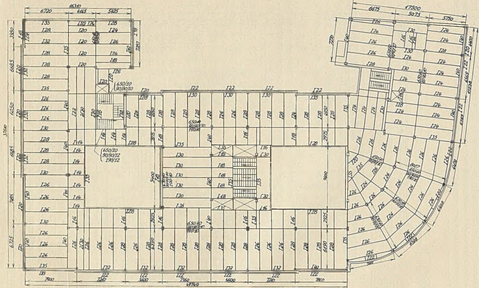
Abb. 25. Hochhaus der Berg- und Hüttenwerks-Gesellschaft in Prag. Grundriß. Trägereuteilung I. Stock. Entwurf: Dr.-Ing. Hawranek.
