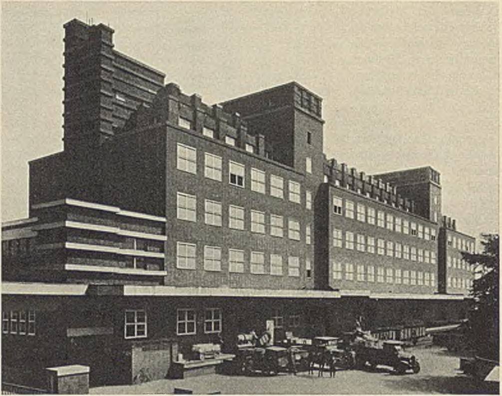
Abb. 416. Hauptlagerhaus der G. H. H. Oberhausen. Ansicht des fertigen Baues. Architekt Peter Behrens. Ausführung: Gutehoffnungshütte Oberhausen.
