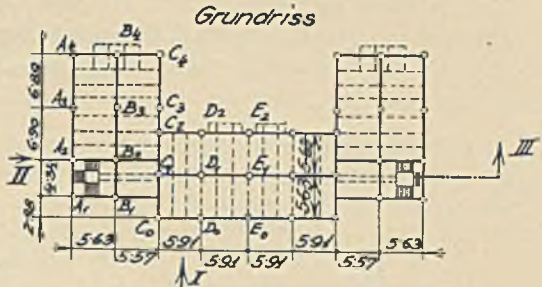
Abb. 440. Grundriß.
