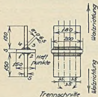
Abb. 344. Probestück zur Schweißprüfung (Stirnkehlnähte).
