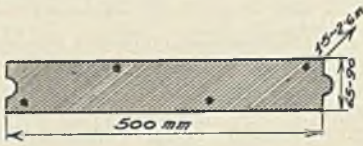
Abb. 215. Vollplatte.
