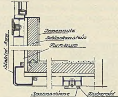
Abb. 281. Querschnitt durch die Wand des „Kästner-Hauses“.
