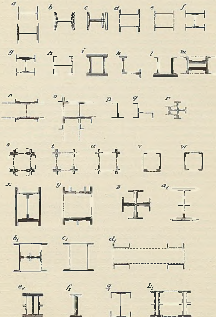
Abb. 86. Stützenquerschnitte.
