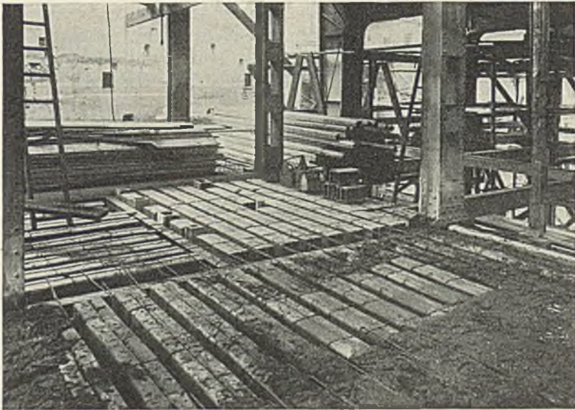
Abb. 335. Hochhaus Suschitzky Prag. Herstellung der Hohlsteindecken.
