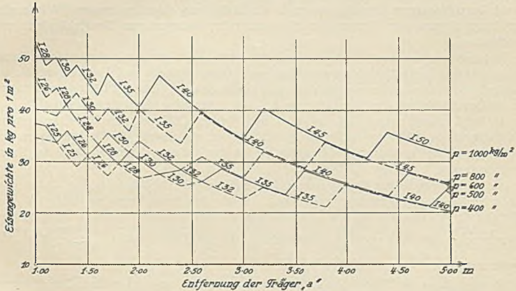
Abb. 43. Österreichische Profile.
