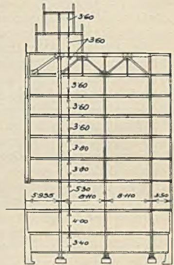
Abb. 41. Geschäftshaus „Ara“, Prag. Querschnitt. Frontteil überhängend.
