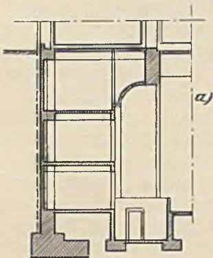
Abb. 413a und b. Hochhaus Berg- u. Hüttenwerks-Ges., Prag.
