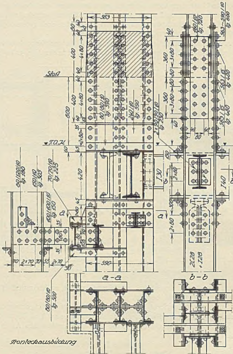
Abb. 53. Hochhaus Berg- und Hüttenwerkses., Prag. Entwurf: Dr.-Ing. A. Hawranek. Säulenstöße und Befestigung der Frontwandträger.
