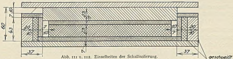
Abb. 111 u. 112. Einzelheiten der Schallsisolierung.
