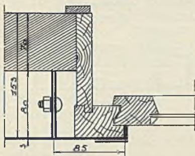
Abb. 276. System „Blecken“. Fensteranschluß.
