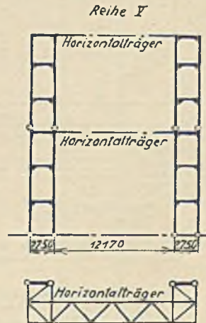
Abb. 428. Rahmenverbände. Horizontallträger.
