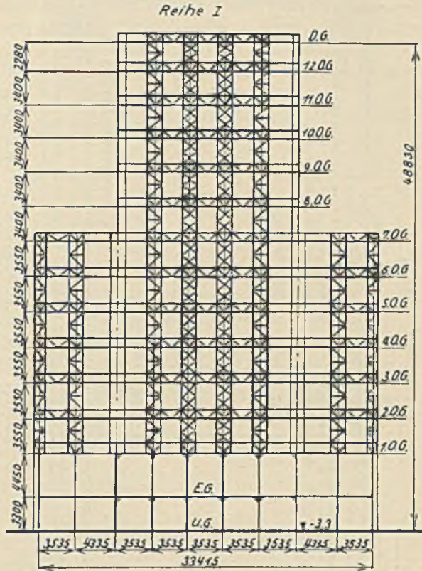
Abb. 426. Aufriß. Wandverbände.
