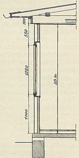
Abb. 275. Stahlhaus System „Blecken“, Düsseldorf.
