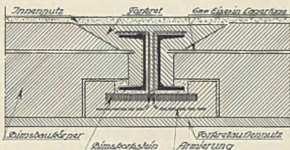
Abb. 269. Wohnhausbau. Torkret-Bauweise. Konstruktion einer Stütze.
