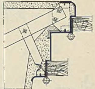
Abb. 300. Doppeltür.
