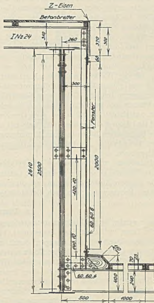
Abb. 296. Walzwerkhalle.
