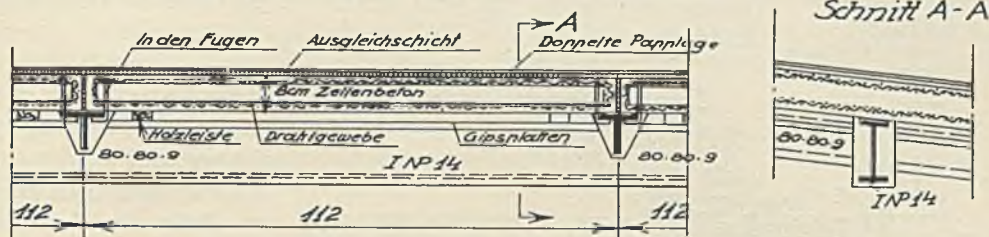
Abb. 246. Dachkonstruktion eines Hamburger Hauses. Aus „Der Zellenbeton“.
