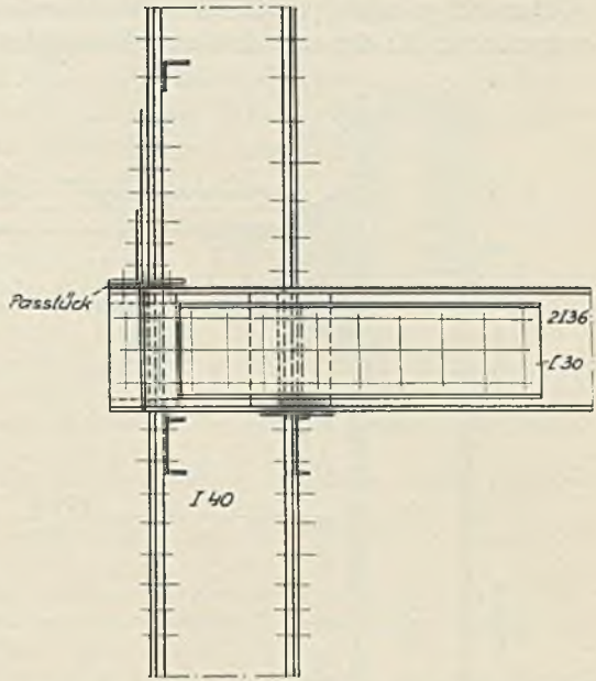
Abb. 169. Verwaltungsgebäude des Deutschnaf. Handlungsgehilfen-Verbandes in Hamburg. (Nach Timm, G.: Der P-Träger 1930.)
