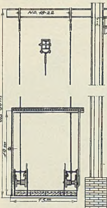
Abb. 313. Torkret-Schnellbaurüstung D.R.P. a. Querschnitt.
