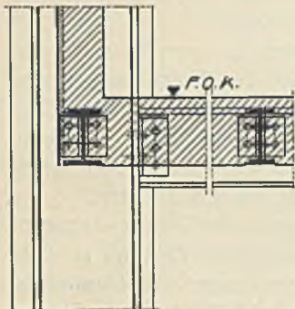
Abb. 60. Ausladender Deckenträger.
