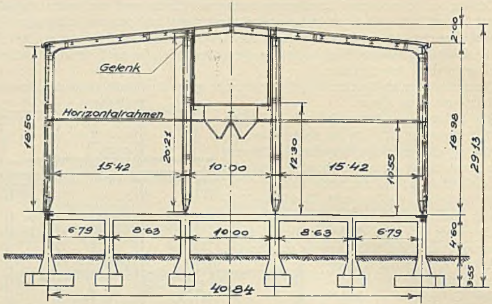
Abb. 38. Kesselhaus Oberlandzentrale „Oslawan“. Querschnitt. Zweigelenkranken mit zwei Pendelzwischenstützen. Entwurf: Dr.-Ing. A. Hawranek.
