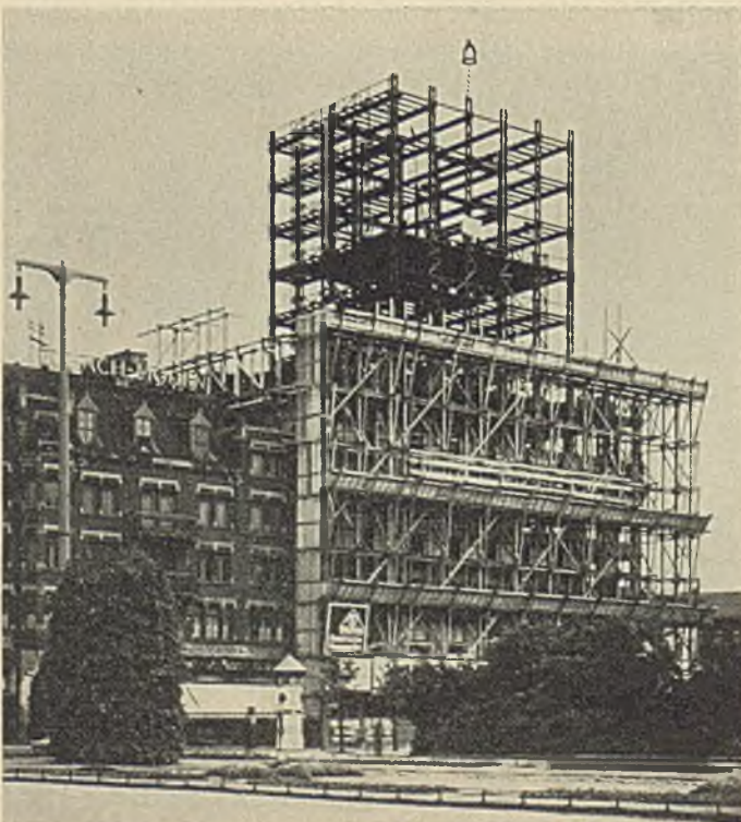
Abb. 8. Europabau in Leipzig. Architekt O. P. Burghardt, Leipzig. Ausführung des Stahlskelettes: Vereinigte Hüttenwerke Burbach-Eich-Düdelingen.
