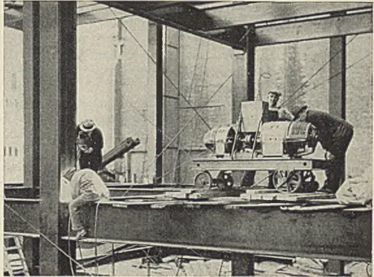
Abb. 341. Lichtbogenschweißung eines Stahlskelettes. Fahrbarer Schweißumformer. (Aus V. d. I.-Nachrichten 1930.)
