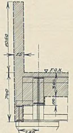
Abb. 81. Detail „A“.
