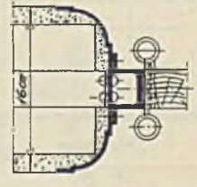
Abb. 298. Pendeltür.
