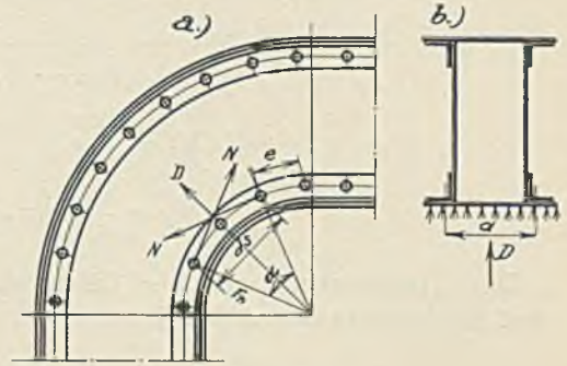
Abb. 127. Rahmenecke.
