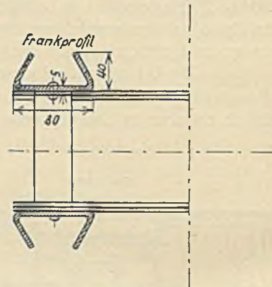
Abb. 430. Wandstützenquerschnitt nach Frank.
