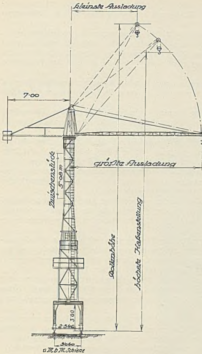
Abb. 310. Wolfkran.
