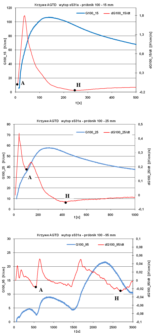
Rys. 4. Wykresy gradientu temperatury i jego pochodnej (krzywe AGTD) badanego żeliwa chromowego na przekrojach odlewu modelowego oddalonych o 15; 25 i 95 mm od powierzchni formy
