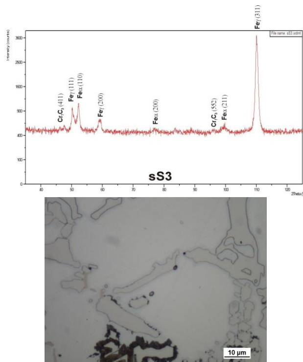
Rys. 3. Dyfraktogram rentgenowski i zdjęcie struktury żeliwa chromowego podutektycznego- wytop sS3
