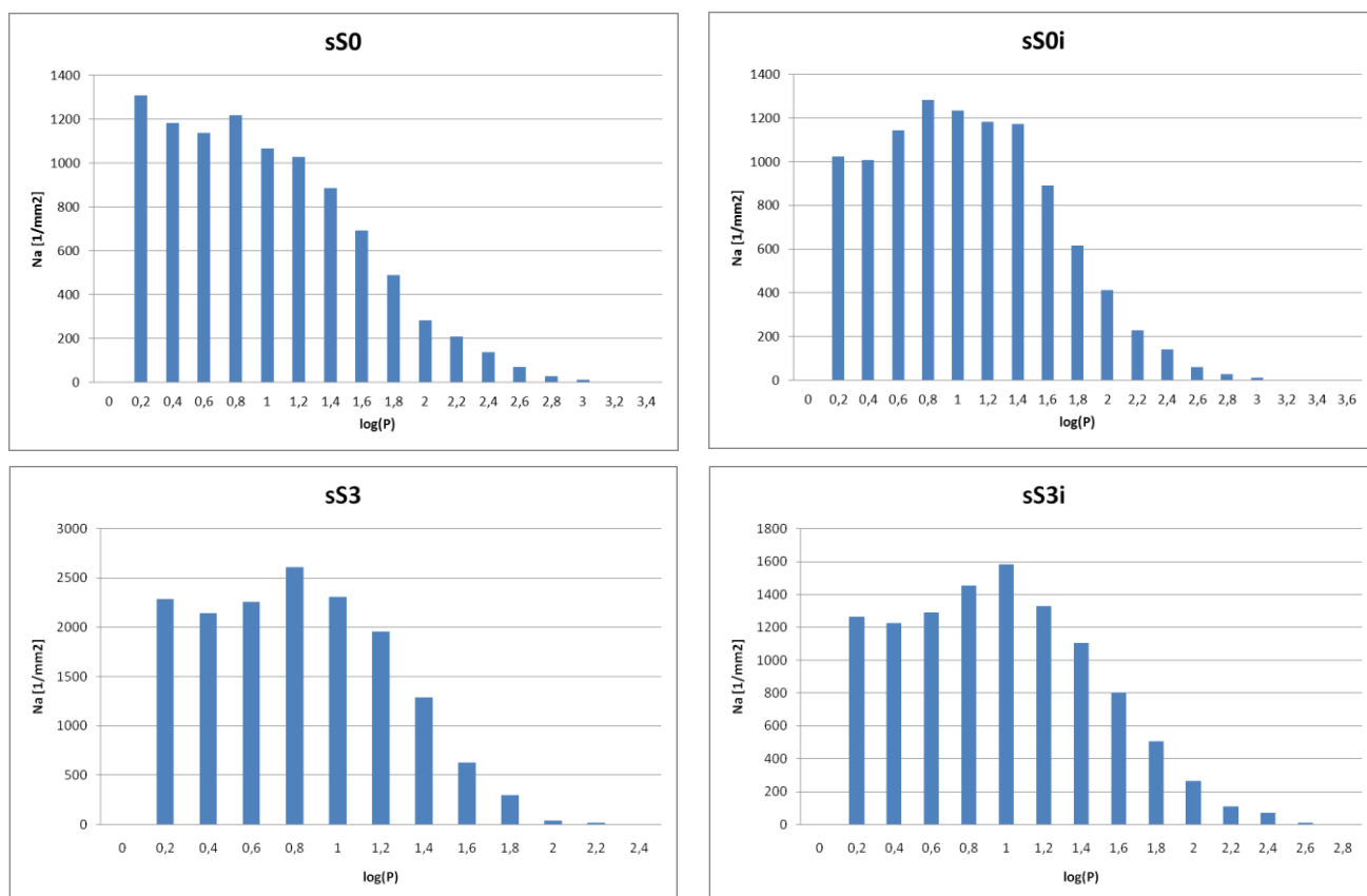
Rys. 4. Histogramy rozkładu ilości węglków Na w klasach ich wielkości P – żeliwo podeutektyczne niemodyfikowane sS0 oraz modyfikowane mieszaniną FeNb+FeV+MZR – sS3
