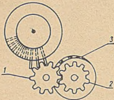
Rys.6. Zasada rejestracji liczby za pomocą koła Odhnera 1- zębatka pośrednia, 2- zębatka koła cyfrowego, 3- koło cyfrowe
