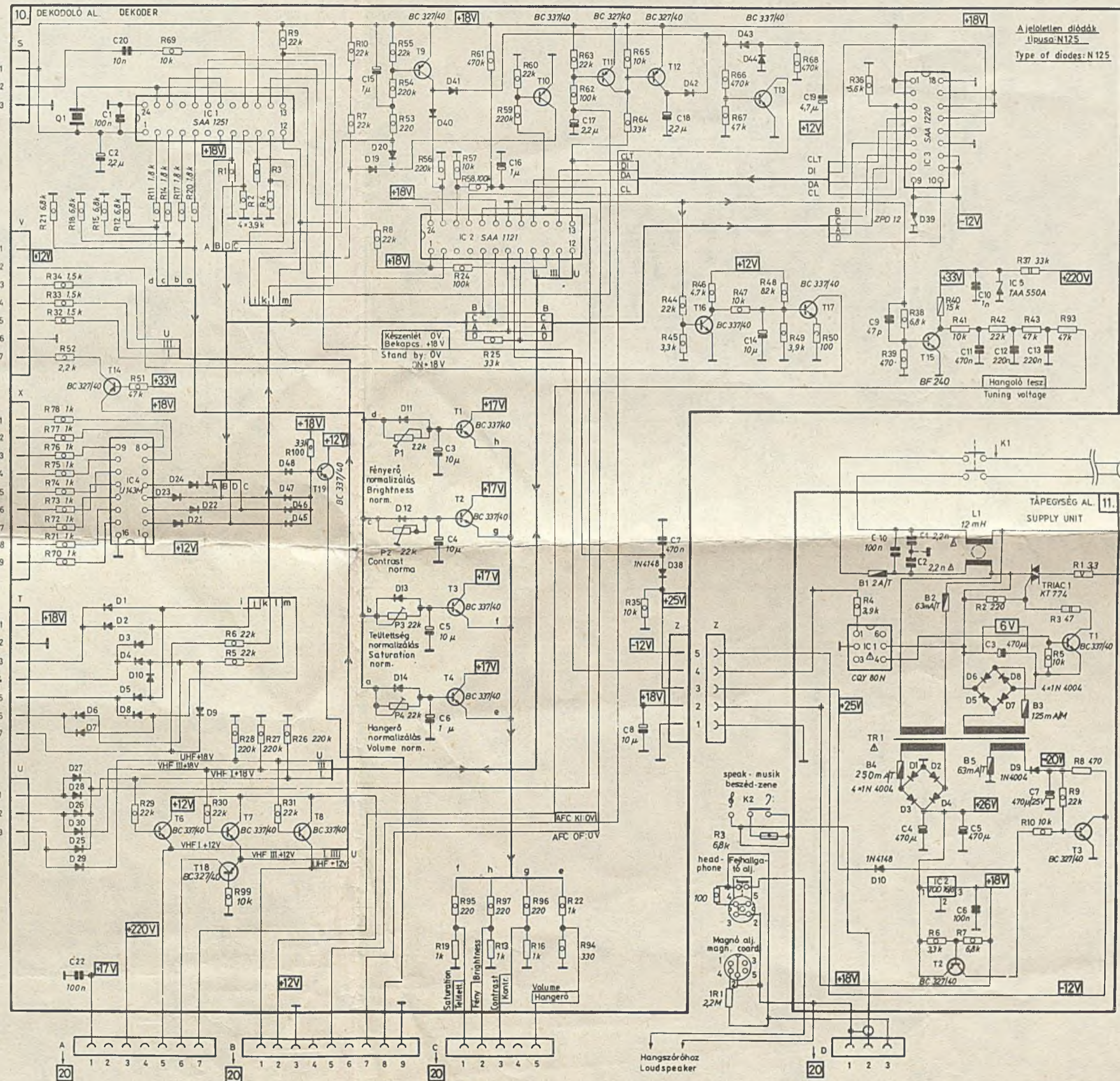
ELVI KAPCSOLÁSI RAJZ CIRCUIT DIAGRAM 2. side
