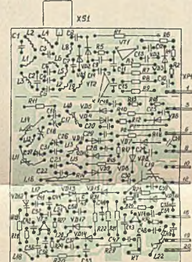
Селектор каналов СК-М-30
