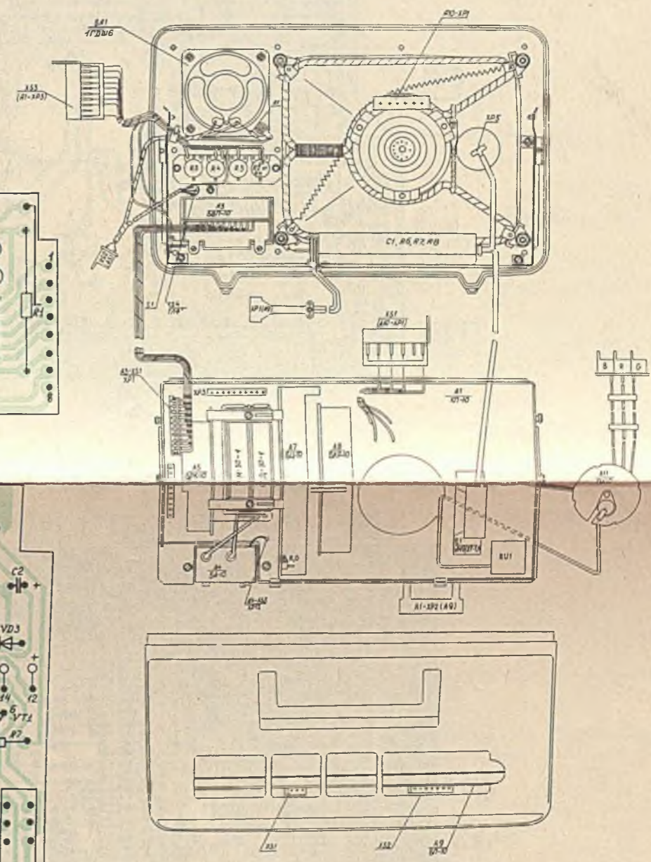
Схема расположения блоков
