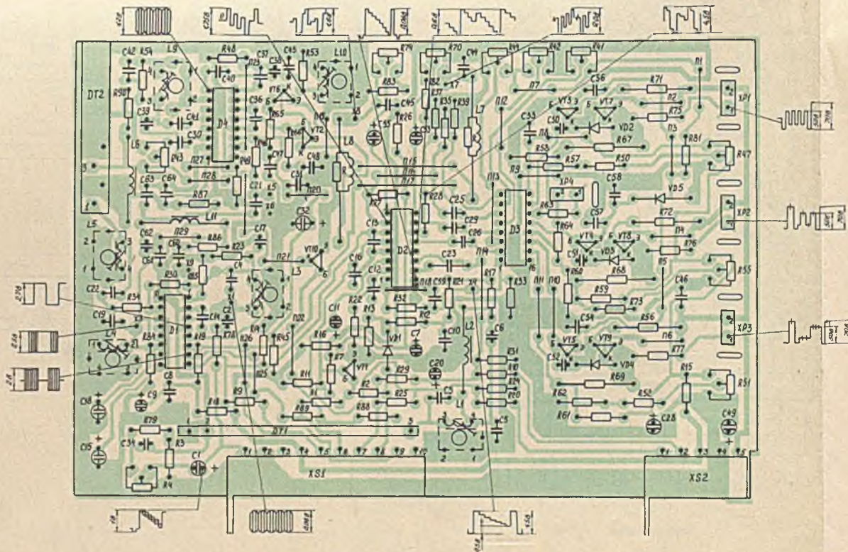
Блок цвета (BC-10)
