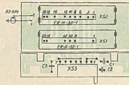
Селектор каналов СК-Д-30
