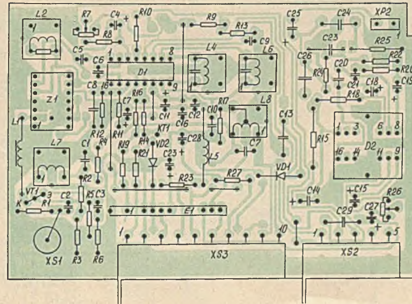
Блок радиоканала (BRK-10-2)
