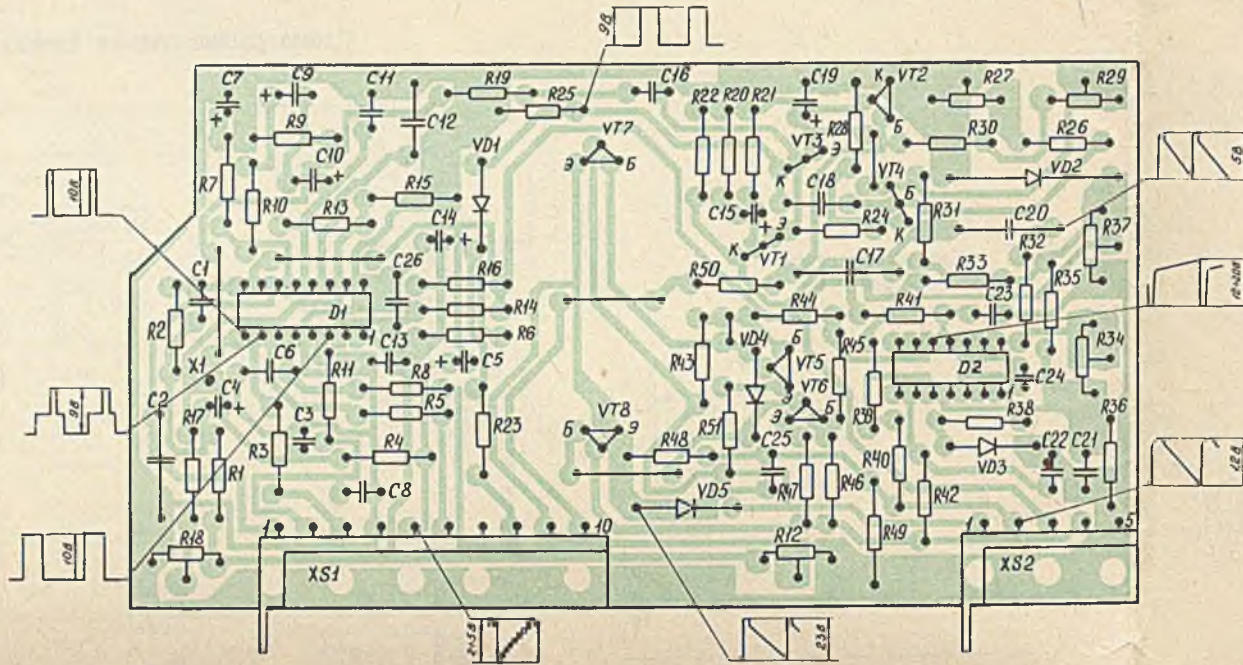
Блок кадровой развертки (ВКР-10)
