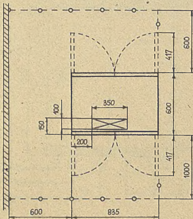
Rys. 3. USYTUOWANIE JEDNOSTKI STERUJĄCEJ EC 7911
