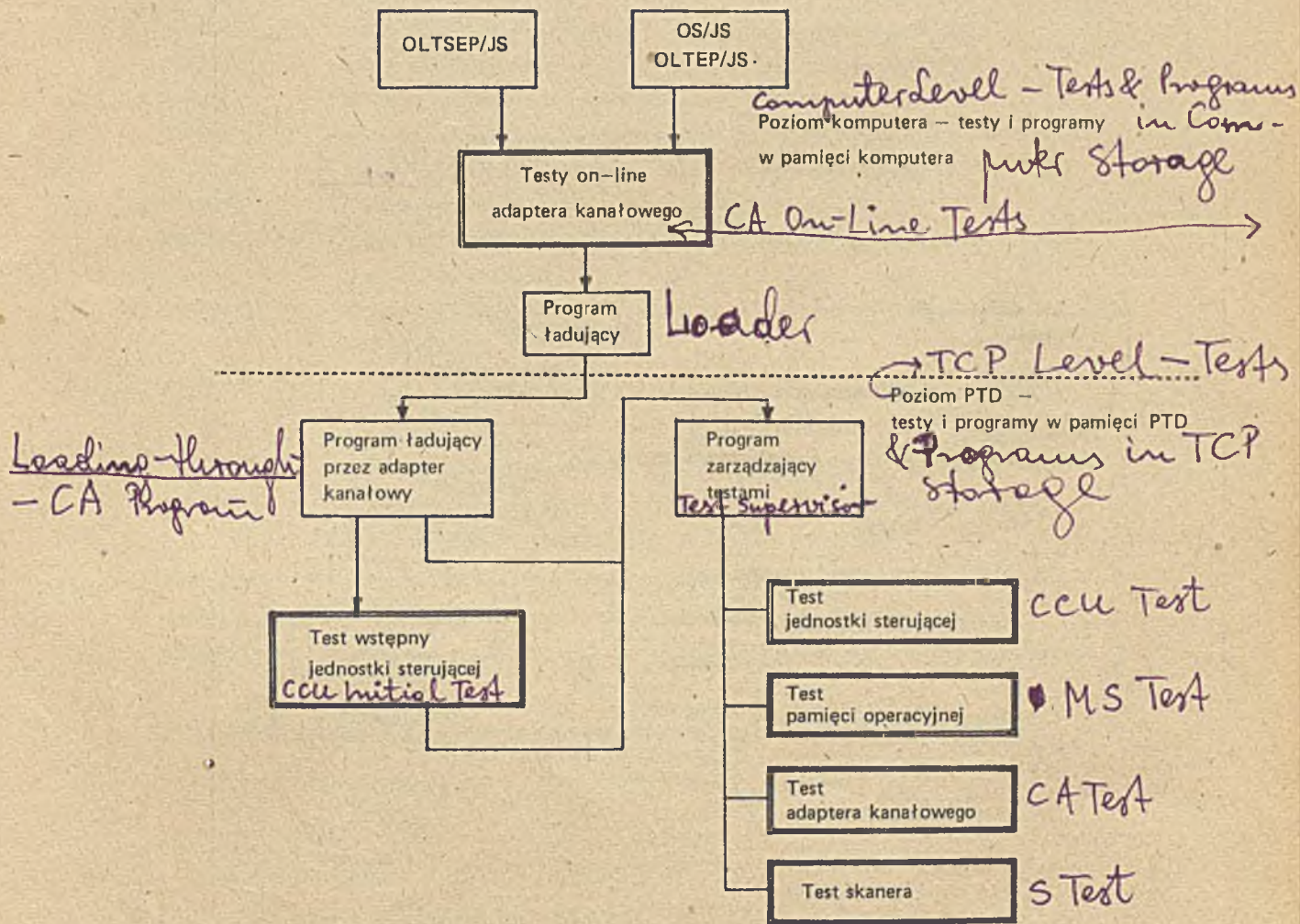
Fig. 8. Block-Functional Diagram of TCP Test Set Rys. 8. SCHEMAT BLOKOWO-FUNKCJONALNY ZESTAWU TESTÓW PTD
