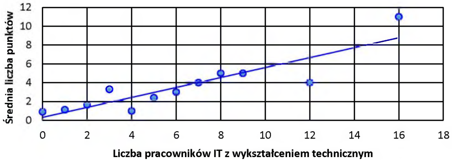
Rys. 13. Zależność stopnia wdrożenia przepisów KRI dotyczących zarządzania usługami realizowanymi za pomocą systemów teleinformatycznych od liczby pracowników IT z wykształceniem wyższym technicznym
