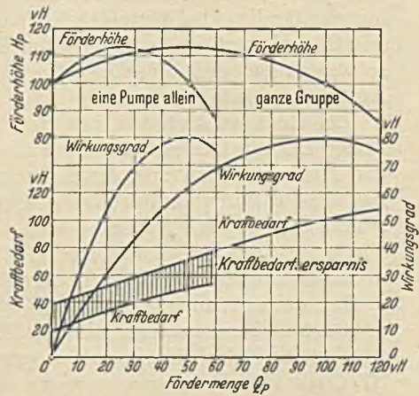
Abb. 376. Leistungskennlinien für eine Zwillingspumpspeicherpumpengruppe mit einer zu- und abschaltbaren Pumpe (Tremorglio).
