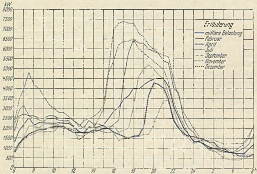
Abb. 7. Durchschnittlicher Monatslastverlauf eines Betriebsjahres für ein mittleres Kraftwerk mit vorwiegendem Licht- und Gewerbeanschluß ohne größere Industriebelegung.
