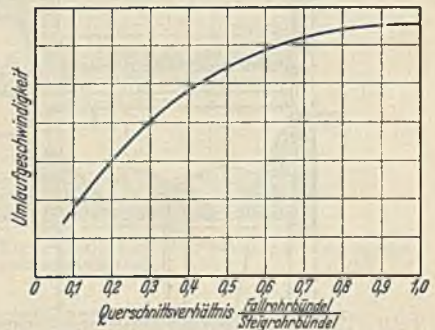
Abb. 127. Wasserumlaufgeschwindigkeit in Abhängigkeit vom Querschnittsverhältnis des Fallrohr- zum Steigrohrbündel.
