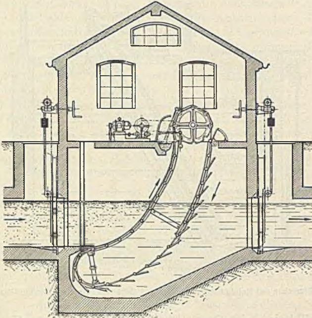
Abb. 74. Siebbandrechen mit Reinigungsvorrichtung und elektromotorischem Antrieb (Bauart Geiger).
