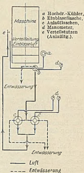
Abb. 287 e. Luftleitung.
