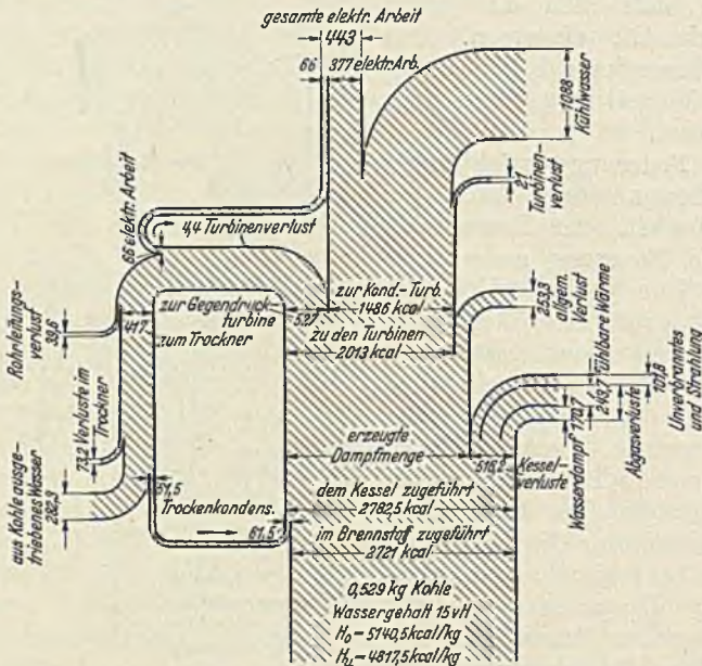
Abb. 156. Wärmestrombild für Verfeuerung von 1 kg Rohbraunkohle in getrocknetem Zustand mit 15 vH Wassergehalt in einer Kohlenstaubeuerung, Trocknen durch Dampf einer Gegendruckturbine.
