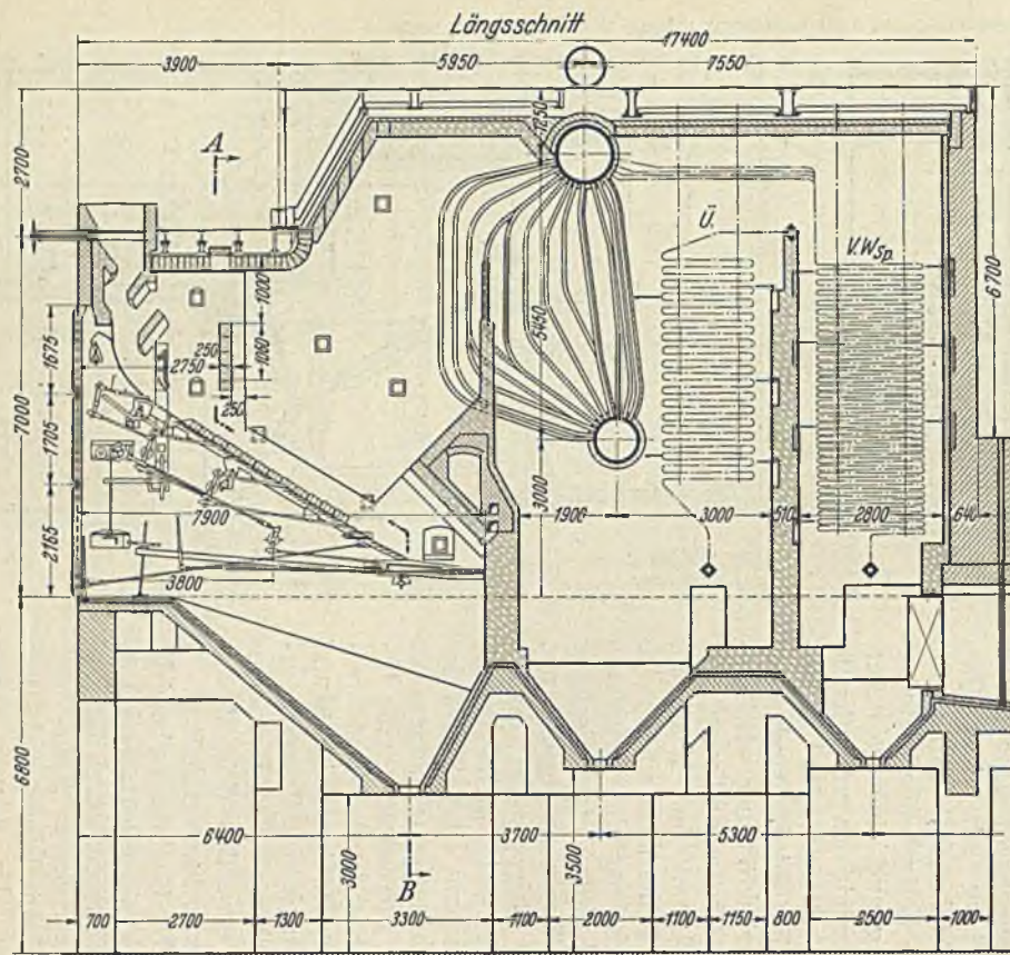
Abb. 160. Keilmann & Vöcker-Halbgasfeuerung für Steilrohrkessel.
