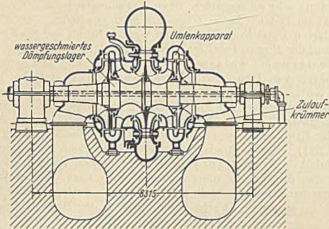
Abb. 369. Querschnitt durch eine zweistufige Speicherpumpe mit zwei einfachen Laufrädern in der ersten und einem Doppelrad in der zweiten Stufe. 33200 PS, H_P = 140 bis 167 m, Q_P = 14,88 bis 13,16 m^3/s , Stufendruck je 80 m, n = 300 U/min (Volth).
