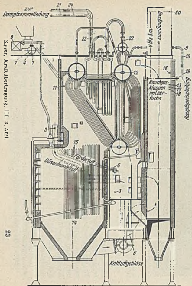
Abb. 220. Meßstellen zur wärmetechnischen Betriebsüberwachung eines Stellrohrkessels mit Kohlenstaubfeuerung.
