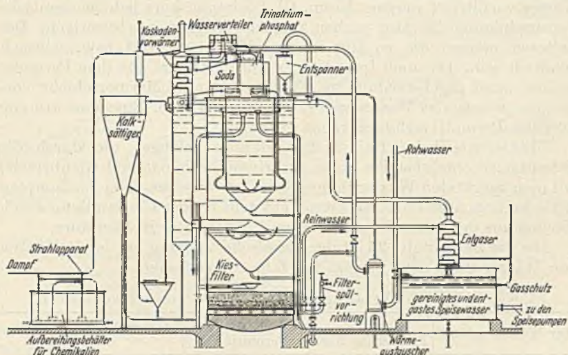
Abb. 104. Babcock-Speisewasseraufbereitungsanlage mit Entgaser und Gasschutz nach dem Kalk-Soda-Trinitriumphosphat-Verfahren.
