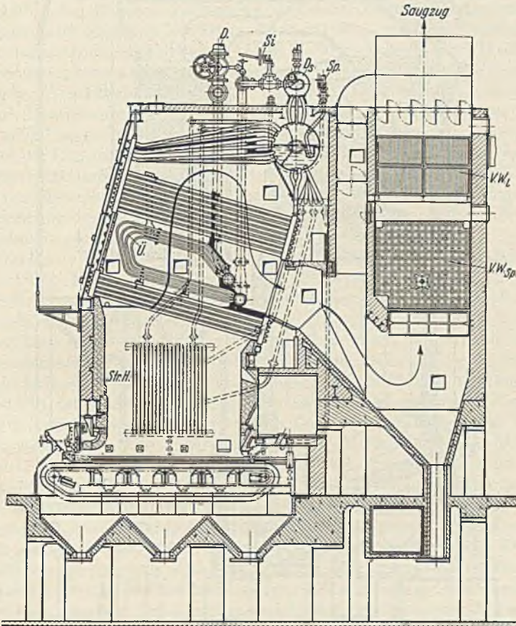
Abb. 119. Steinmüller-Teilkammer-Hochleistungskessel mit querliegender Obertrommel hinten, mit Unterwind-Zonenwandlerrost, Strahlungheizfläche (Str. H.), Überhitzer, Rippenrohr-Speisewasservorwärmer 1978 m 2 und Luftvorwärmer 860 m 2 (Saugzuganschluß) (1000 m 2 Heizfläche, 26,5 atü, 400° C, Rostbreite 6 m, Rostlänge 5,6 m).
