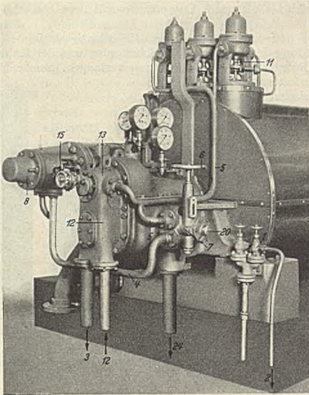
Abb. 40. Ansicht einer gestängellosen BBC-Turbinen-Öldrucksteuerung mit ölgesteuerter Hauptabschließung.
