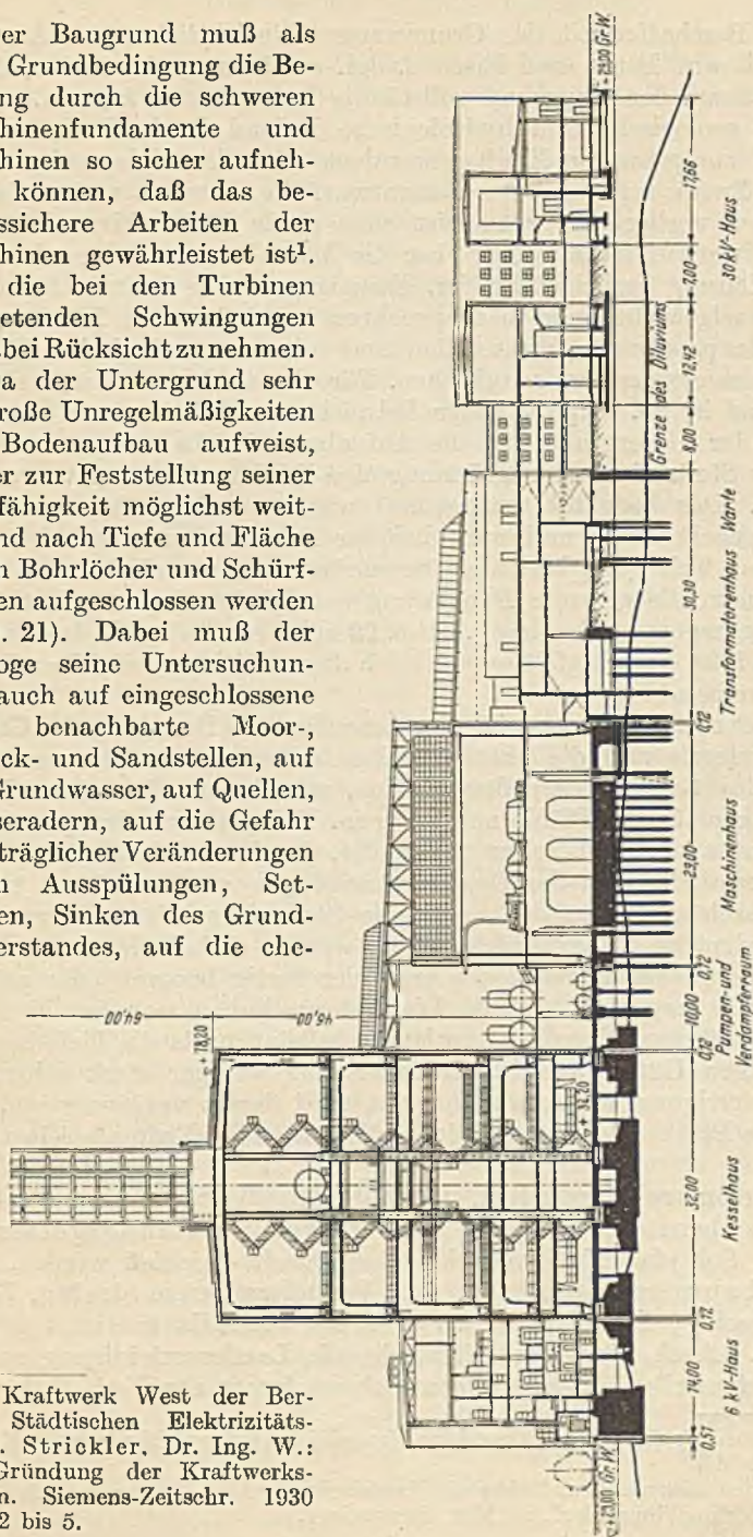
Abb. 22. West-Ost-Querschnitt durch den Kraftwerkblock mit Fundierung des Kraftwerkes West der Bewag.
