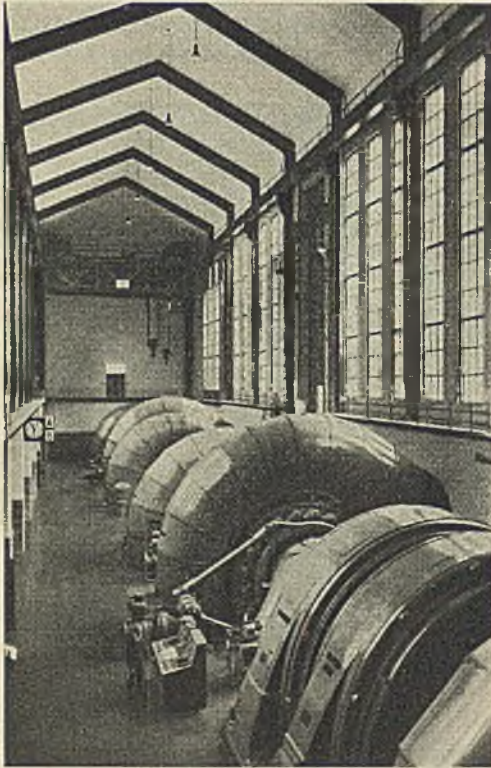
Abb. 359. Blick in den Maschinenraum des Bleiloch-Pumpapfelcherkraftwerkes.
