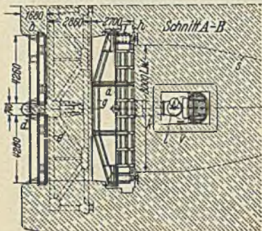
Abb. 354. Einlaufbauwerk in der Sperrmauer der Saaleletzsperre am Bleiloch.
