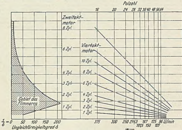
Abb. 281. Zulässiger Ungleichförmigkeitsgrad für gleichmäßiges Licht in Abhängigkeit von der Bauform des Dieselmotors.
