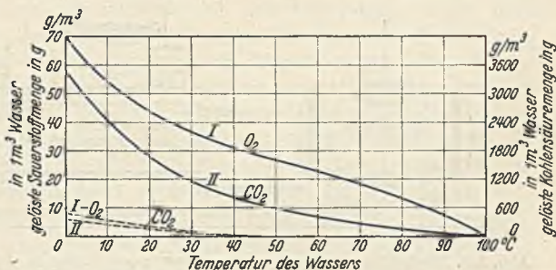
Abb. 107. Kohlensäure- und Sauerstoffaufnahme von reinem Wasser bei verschiedenen Wassertemperaturen (bei Lösungen Luft in Wasser beträgt die Aufnahme etwa \frac{1}{2} der Werte).
