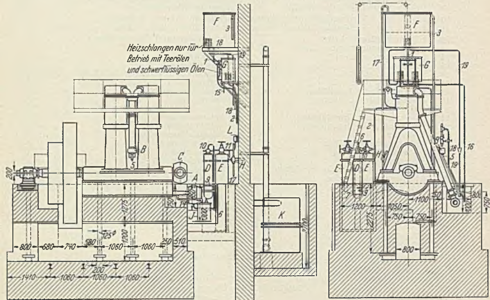
Abb. 287a. A Kühlgefäß, B Ablauftrichter, C Einblaspumpe, D Einblasflasche, E Anlaßflasche, F Brennstoff-Vorratsbehälter, G Brennstoff-Filtergefäße, H Brennstoff-Handpumpe, J Schmutzöl-Sammeltopf, K Auspufftopf, L Druckmesser.
