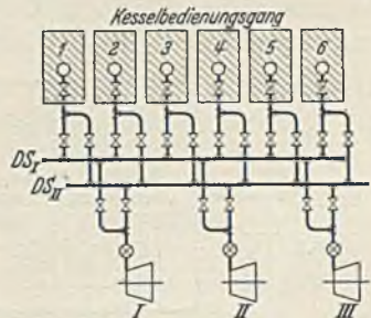
Abb. 197. Rohrleitungsplan, Doppelsammelleitung.
