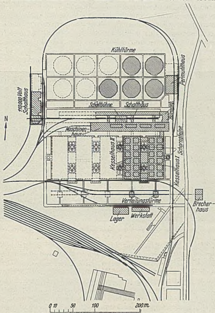
Abb. 249. Großkraftwerk Fortuna II der „Rheinisches Elektrizitätswerk im Braunkohlenrevier A.G.“ Köln. 2 Kesselhäuser mit Stellrohrkesseln 15,5 atü, 375° C, Treppenrostfeuerung, Rohbraunkohle 1800 kcal/kg, 5 Turbosätze zus. 115 000 kVA, 6,3 kV Drehstrom. Voller Ausbau 230 000 kVA.
