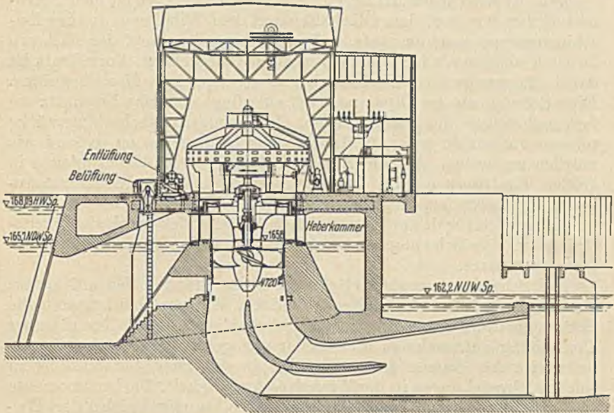
Abb. 346. Einbau einer Kaplan turbine in eine Heberkammer.
