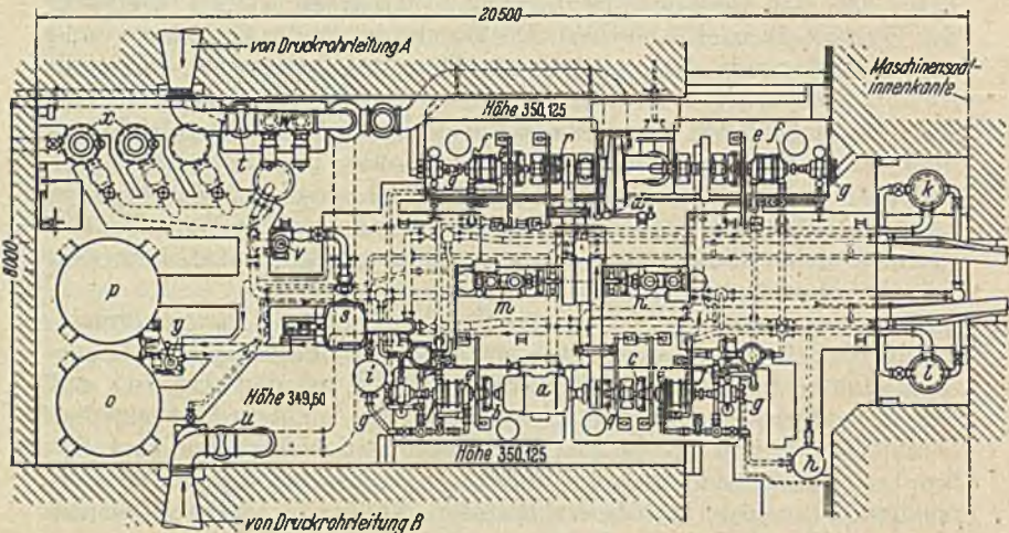
Abb. 357. Grundriß des Hilfsmaschinenraumes des Biebloch-Pumpspeicherkraftwerkes.
