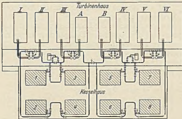
Abb. 202. Frischdampf-Rohrplan für ein Großkraftwerk.
