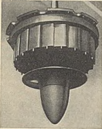
Abb. 336. Kaplanturbine, Leitapparat und Laufrad geschlossen.
