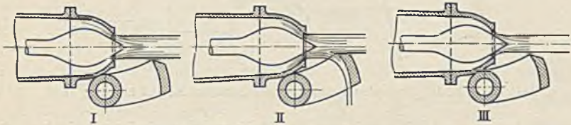
Abb. 328. Doppelregelung mit Strahlablenker.
