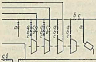
Abb. 224b. Das dritte Feld der Meßtafel Abb. 224a mit eingetragenem Meßstellen für Wassermenge (a) Temperatur (b) und Druck (c).
