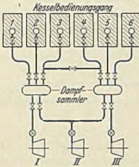
Abb. 198. Dampfsammler.
