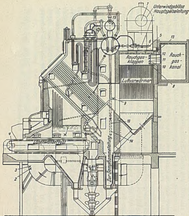
Abb. 219. Meßstellen zur wärmetechnischen Betriebsüberwachung eines Schrägrohrkessels mit Wanderrost, Unterwind und Luftvorwärmer.
