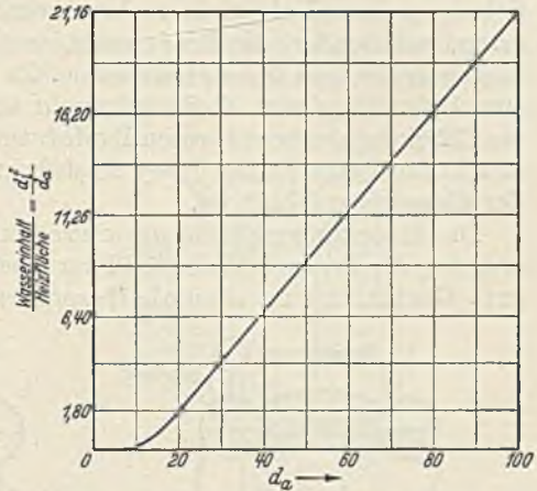
Abb. 122. Verhältnis des Wasserinhaltes ( d_i = innerer Siederohrdurchmesser) zur Heizfläche ( d_a = äußerer Siederohrdurchmesser) in Abhängigkeit von der Heizfläche bei Siederohren.
