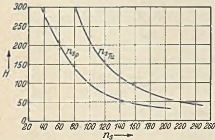
Abb. 366. Grenzl意思 für die spezifische Drehzahl der Turbinen und Pumpen.
