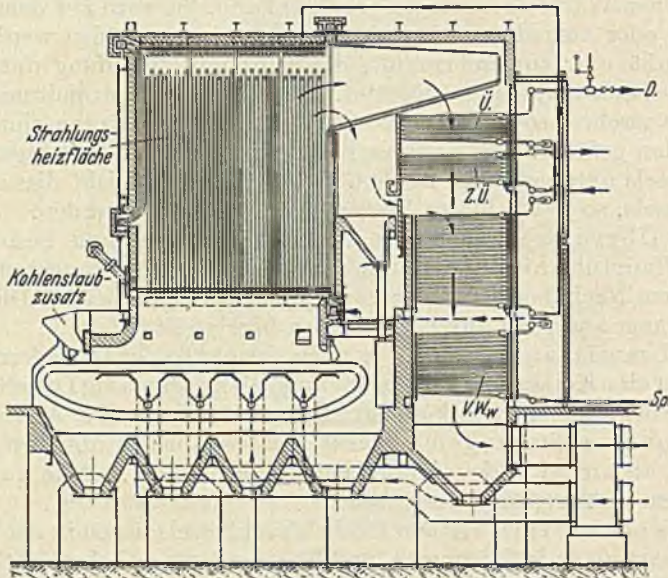
Abb. 140. S.S.W.-Bensonkessel mit Unterwindzonenwanderrost und Kohlenstaubzusatzfeuerung (ZÜ Zwischenüberhitzer).
