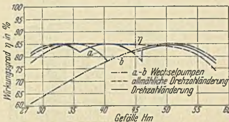
Abb. 378. Wirkungsgradverlauf für verschiedene Pumpenausführungen.
