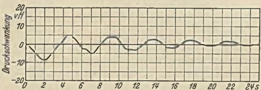
Abb. 373. Abschalten einer Speicherpumpe mit Schwungmassenwirkung.
