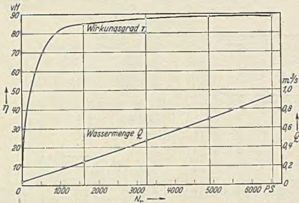
Abb. 327. Wirkungsgradkennlinie einer EWC-Freistrahlturbine, H_n = 600 m, Q = 0,94 m^3/s , N_n = 6200 PS, n = 500 U/min, n_s = 13,31 .
