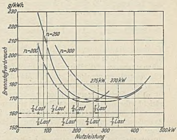
Abb. 273. Brennstoffverbrauch eines Sechszylinder-Dieselmotor ohne Verdichter, 275 bis 370 \text{PS}_e , 275 bis 370 kW, n = 215 bis 300 U/min.
