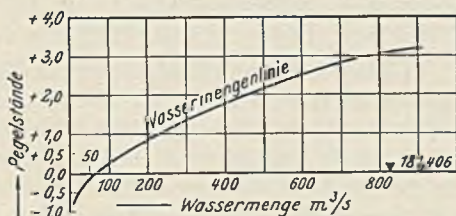
Abb. 313. Wassermengenlinie zu Abb. 310 nach Pegelangaben.
