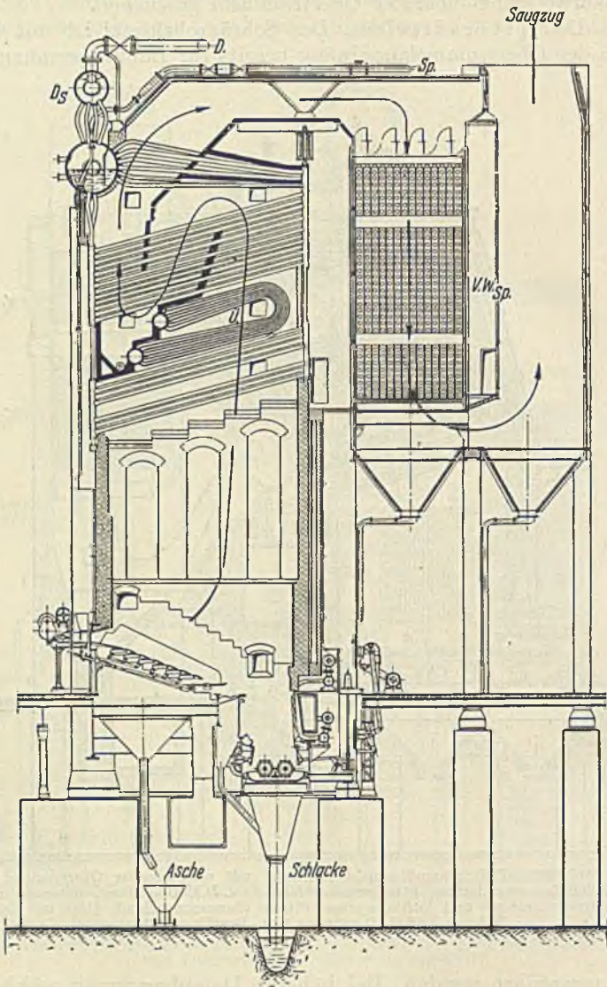
Abb. 120. Borsig-Teilchammerkessel mit querliegender Obertrommel vorne, 1850 m 2 Heizfläche, 32 atü, 400° C, mit Stokerfeuerung, Überhitzer und Rippenrohr-Speisewasservorwärmer (Saugzugsanschluß).
