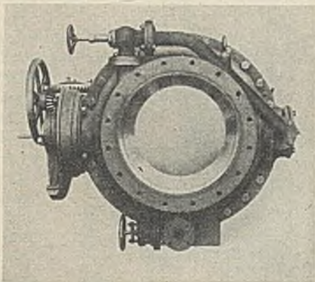
Abb. 353a. Kugelschieber mit Handantrieb, geöffnet.
