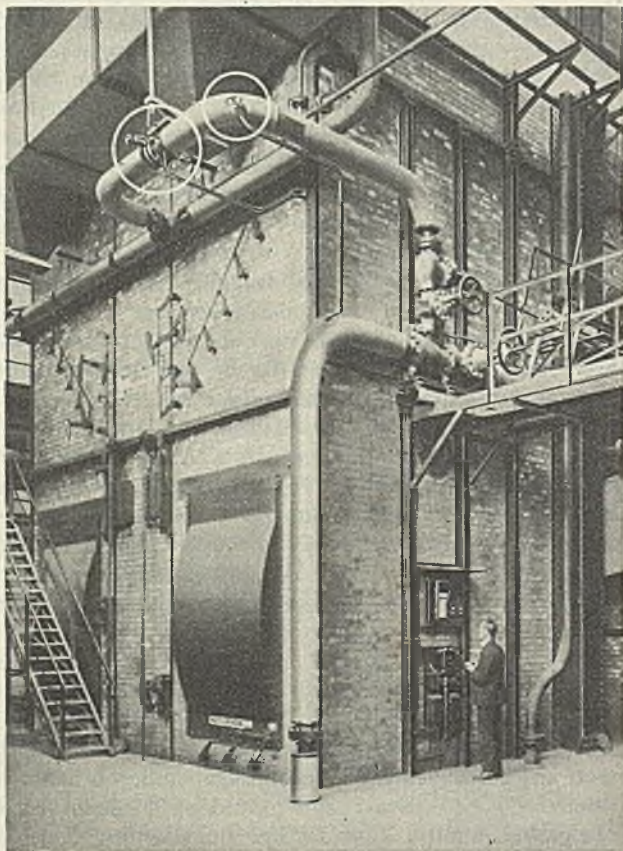
Abb. 217. Dampfmenagemessung durch Meßflansch und Dampftemperaturmessung mit schreibendem Anzeigerät.
