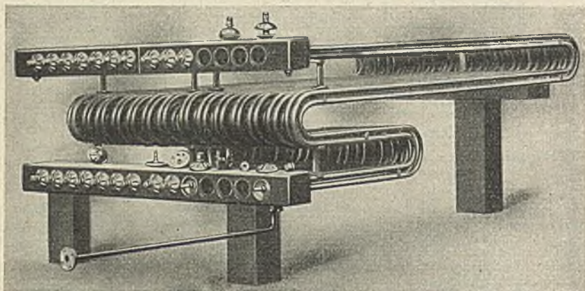
Abb. 170. Dampfüberhitzer (Berührungsoberhitzer).
