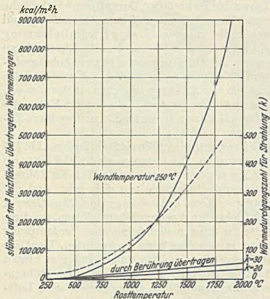
Abb. 121. Wärmedurchgang durch Strahlung und durch Berührung in Abhängigkeit von der Feuerraumtemperatur.
