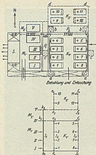
Abb. 253. Gesamtentwurf I eines Kraftwerkes mit Rohrplan. Maschinen- und Kesselhauslängsachsen parallel.
