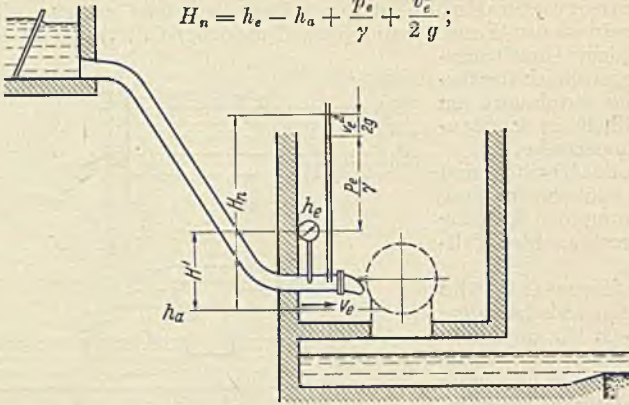
Abb. 319. Freistrahlturbine mit Druckrohrleitung und Freihang.
