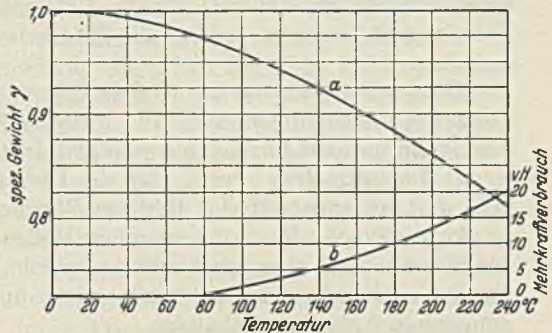
Abb. 216. Spezifisches Gewicht des Wassers in Abhängigkeit von der Temperatur (a) und Erhöhung des Pumpenkräftebedarfes bei Wassertemperaturen über 80° C (b).
