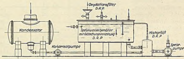
Abb. 108. Mischanlage für Kondensat und Zusatzspeisewasser in einem mit Gasschutz versehenen Speisewasserbehälter (Bauart Balcke).
