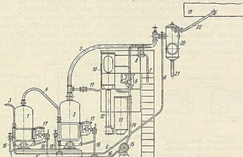
Abb. 106. Verbund-Verdampferanlage mit Rohwasservorreinigung und Mischdüse (Bauart Atlaswerke, Kiel.)
