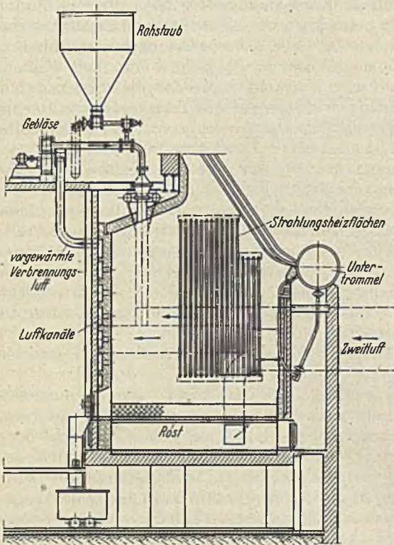
Abb. 167. Vereinigte Kesselwerke A. G. Rohkohlensaubfeuerung für einen Stellrohrkessel.
