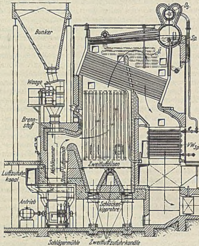
Abb. 168. Borsig-Mühlenernung (Patent Krämer).
