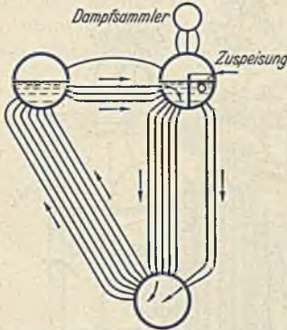
Abb. 125. Unrichtige Lage der Fallrohre.
