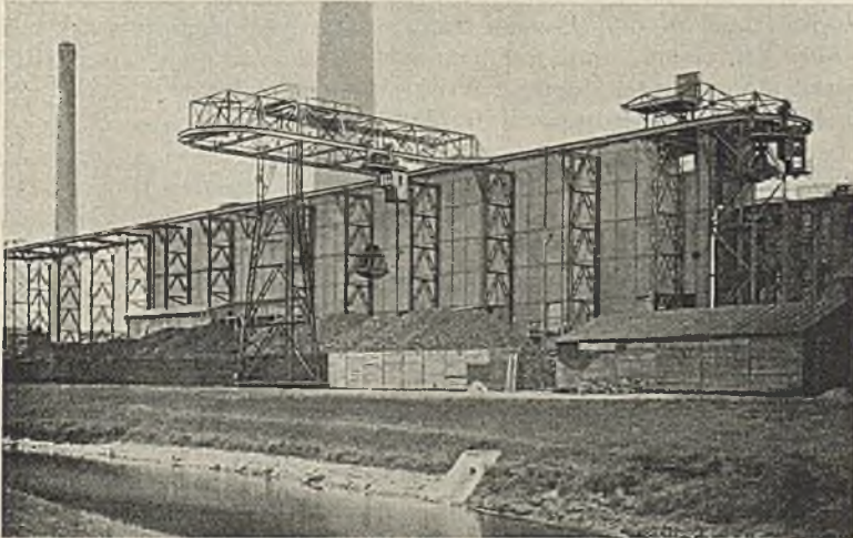
Abb. 232. Elektrohängebahn mit 2 Führerstandsgreiferkatzen, Stundenleistung je 15 t.
