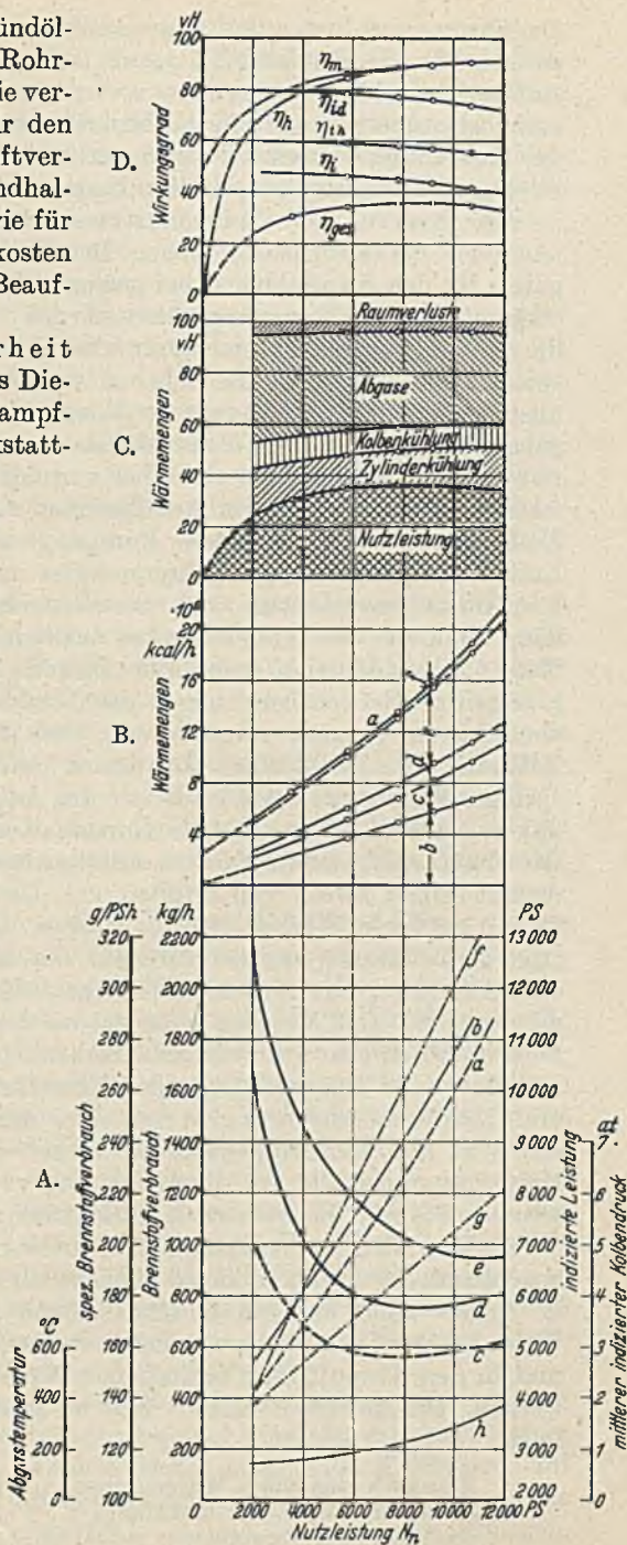
Abb. 290. Betriebskennlinien für einen 12000 PS doppelwirkenden Zweitakt-Dieselmotor (MAN).
