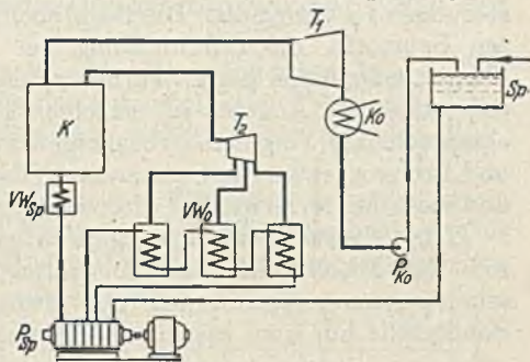
Abb. 206. Schaltplan einer Kesselspeisanlage mit vereinigter Vorwärm- und Speisepumpe.
