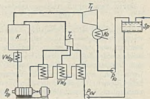
Abb. 207. Schaltplan einer Kesselspeisanlage mit besonderer Vorwärmerpumpe vor der Hauptspeisepumpe. K Kessel, T_1 , T_2 Turbinen, Ko Kondensator, P_{Ko} Kondensatpumpe, P_{Sp} Speisepumpe, P_{VW} Vorwärmerpumpe, VW_0 Oberflächenvorwärmer, VW_{Sp} Speisewasservorwärmer, Sp Speisewasserbehälter.
