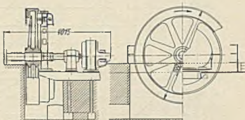
Abb. 278. Außenpolgenerator.
