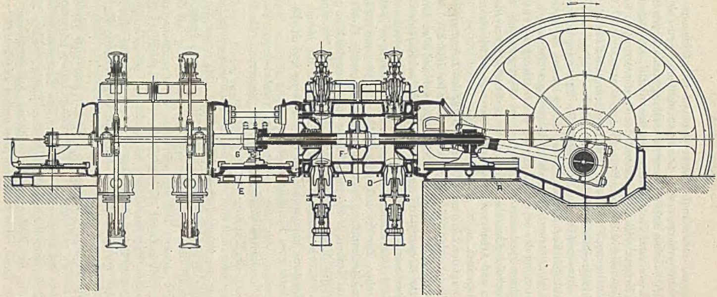
Abb. 291. Längsschnitt einer 3000 PS doppeltwirkenden MAN-Großgasmaschine.
