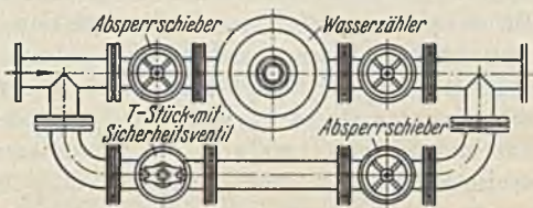
Abb. 220. Einbau eines Wasserzählers mit Umgehungsleitung und Absperrschieber.
