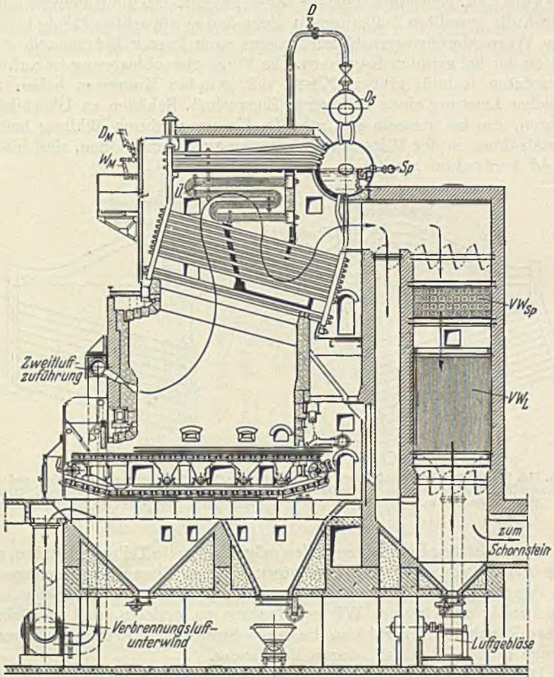
Abb. 118. Babcock-Teilkammer-Hochleistungskessel mit querlegender Oberstrommel hinten, mit Unterwind-Zonenwandlerrost, Zweitluftzuführung, Überhitzer, Rippenrohr-Speisewasservorwärmer und Luftvorwärmer (Schornsteinanschluß).
