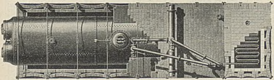
Abb. 181 a. Topfsche Bogenform-Einmauerung eines Flammrohrkessels.
