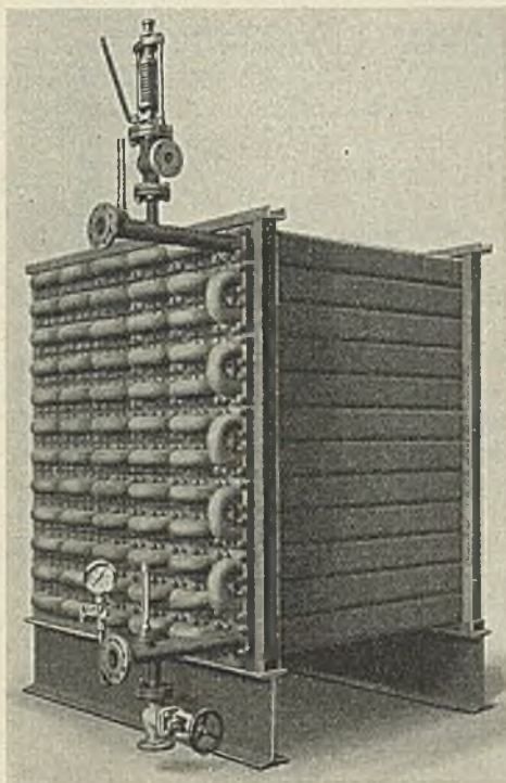
Abb. 174. Rippenrohr-Speisewasservorwärmer (Bauart Babcock).
