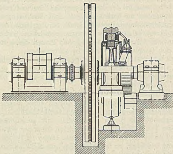
Abb. 293. Gleichstromgenerator mit Schwungrad und Schaltkranz für Gasmotorenantrieb.
