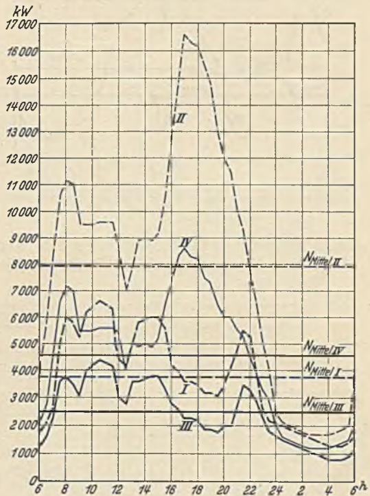
Abb. 5. Lastverlauf eines mittleren Kraftwerkes für Stadt- und Landbelleferung an einem Wochentage des hellsten und dunkelsten Monates.
