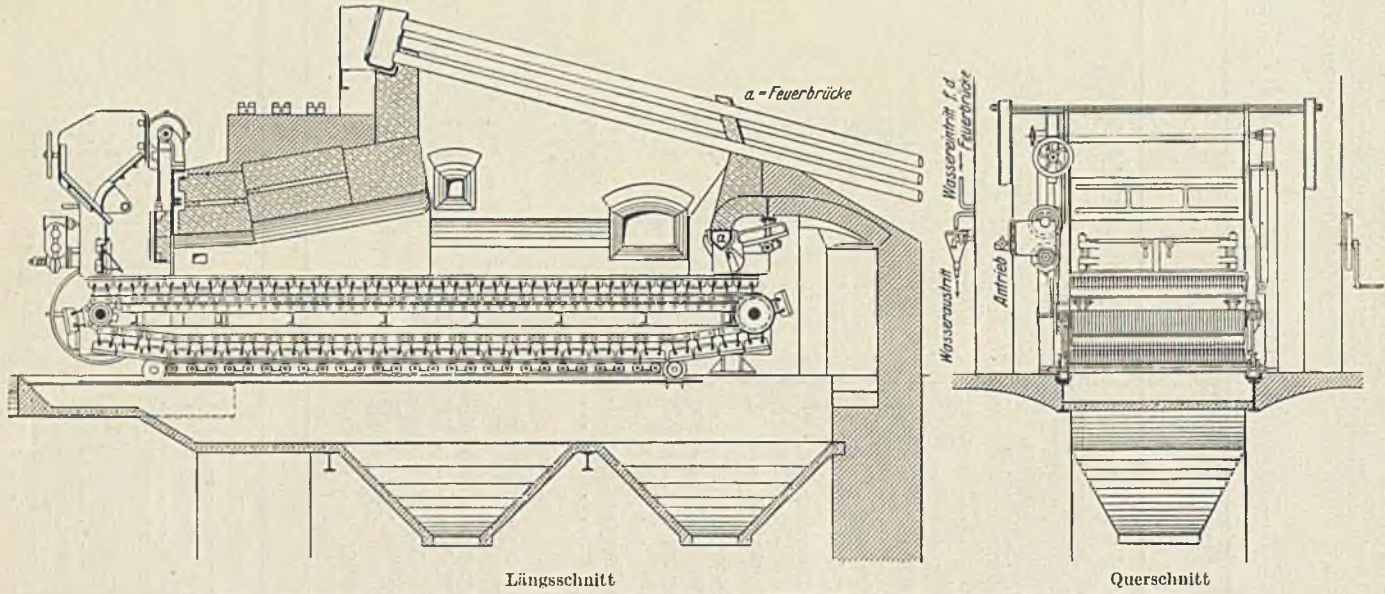
Längsschnitt Querschnitt Abb. 147. Einfacher Wanderplanrost mit Antrieb und wassergekühlter Feuerbrücke (Bauart L. & C. Steinmüller).
