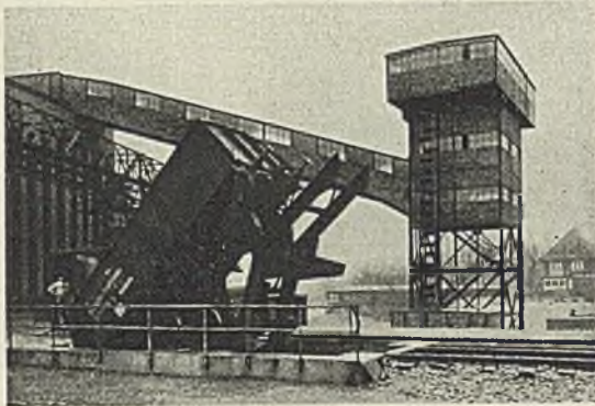
Abb. 239. Wagenkipper, Becherwerk, Übernahmeturm und Gurtförderer.
