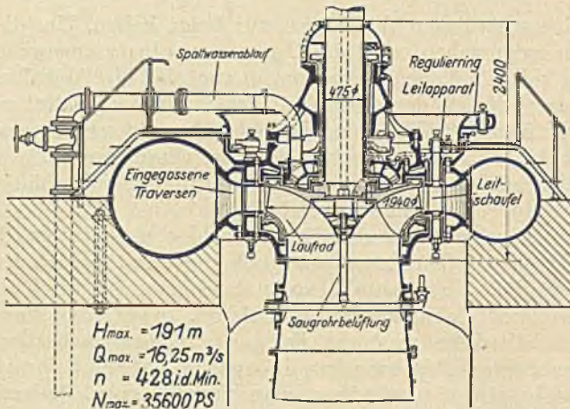
Abb. 330. Axialschnitt durch eine Voith-Spiralturbine mit stehender Welle.
