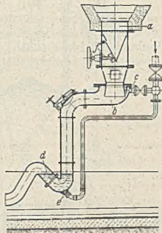
Abb. 192. Abzugsgerät für die Rothstein-Spülwasserentschung (D.R.P.). a Ascheinfall, b Stützfläche, c Wasserzutritt, d Syphon, e Ausstoßdüse. f Zulaufregler.
