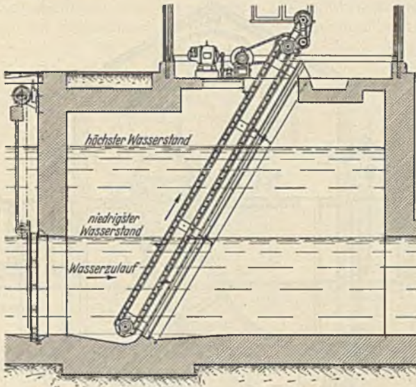
Abb. 73. Schlitzrechen mit Reinigungseinrichtung und elektromotorischem Antrieb (Bauart Gelger).
