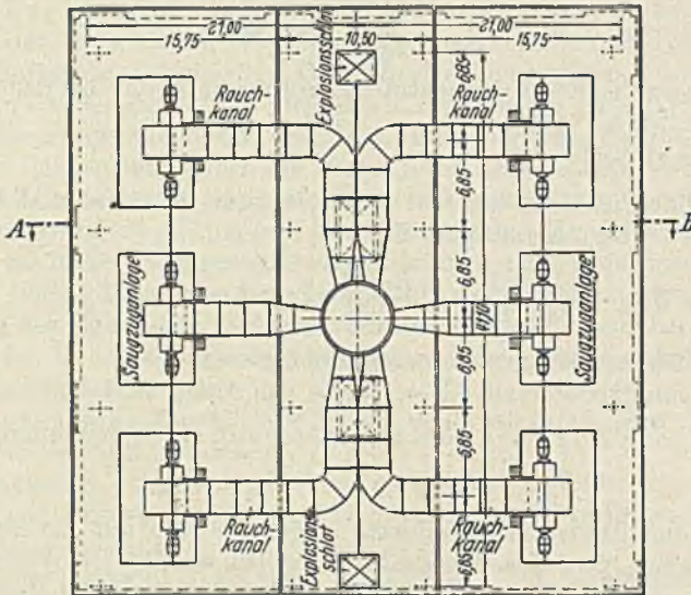
Abb. 185 a. Dachaufsicht.
