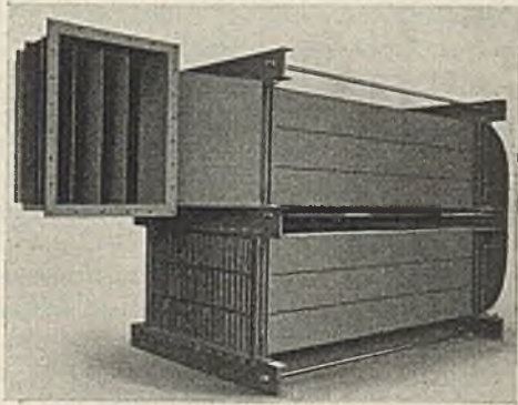
Abb. 178. Luftvorwärmer (Bauart L. & C. Steinmüller).
