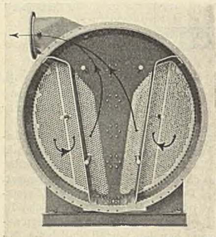
Abb. 69. Wasserkammeraustrittsseite.
