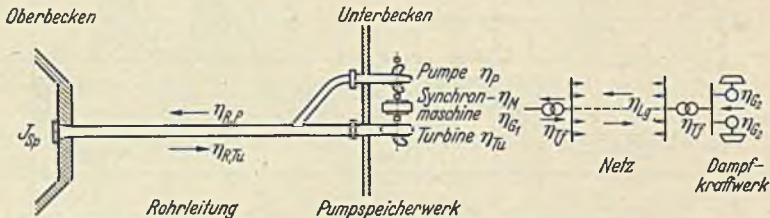
Abb. 362a. Übertragungsverhältnisse für eine Pumpspeicheranlage.
