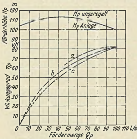
Abb. 374. Wirkungsgradverlauf für verschiedene Regelungsarten. a Drehzahlregelung, b Drehschaufelregelung, c Drosselregelung.
