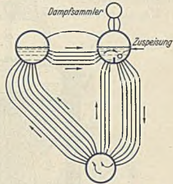
Abb. 126. Richtige Lage der Fallrohre.
