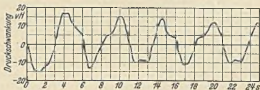
Abb. 372. Abschalten einer Speicherpumpe durch Trennen der Kupplung.
