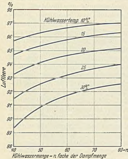
Abb. 70. Kühlwassertemperatur, Kühlwassermenge und erzielbare Luftleere im Oberflächenkondensator.
