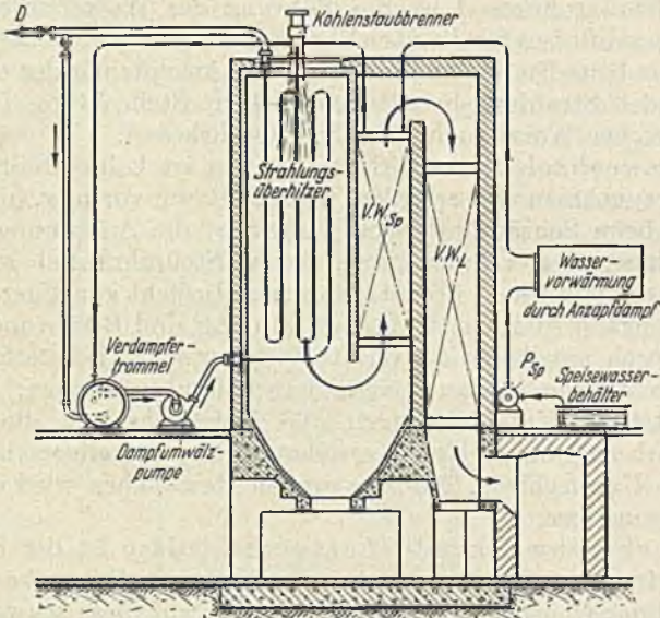
Abb. 130. Aufbau, Wasser- und Dampf-bewegung beim MAN-Löfflerkessel mit Kohlenstaubfeuerung ( P_{Sp} Speisepumpe).
