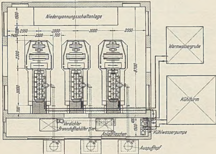
Abb. 285. Dieselmotorenkraftwerk mit 3 Fünfzylinder-Viertaktmotoren je 220 Psc, n = 500 U/min. Motorgewicht 9000 kg ohne und 14000 kg mit Zubehör und Schwungrad, Brennstoff: Südamerikanisches Dieselöl; Zylinderdurchmesser 250 mm, Kolbenhub 350 mm. Aufstellung 550 m über Meereshöhe, 45° C Tagestemperatur.
