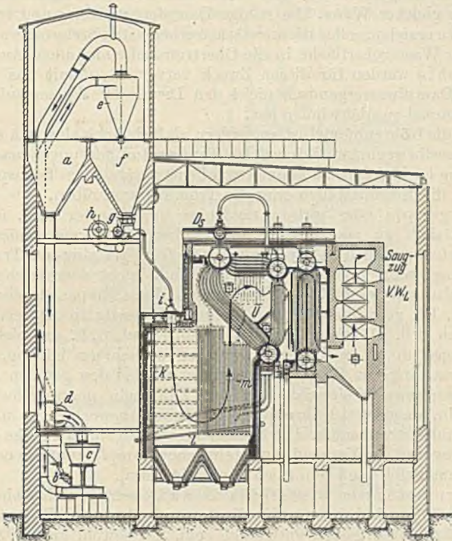
Abb. 131. Fünftrommelteilrohrkessel mit Kohlenstaubfeuerung, Bauart Lopulco, Mahlanlage, Wasserrohrrost, Strahlungsheizflächen, Überhitzer und Luftvorwärmer (Saugzuganschluß).
