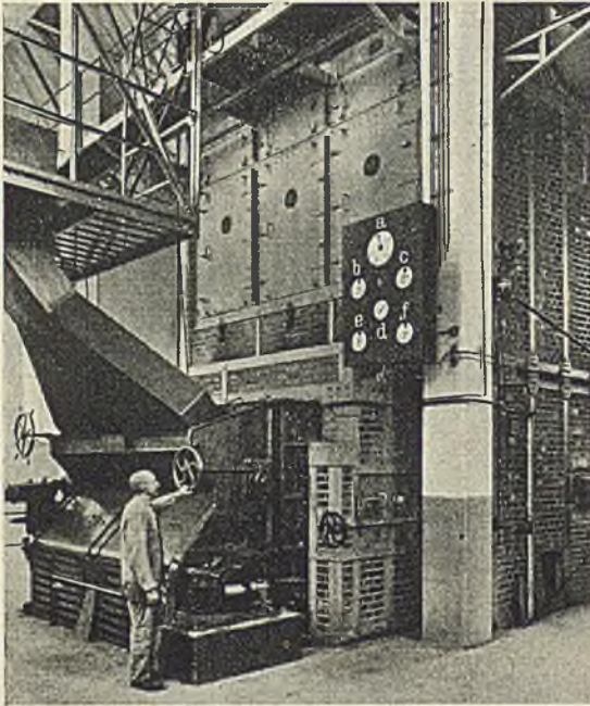
Abb. 221. Kesselschilder mit Rundmeßgeräten für einen Wanderrostkessel.
