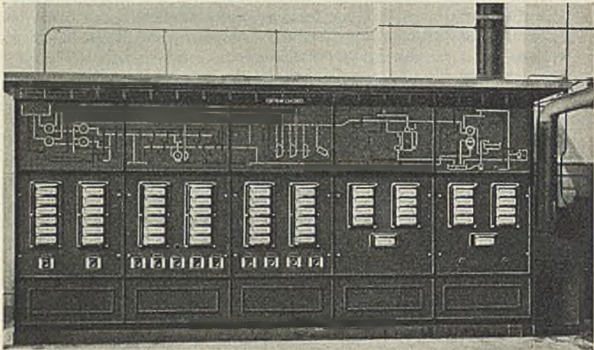
Abb. 224a. Wärmewarte mit Leuchtschaltbild im Pumpenraum eines Kraftwerkes.
