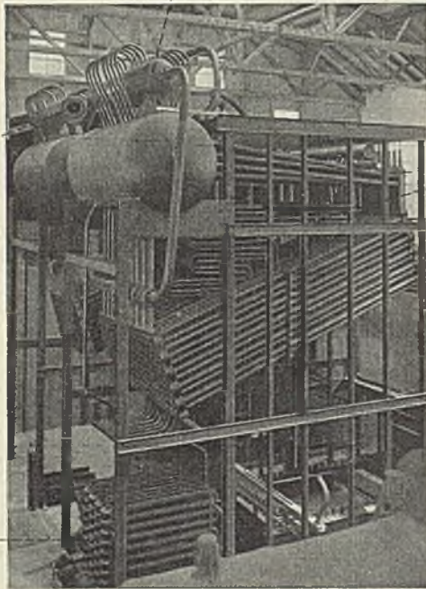
Abb. 137. Borsig-Telkammerschräghrohrkessel mit zwei querliegenden Obertrommeln hinten, Überhitzer und Rippenrohrspeisewasservorwärmer im Eisengerüst fertig zusammengebaut zur Einmauerung bereit.
