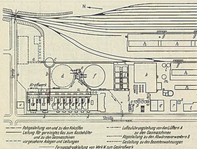
Abb. 301. Lageplan eines Gasmaschinenkraftwerkes mit Hilfsanlagen.
