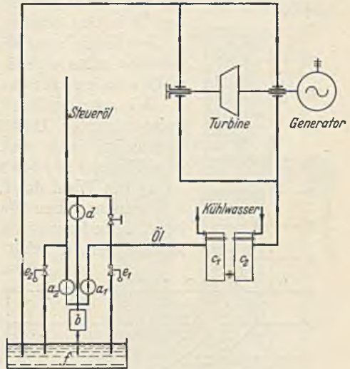
Abb. 46. Ölumlaufschmierung.
