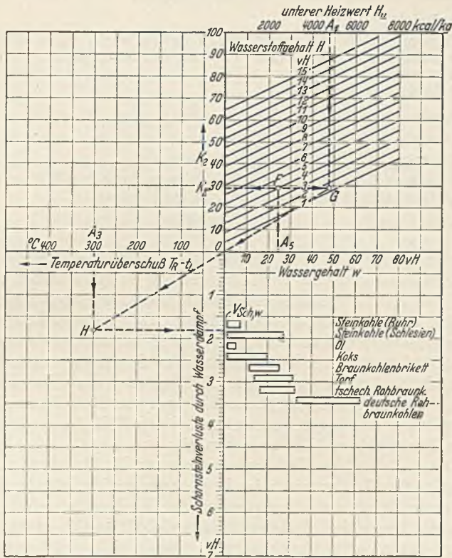
Abb. 95. Schornsteinverluste durch Wasserdampf.
