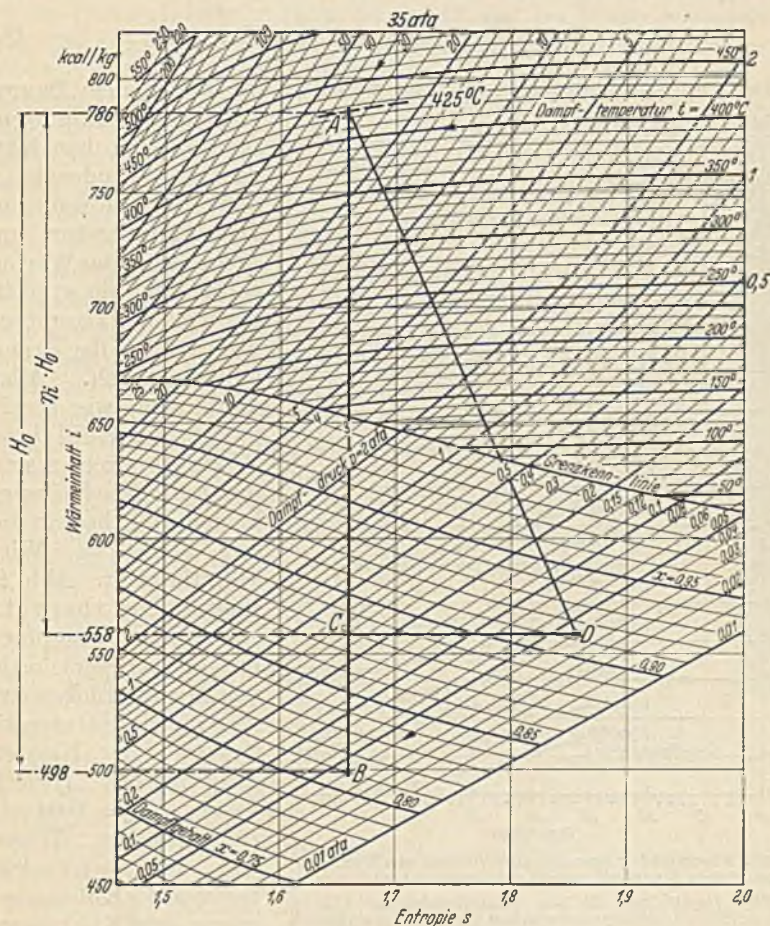
Abb. 26. JS-Diagramm für Wasserdampf (Mollier-Diagramm).
