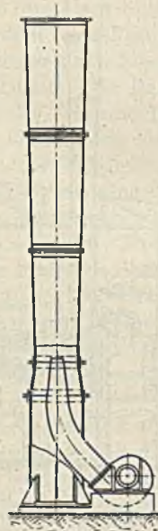
Abb. 189. Saugzuganlage (Bauart Schwabach) mit unmittelbarer und mittelbarer Luftregelung.
