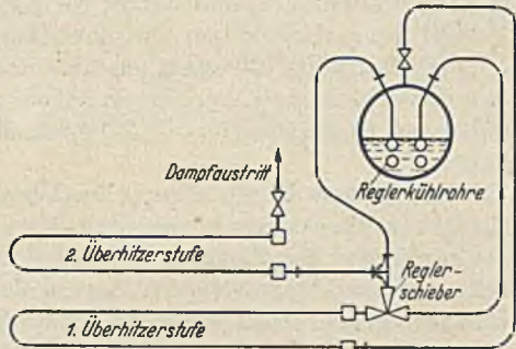
Abb. 171. Schaltbild der Babcock-Heißdampf-Temperaturregelung (D.R.P.).
