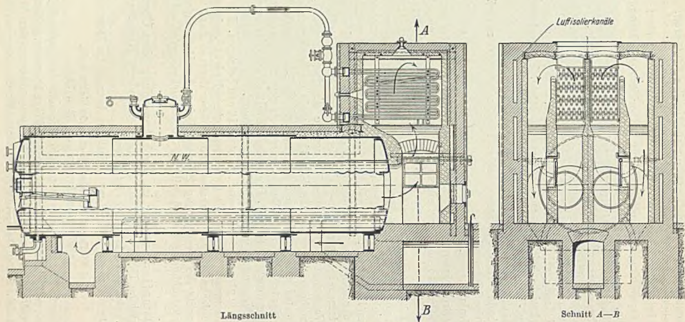
Abb. 113. Zweiflammrohrkessel (Wellrohrkessel) mit Planrostfeuerung und getrenntem Überhitzer.
