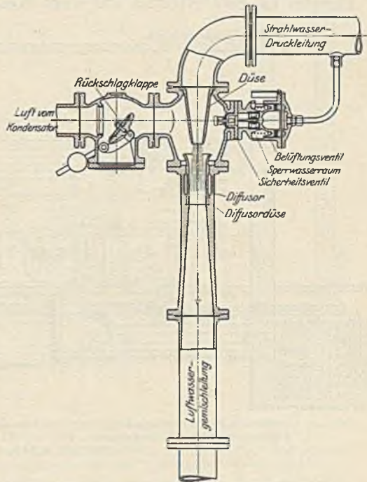
Abb. 78. MAN-Wasserstrahl-Luftpumpe.
