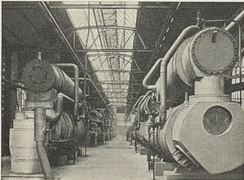
Abb. 307. MAN-Abwärmeverwerteranlage mit Abwärmekessel, Überhitzer und Speisewasservorwärmer, 14 ata, 350° C. 10 Gasmotoren.
