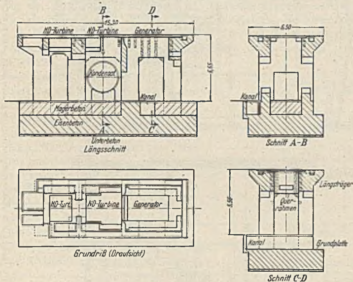
Abb. 61. Dampfturbinenfundament.
