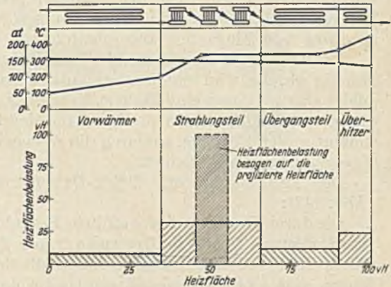
Abb. 141. S.S.W.-Bensonkessel, Druckverlauf, Temperaturverlauf und Heizflächenbelastung.
