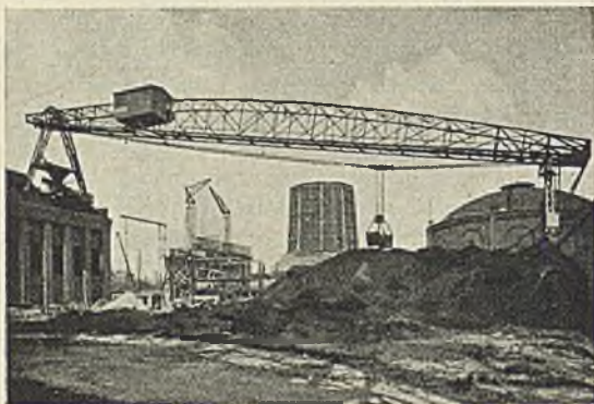
Abb. 234. Fahrbarer Brücken-Kabelkran zur Bedienung des Kohlenlagers und der Kohlenbunker eines Kraftwerkes (Spannweite 64 m, Tragkraft 5 t; Ausführung: Bleichert).
