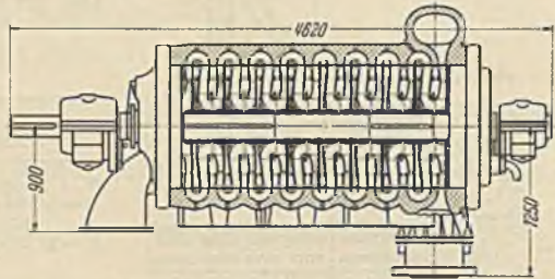
Abb. 363. Schnitt durch die Speicherpumpe des Tremorgio-Kraftwerks.
