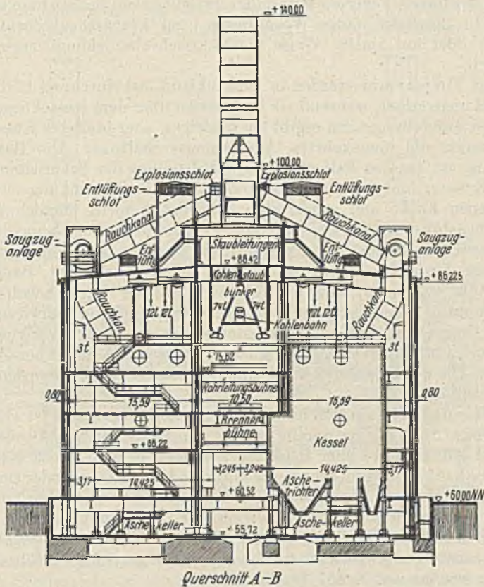
Abb. 186 b. Querschnitt.
