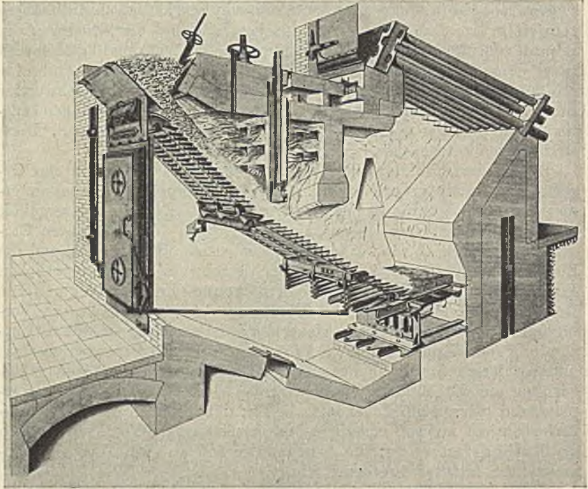
Abb. 157. Einfache Treppenrostfeuerung für Rohbraunkohle (Bauart Babcock).
