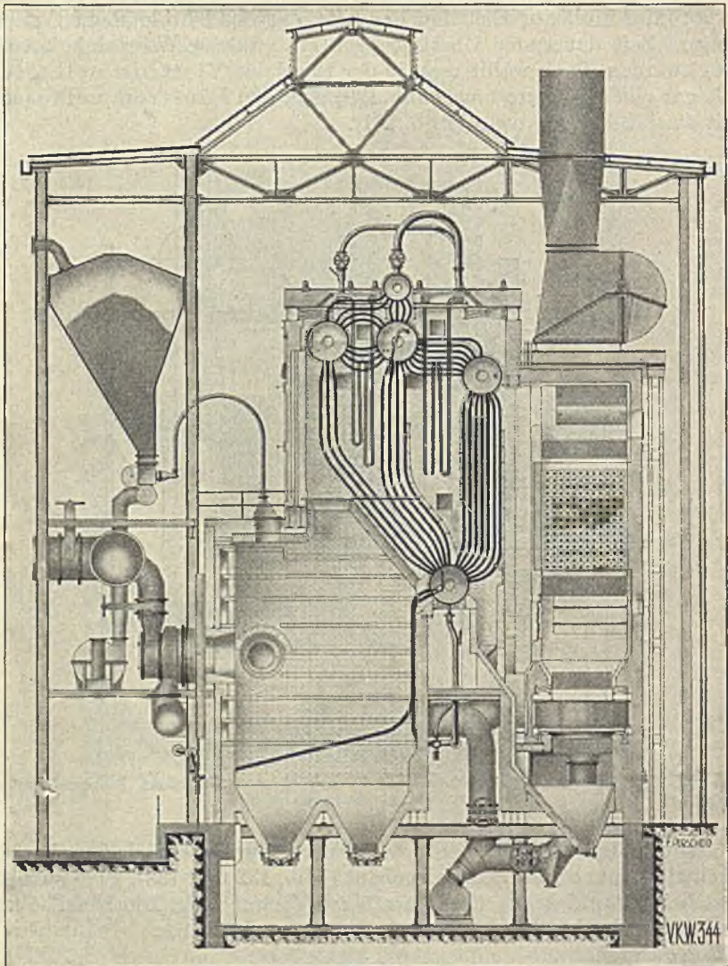
Abb. 130. Vereinigte Kesselwerke, Viertrommelstellrohrkessel mit einer Untertrummel, Kohlenstaubfeuerung, geteiltem Überhitzer und Rippenrohrspeisewasservorwärmer (Saugzuganschluß).
