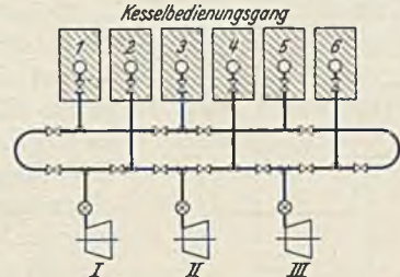
Abb. 196. Rohrleitungsplan, Ringsammelleitung.
