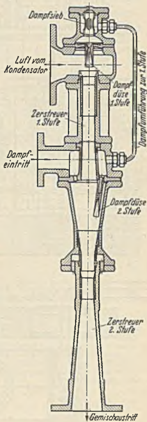
Abb. 82. Balcke-Dampfstrahlluftpumpe.
