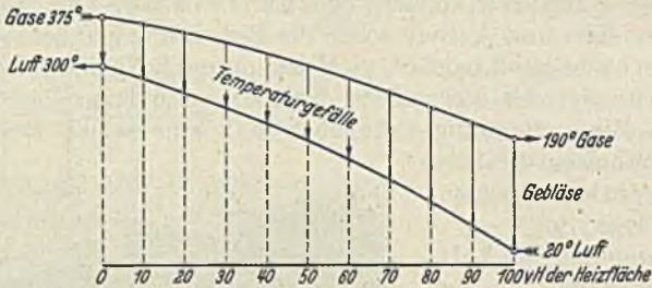
Abb. 170. Temperaturverlauf für die Abgasverwertung durch Luftvorwärmer.
