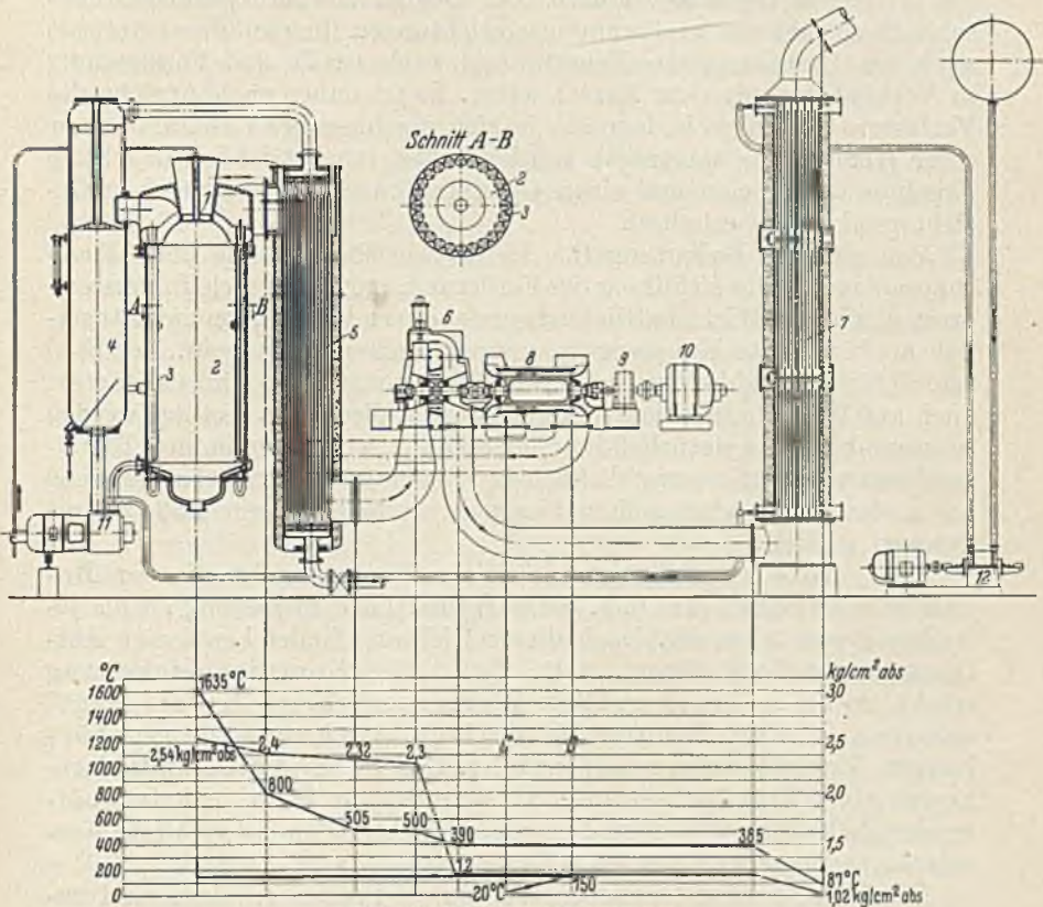
Abb. 142. BBC-Velox-Kesselanlage.
