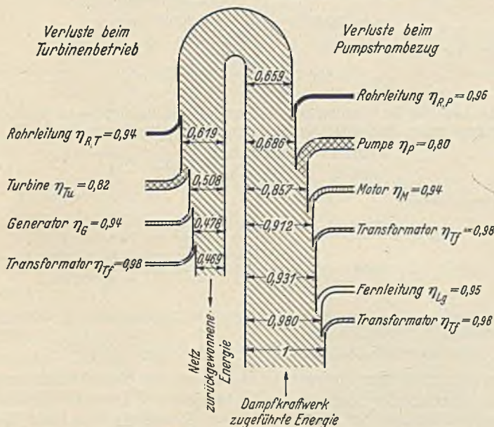
Abb. 362b. Energiestrombild für eine Pumpspeicheranlage.
