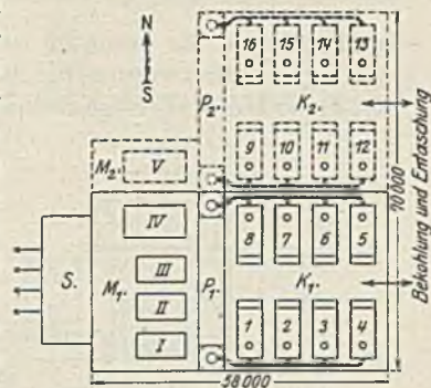
Abb. 256. Front bleibt bei Erweiterung von M und K nicht in Übereinstimmung. Bekohlung bei Erweiterung ungestört. Schornsteinplätze für Fuchsführung gut. Lage der Pumpenräume P_1 und P_2 , zwischen den Schornsteinen gut. Eingliederung der Frischdampfleitungen von K_2 nicht günstig. Explosionsausdehnung auf M durch Pumpenraum abgeschwächt, zwischen K_1 und K_2 durch Mittelmauer abgeschwächt, Explosionsausdehnung auf M durch Pumpenraum abgeschwächt, zwischen K_1 und K_2 durch Mittelmauer abgeschwächt.
