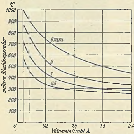
Abb. 102. Abhängigkeit der Blechtemperaturen von der Wärmeleitfähigkeit in \text{kcal/m}^2 \text{h}^\circ \text{C} und der Dicke des Kesselsteinbelages unter Zugrundelegung eines Wärmedurchganges von 15000 \text{kcal/m}^2 \text{h}^\circ \text{C} .
