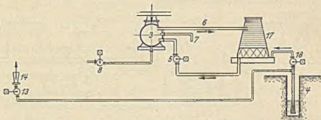
Abb. 20. Aufbau einer einfachen Dampfkraftanlage mit Kondensationsturbine für Kühlwasserrückkühlung (Ergänzung zu Abb. 19).
