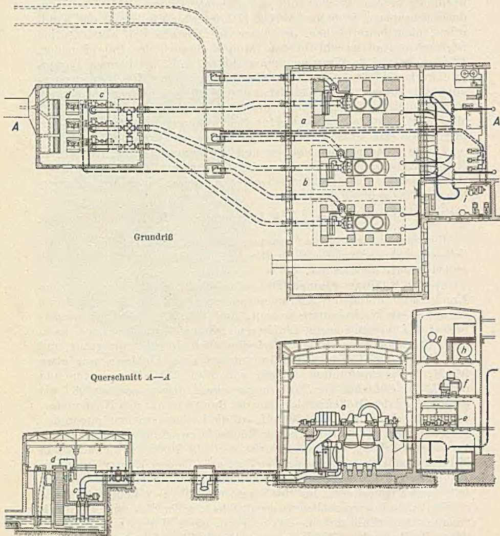
Abb. 77. Kraftwerk Schulau: Kühlwasserzu- und -ableitung, Maschinen und Rohrleitungen (AEG). a = 28000 kW-Turbine, b = 17000 kW-Turbine, c = Kühlwasserpumpen, d = Siebbänder, e = Kesselspeispumpen, f = Verdampfer, g = Warmspeicher, h = Kaltspeicher, i = Notturbine.
