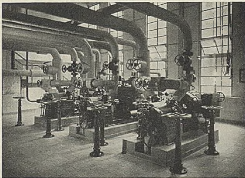
Abb. 213. Pumpenraum eines Kraftwerks mit 2 Turbo- und 1 Elektropumpe.
