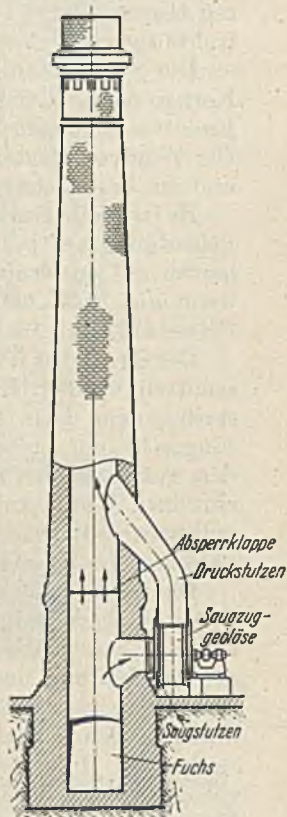
Abb. 190. Zusammengesetzte Zugsanlage (Schornstein- und Saugzug).
