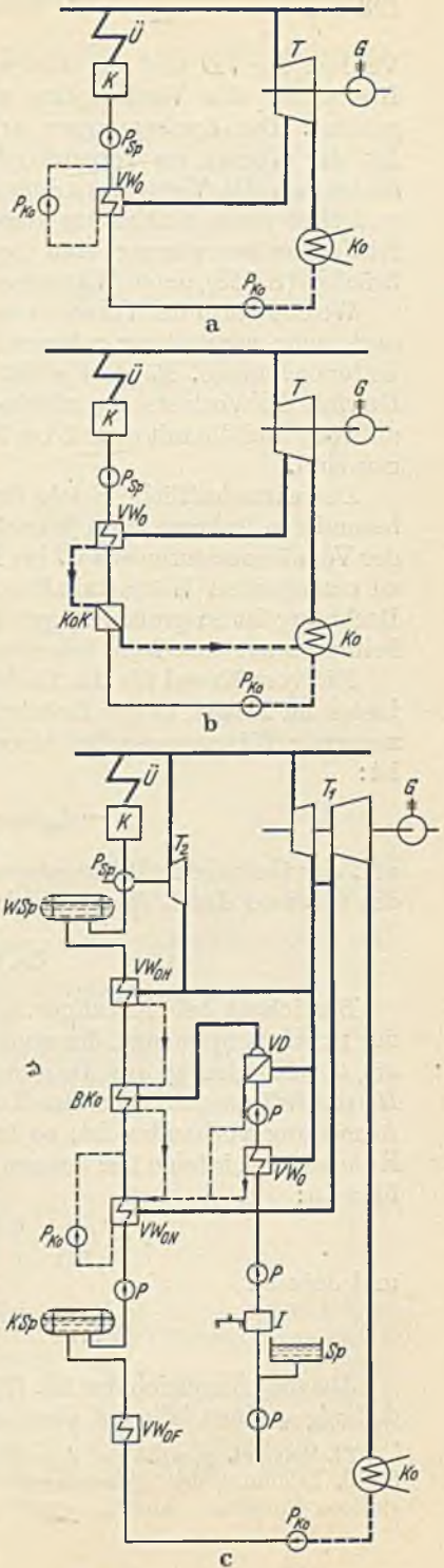
Abb. 111a bis c. Speisewasservorwärmung durch Anzapfdampf mit Oberflächenvorwärmer. a einstufig, b einstufig mit Kondensatkühler, c zweistufig mit Vorwärm- und Verdampferanlage für das Zusatzwasser.
