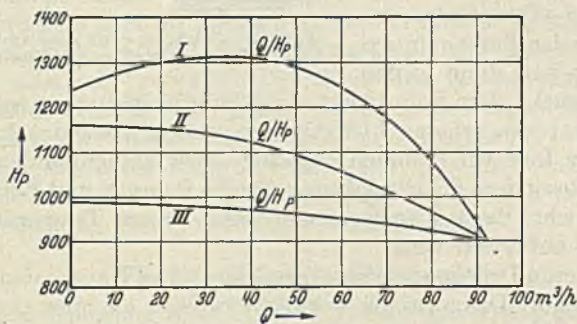
Abb. 208. Verlauf der QH_p -Linien von Kesselspeispumpen bei gleichbleibender Drehzahl. I unstetiger (labiler) Verlauf, II u. III stetiger (stabiler) Verlauf.
