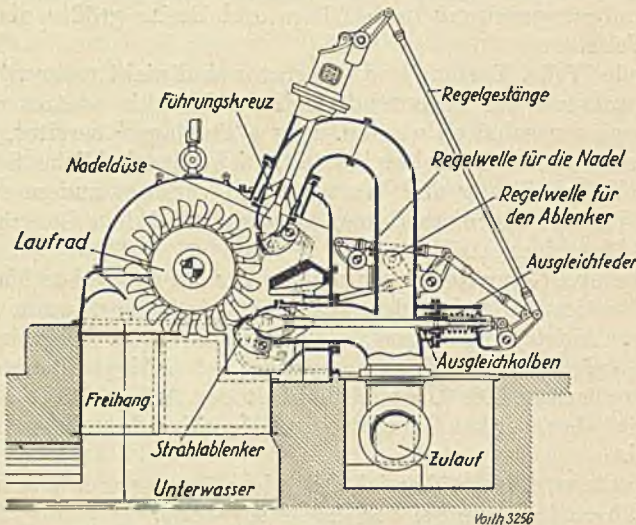
Abb. 325. Zweidüsige Voith-Freistrahlturbine mit Doppelregelung.
