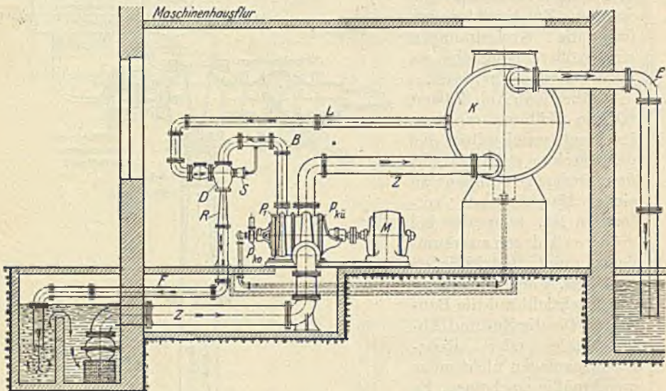
Abb. 79. Oberflächen-Kondensationsanlage für Frischwasserbetrieb mit elektrisch angetriebener Kühlwasser- und Kondensatpumpe und mit Wasserstrahl-Luftpumpe. MAN. (Erläuterungen s. Abb. 80.)
