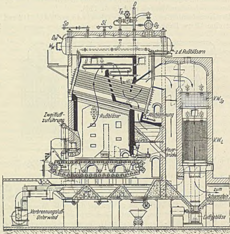
Abb. 115. Babcock-Tellkammerkessel mit längslegender Obertrommel, 350 m 2 Heizfläche, 33 atü, mit Unterwind-Zonenwandlerrost, Zweitluftzuführung, Überhitzer, Rippenrohr-Speisewasservorwärmer und Luftvorwärmer (Schornsteinanschluß).
