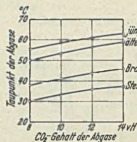
Abb. 176. Taupunkt der Abgase (Rauchgase) verschiedener Brennstoffe in Abhängigkeit vom CO 2 -Gehalt (85 vH Feuchtigkeit der Brennluft bei 15° C).
