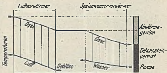
Abb. 172. Allgemeiner Temperaturverlauf für die Abgasverwertung durch Luft- und Speisewasservorwärmer.
