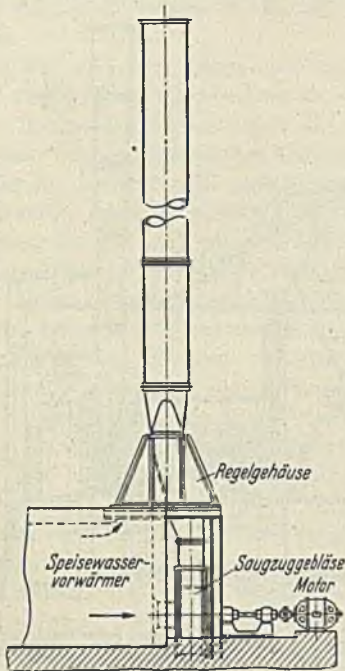
Abb. 188. Saugzuganlage mit unmittelbarer Luftbewegung.
