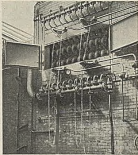
Abb. 175. Speisewasservorwärmer betriebsfertig eingebaut, Türen geöffnet (L. & C. Steinhüller).
