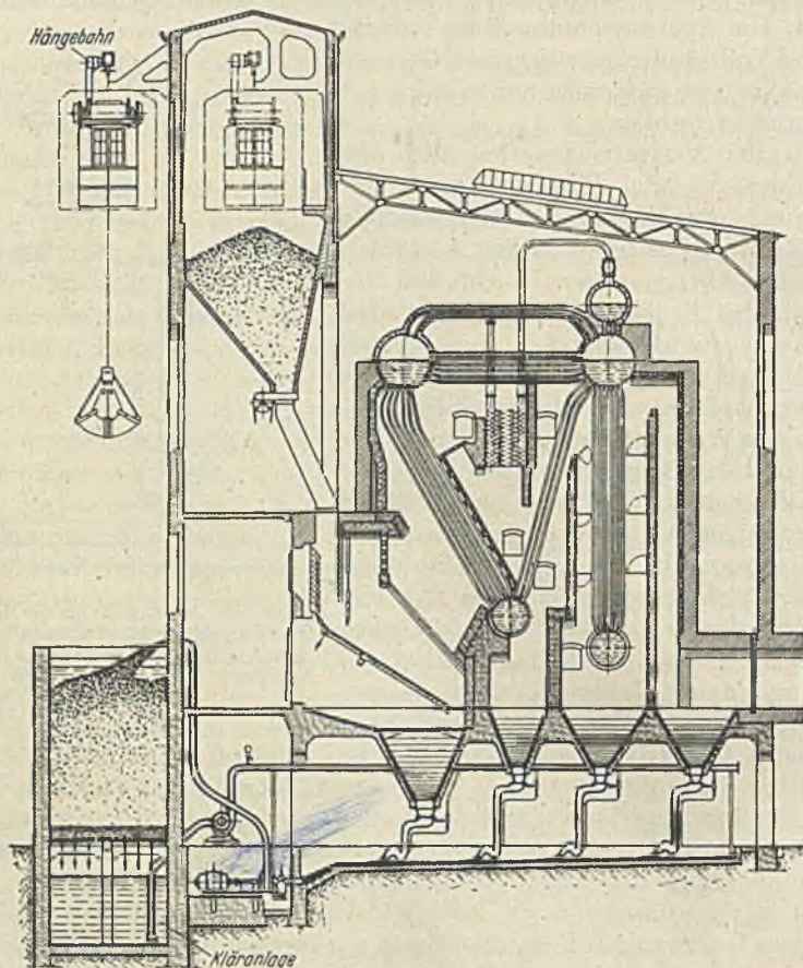
Abb. 193. Kesselanlage mit Rothstein-Spülwasserentschung, Kläranlage und Ascheentfernung.
