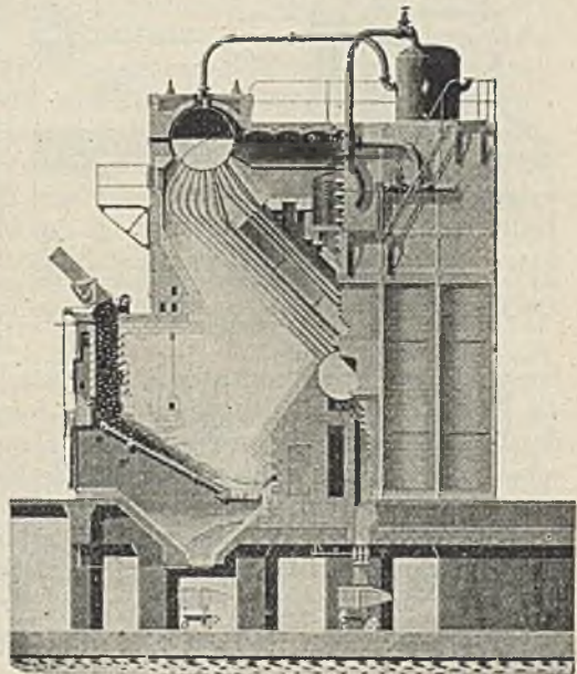
Abb. 182. Topsche Bogenform-Einmauerung eines Stellrohrkessels mit Überhitzer für Rohbraunkohlenfeuerung.
