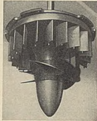
Abb. 337. Kaplanturbine, Leitapparat und Laufrad offen.
