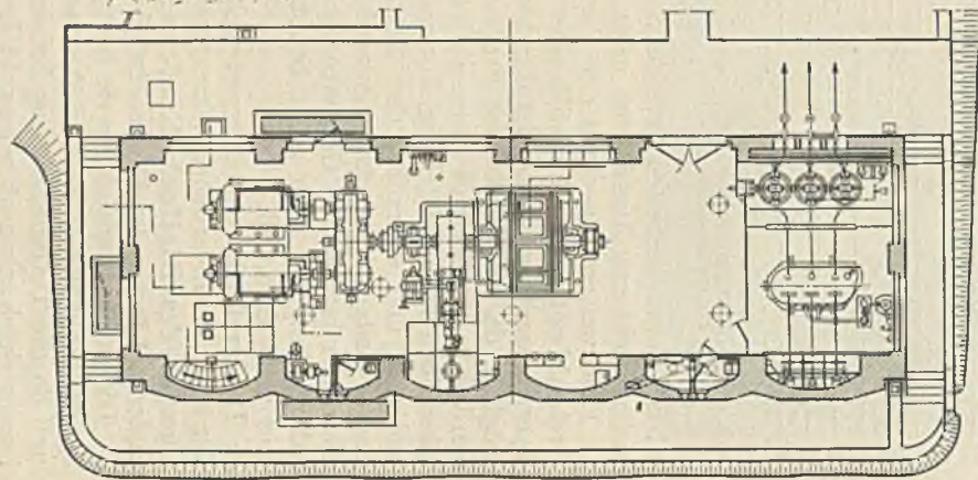
Abb. 377. Kraftwerk Tremorglo, Hochdruck-Pumpspeicherwerk.
