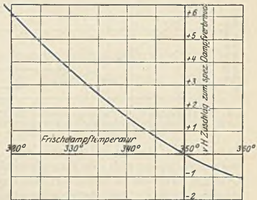
Abb. 55. Abhängigkeit des Dampfverbrauches für Abb. 54 von der Frischdampftemperatur.
