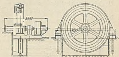
Abb. 280. Generator mit eingebautem GD^2 .
