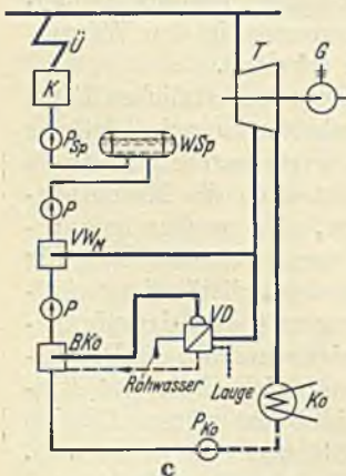
Abb. 110a bis c. Speisewasservorwärmung durch Anzapfdampf mit Mischvorwärmer. a einstufig, b zweistufig, c einstufig mit Verdampferanlage für das Zusatzwasser.
