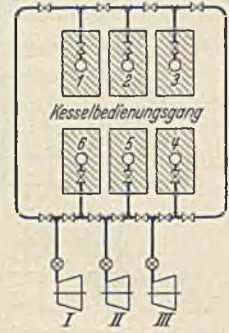
Abb. 199. Ringsammelleitung, Kessel gegenüber.
