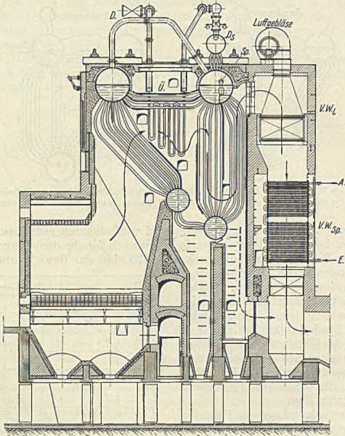
Abb. 128. Borsig-Viertrommelsteilrohrkessel mit Unterschubfeuerung, Überhitzer, Rippenrohrspewasservorwärmer und Luftvorwärmer (Schornsteinanschluß).
