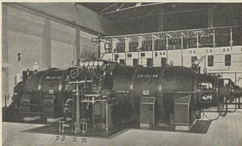
Abb. 64. Bedienungssseite einer 7700 kW MAN-Gegenlauf-Gegendruckturbine (Ljungströmturbine) n = 3000 U/min, 14 ata, 325° C, 3,5 ata Gegendruck.
