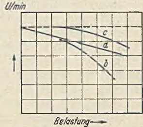
Abb. 282. Drehzahlkennlinie für Belastungsänderungen bei Kolbenkraftmaschinen.
