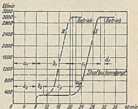
Abb. 63. Anwärms- und Anfahrvorschrift für Regel- und Schnellfahrmaschinen.
