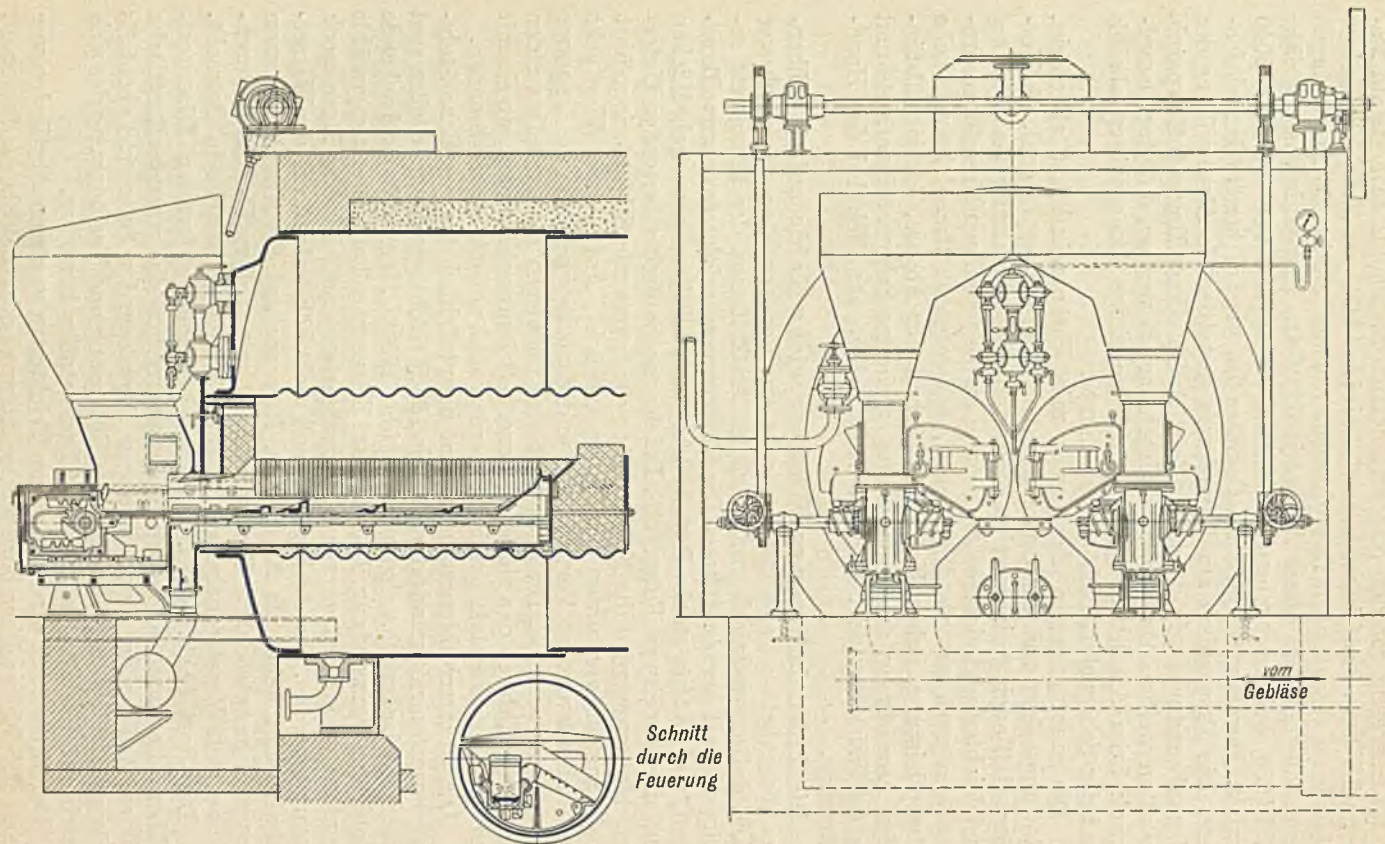
Abb. 144. Zweiflammrohrkessel mit Unterschubfeuerung und Unterwind.
