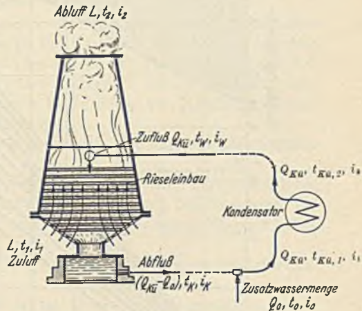
Abb. 90. Kühlverlauf beim Gegenstrom-Kammlukühler.
