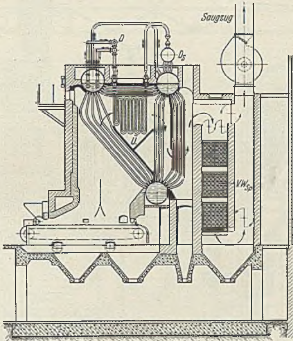
Abb 129. MAN-Dreitrommelstahlrohrkessel mit Zonenwanderrost. Überhitzer, Rippenrohrspeisewasservorwärmer (Saugzuganschluß).
