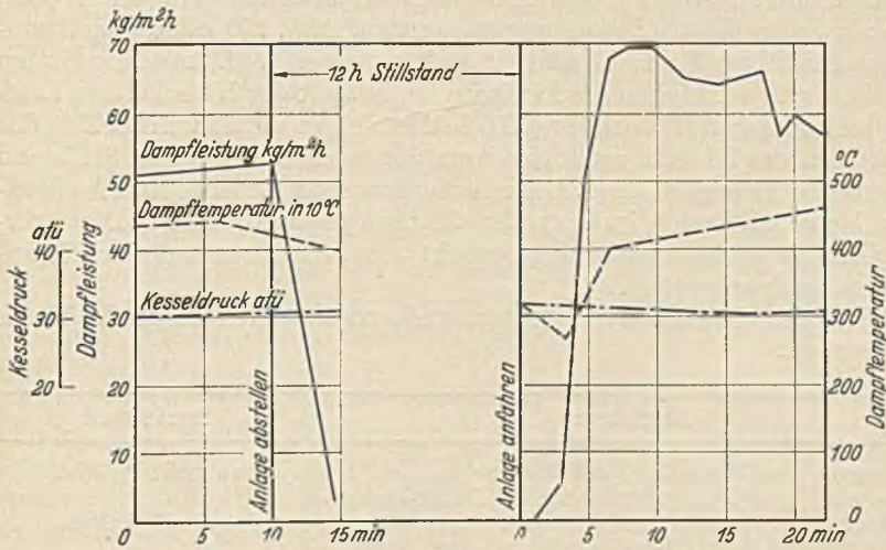
Abb. 150. Betriebskennlinien für einen Babcock-Schrägröhrokessel mit Unterwind-Zonenwanderrost (Brennstoff: Anthrazit-Mittelprodukt).
