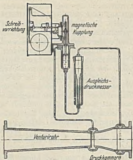
Abb. 227. Venturimeter mit Schreibvorrichtung.
