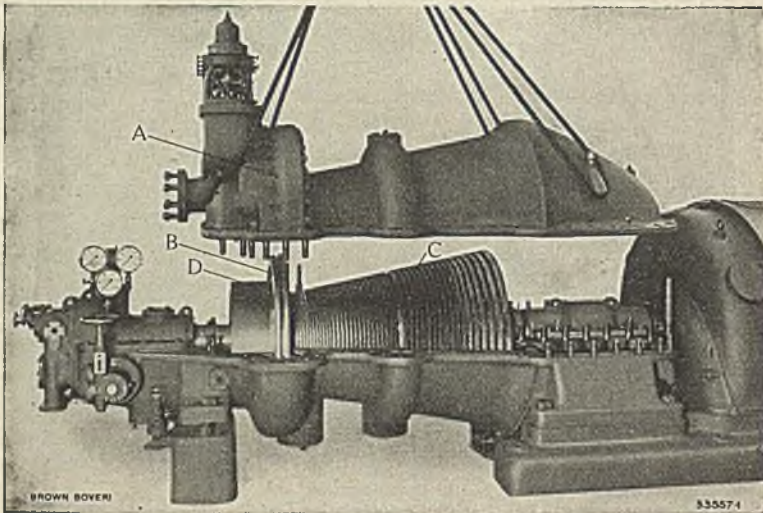
Abb. 65. 10000 kW-Einzylinder-Kondensationsturbine, Drehzahl 3000 U/min. Gehäuseoberteil abgehoben.
