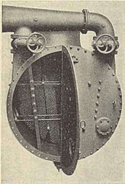
Abb. 76. Geteilter Kondensator als Dauerbetriebskondensator (Bauart BBC).
