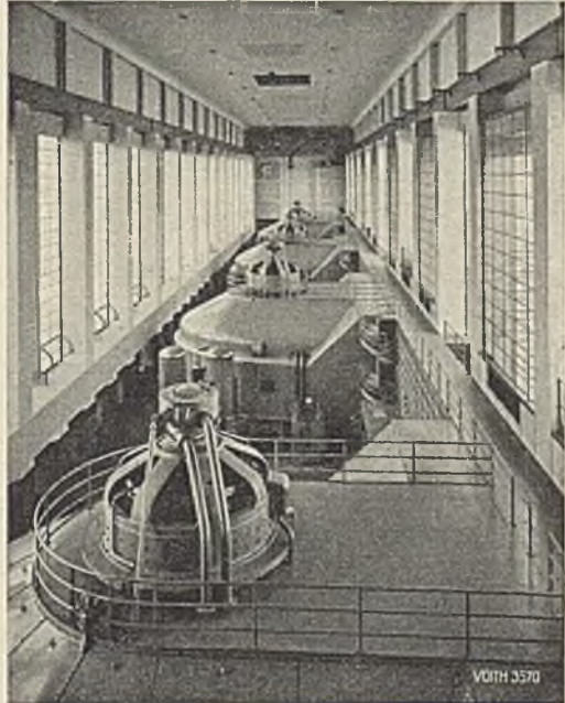
Abb. 360. Blick in den Maschinenraum des Rheinkraftwerkes Ryburg-Schwörstadt.
