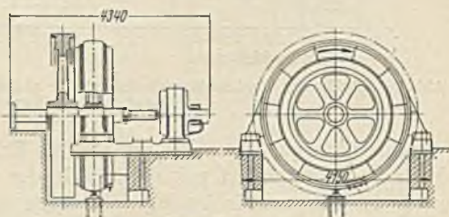
Abb. 279. Generator mit Schwungrad.
