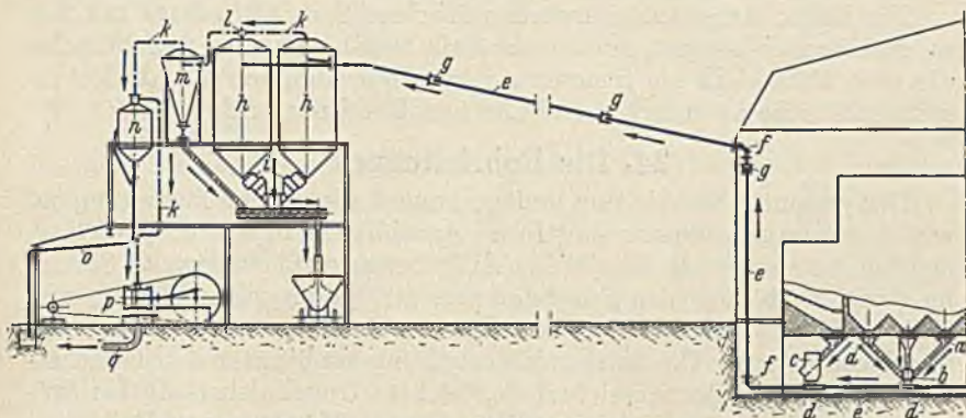
Abb. 194. Saugluftentäsungsanlage (Bauart Hartmann A.G., Offenbach a. Main).
