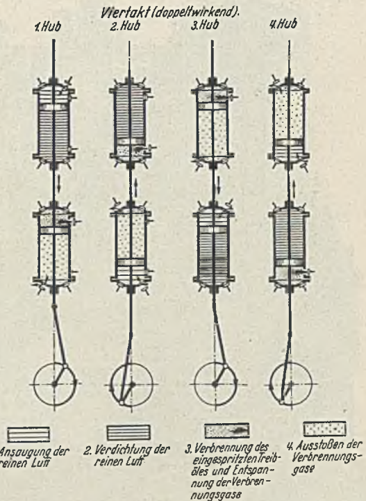
Abb. 269. Arbeitsverlauf beim doppeltwirkenden Viertakt-Dieselmotor.
