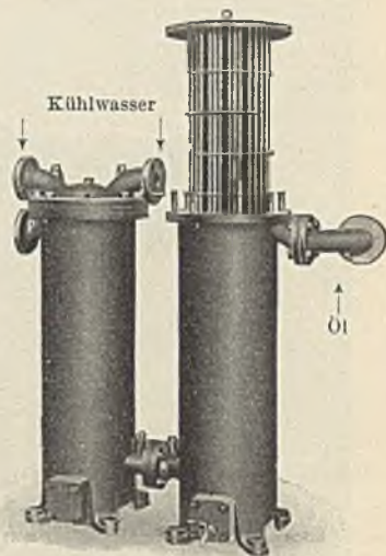
Abb. 48. Ölkühler (teilweise herausgezogene Kühlschlangen).
