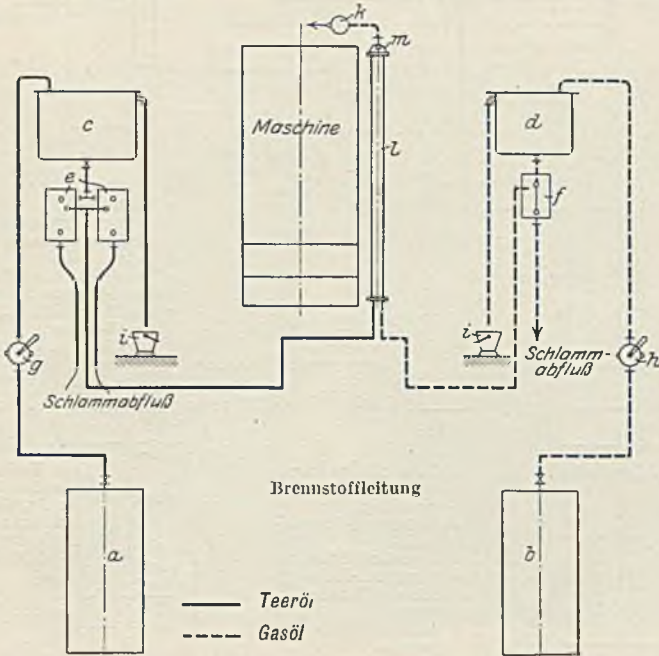
Abb. 287 b. a Teeröl-Lagerbehälter, b Gasöl-Lagerbehälter, c Teeröl-Betriebsbehälter, d Gasöl-Betriebsbehälter, e Teeröl-Filter, f Gasöl-Filter, g Teeröl-Handpumpe, h Gasöl-Handpumpe, i Eimer, k Schwimmertopf, l Vorwärrohr nur bei dickflüssigen Brennstoffen, m Umschalhahn.
