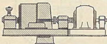
Abb. 43. Dreilagerausführung.
