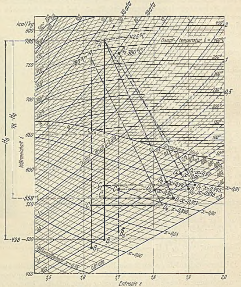
Abb. 29. Einfluß von Dampfspannung, Dampftemperatur und Kondensatorluftlere auf die Dampfeuchtigkeit am Turbinenende.
