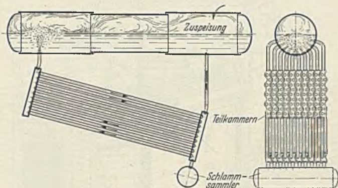
Abb. 114. Teilkammer-Schrägrohrkessel mit längs liegender Obertrommel; Aufbau, Wasser- und Dampf bewegung.
