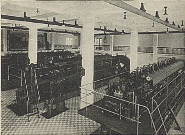
Abb. 288. Kraftwerk mit 3 Zehnzylinder-MAN-Dieselmotoren von je 1780 PS, (Elektrizitätsverband Gröbba).
