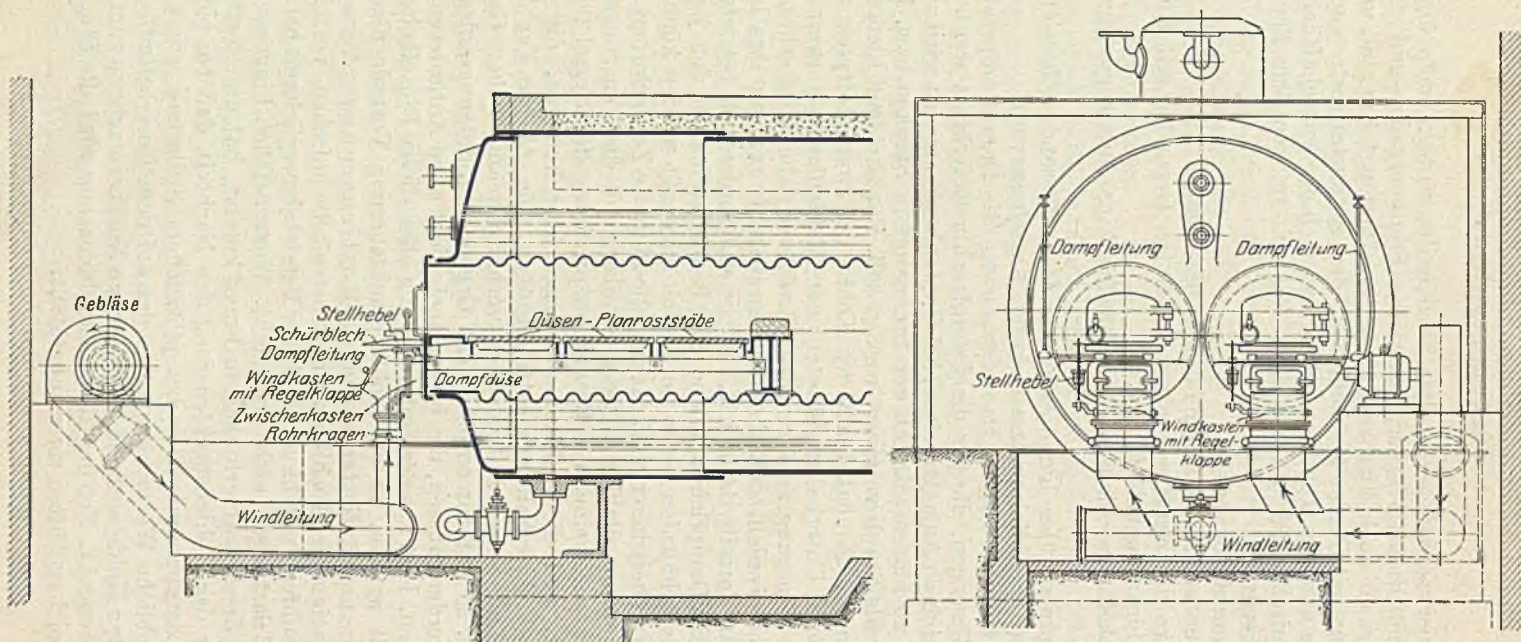
Abb. 143. Zweiflammrohrkessel mit Planrost, Unterwind und Dampfstrahlzusatz.
