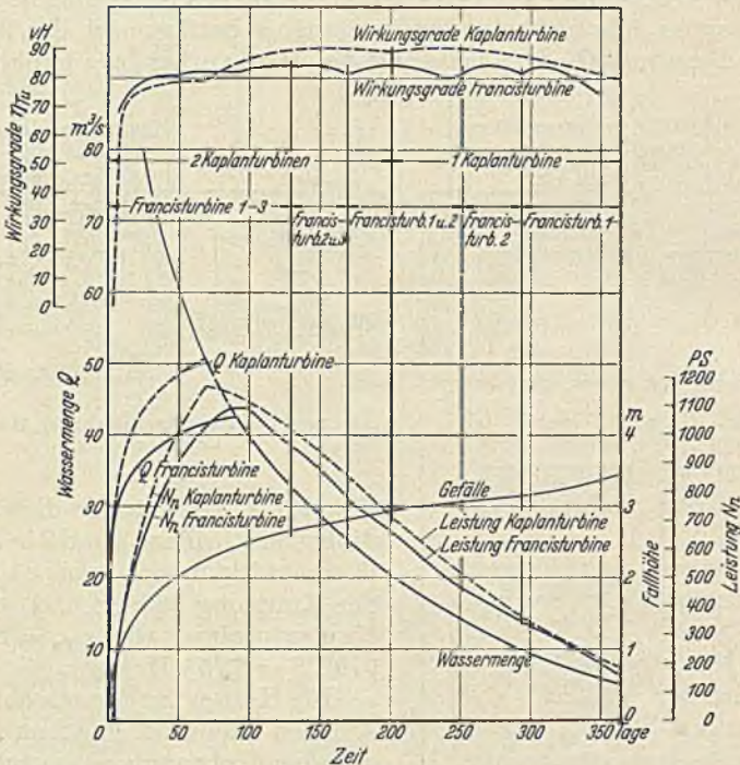
Abb. 343. Turbinenkennlinien für das Laufwasserkraftwerk nach Abb. 341 und 342 bei Francis- und Kaplanmaschinen.
