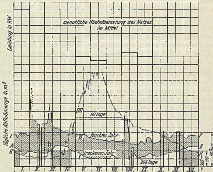
Abb. 308. Wassermengen-Jahresverlauf.
