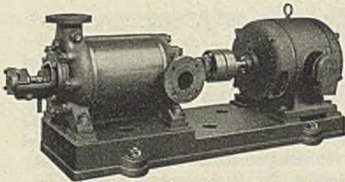
Abb. 211. Speisewasserpumpe mit Elektromotorantrieb.
