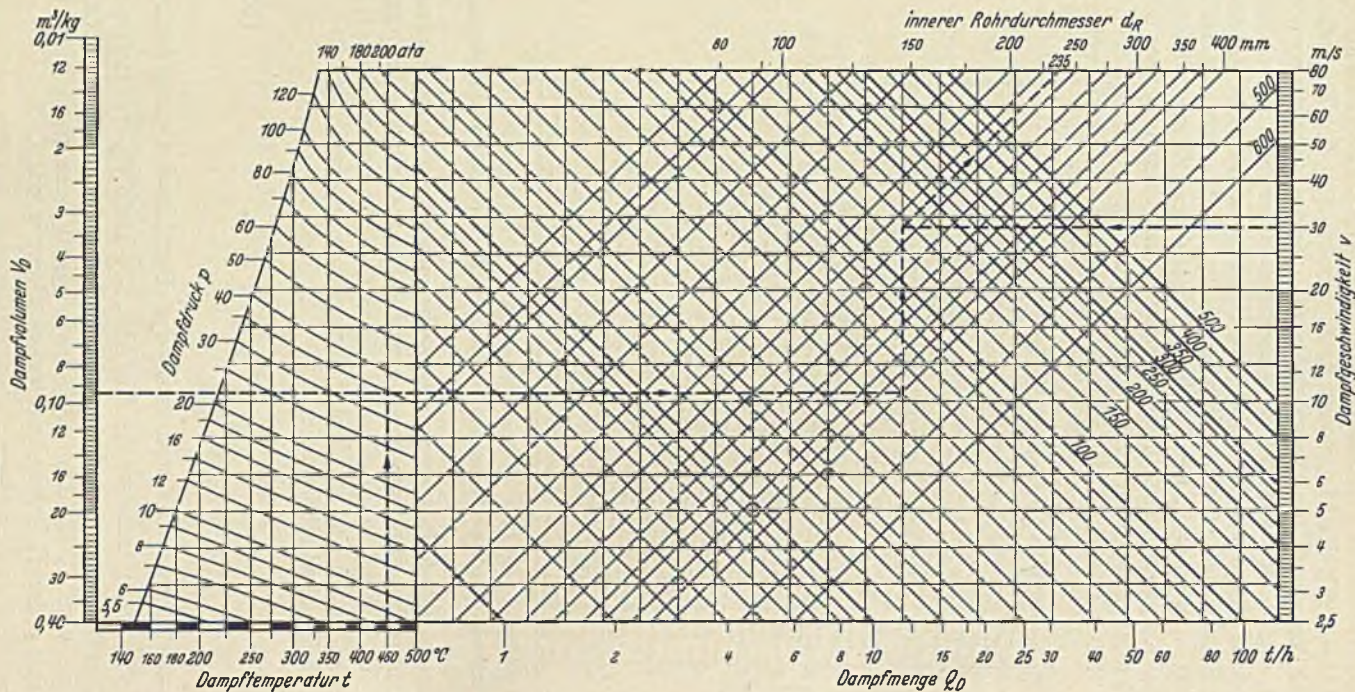
Abb. 204. Strömungsgeschwindigkeit in Dampfleitungen.
