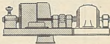
Abb. 44. Vierlagerausführung.
