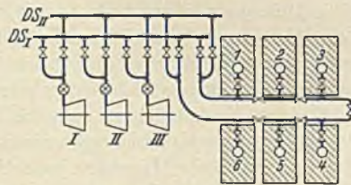
Abb. 201. Doppelsammelleitung.
