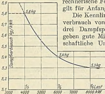
Abb. 54. Dampfverbrauch eines Drehstrom-Turbosatzes einschl. Kondensationsarbeit bei 13,5 m manometrischer Kühlwasser-Förderrhöhe, 11300 PS, 8000 kW, n = 3000 U/min, Frischdampf 14 ata, 350° C Überhitzung am Eintrittsstutzen, Kühlwassertemperatur 27° C.
