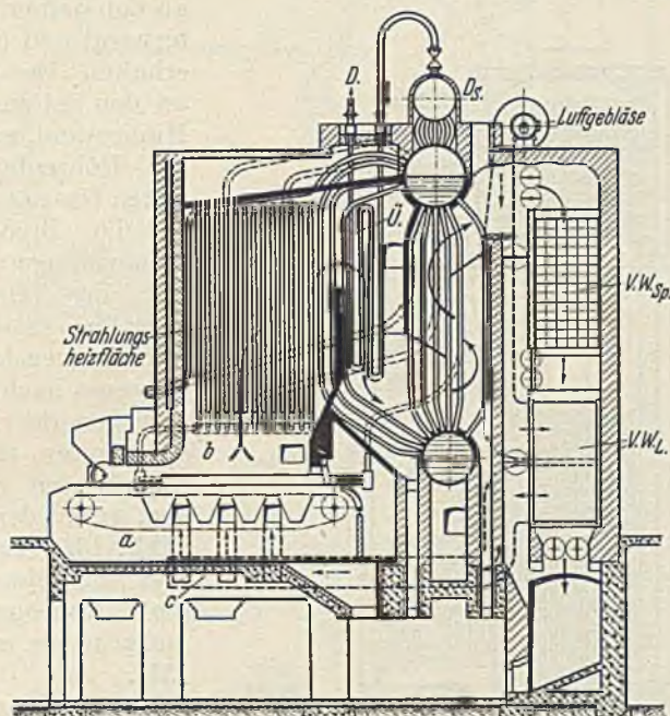
Abb. 132. MAN-Zweitrommelsteilröhrkessel mit Unterwind, Zonenwanderrost, Strahlungsheizflächen, Überhitzer, Rippenrohrspeisewasservorwärmer und Luftvorwärmer (Schornsteinschluß).
