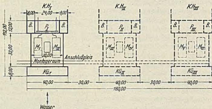
Abb. 258. Kraftwerksgrundriß. Aufgelöste Bauart.
