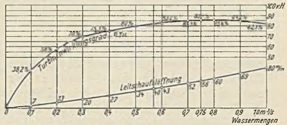
Abb. 323. Wirkungsgrad und Leitschaufelöffnungen einer Francisturbine für verschiedene Wassermengen.
