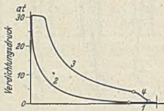
Abb. 267 u. 268. Arbeitsverlauf beim einfachwirkenden Zweitakt-Dieselmotor.
