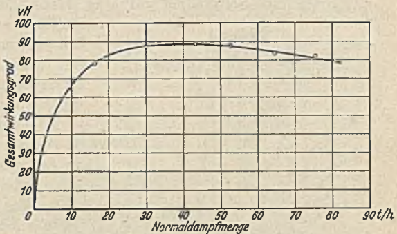
Abb. 161. Kesselwirkungsgrad bezogen auf die Normaldampfmenge in t/h bei einem Steinhüller-Großstelrohrkessel mit Doppelvorschub-Treppenrostfeuerung (Rohbraunkohle 51 bis 53 vH Wassergehalt, 6 bis 7 vH Asche, 40 vH Feingehalt, H_u = 2250 kcal/kg, 1350 m 2 Heizfläche, 40 atü 380^\circ C, 77,8 m 2 nutzbare Rostfläche).
