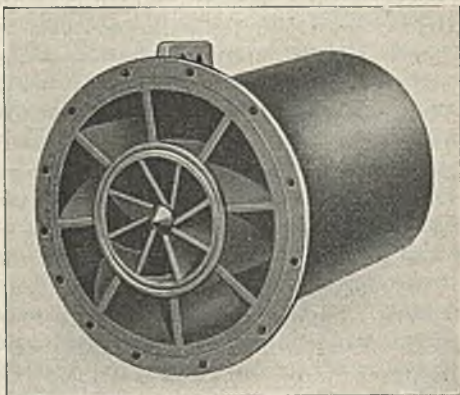
Abb. 165. Steinmüller-Wirbelbrenner.
