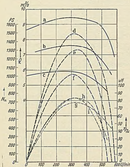
Abb. 322. Leistungs-, Wassermengen- und Wirkungsgradverlauf einer Francisturbine bei drei Leitschaukelöffnungen.
