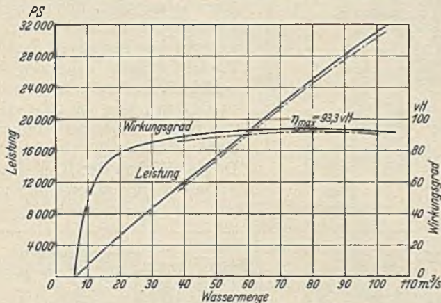
Abb. 340. Wirkungsgrad und Leistung der Shannon-Kaplan turbinen (Voith). H = 25,15 \text{ m} , n = 167 \text{ U}/\text{min} , - - - - - gewähltestet, ——— erreicht.
