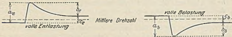
Abb. 347. Drehzahländerung für einen Entlastungs- und einen Belastungsvorgang mit Ungleichförmigkeit im Regler.
