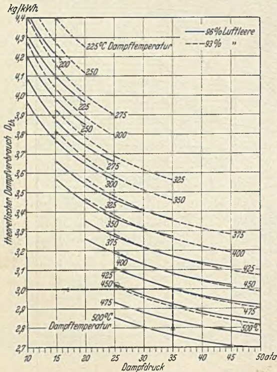
Abb. 27. Theoretischer spez. Dampfverbrauch von Kondensationsturbinen für 96 vH und 93 vH Kondensatorluftleere. Beispiel: Dampfdruck 35 ata, Dampftemperatur 425^\circ \text{C} , Luftleere 96 vH ergibt theoretischen spez. Dampfverbrauch D_{th} \cong 3,0 \text{ kg/kWh} .
