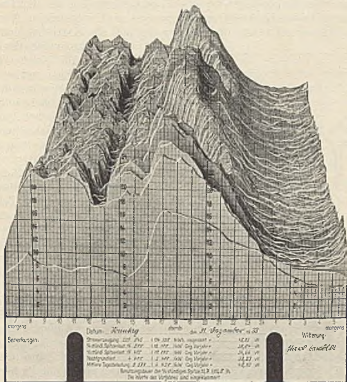
Abb. 13. Kartenaufzeichnungen der Tagesbelastungen in zwei Kalenderjahren (Darstellung der Belastungsgebiete).
