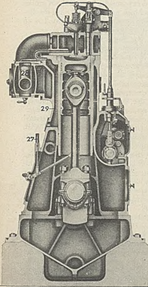
Abb. 271. Querschnitt durch einen kompressorlosen Krupp-Dieselmotor von 220 PS.
