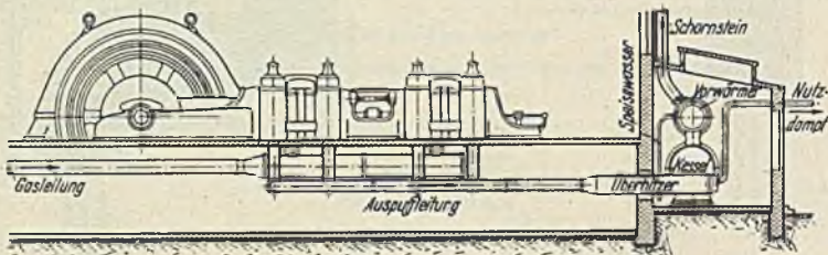
Abb. 305. Gasmachine mit Abwärmedampfkessel, Überhitzer und Speisewasservorwärmer.
