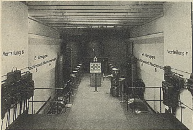
Abb. 358. Ansicht der Bedienungsbühne des Hilfsmaschinenraumes zu Abb. 357.
