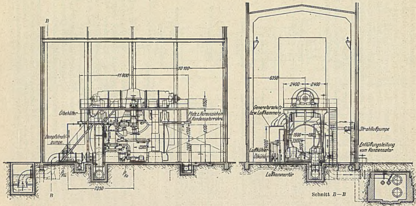
Abb. 62. Aufstellungs- und Rohrplan für eine 12000 kW MAN-Tjungström-Kondensationsturbine, 18 ata, 375° C, n = 3000 U/min.
