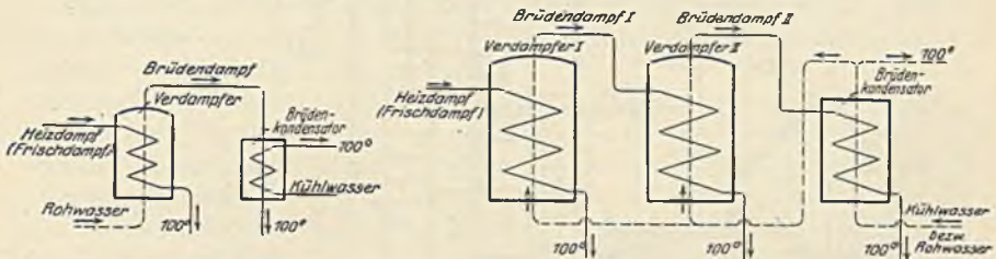
Destillat aus Heizdampf Brühdampf a Einfache Verdampferanlage
