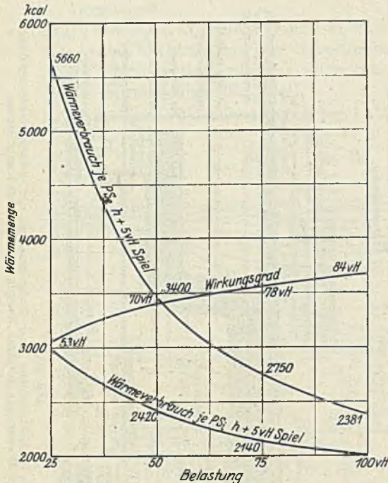
Abb. 304. Betriebskennlinien für eine Großgasmachine.
