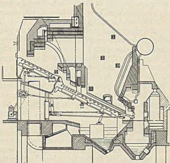
Abb. 158. Doppelvorschub-Treppenrostfeuerung für Rohbraunkohle (Bauart L. & C. Steinmüller).
