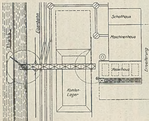
Abb. 233. Kohlenförderanlage für ein mittleres Kraftwerk (Schiff, Eisenbahn und Kohlenlager), Förderband- und Bunkerbeschickung vom Drehkran.
