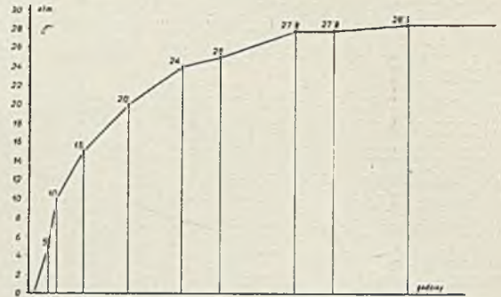
Rys. 8. Krzywa ciśnienia gazu przy pomiarze ciśnienia złoża na szybie „Władysław”.
