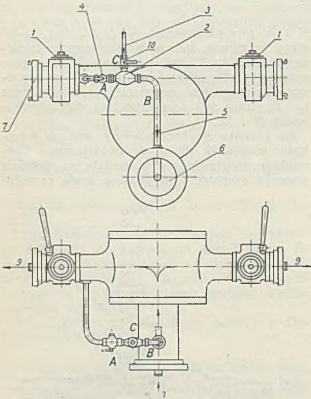
Rys. 10. Sposób wbudowania mieszalnika. 1. Zawór tłoczny. 2. Mieszalnik. 3. Dopływ „Pianolu“. 4. Kurek wodny. 5. Mieszanka pianolowo-wodna. 6. Nasada ssawna. 7. Nasadka tłoczna. 8. Dopływ wody. 9. Waż z prądownicą p. p. 10. Kurek regulujący dopływ „Pianolu“.
