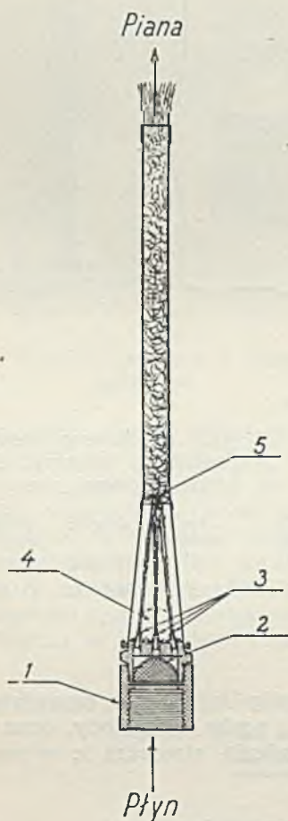
Rys. 8. Prądownica na mieszankę pianolową. 1. Półłącznik śrubowy. 2. Siłko. 3. Dysze. 4. Otwór powietrzny. 5. Zderzenie strumieni.
