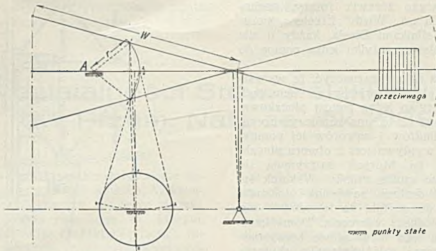
Rys. 21. Schematyczny szkic pompy „Wirth'a“.
