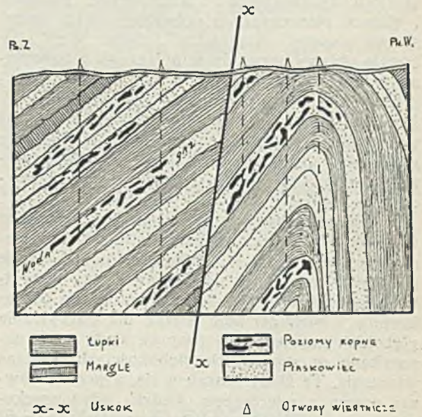
Rys. 2. Przekrój schematyczny złóż ropnych rozdzielonych uskokiem.
