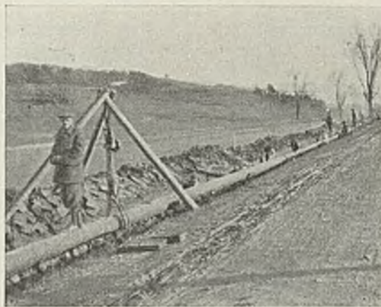
Rys. 4. Budowa gazociągów.
