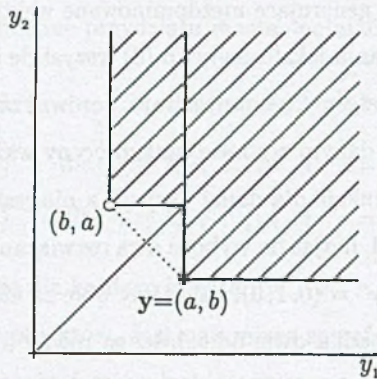
Rys. 1. Struktura dominacji symetrycznej w R^2
