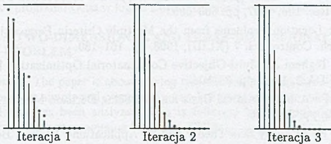
Rys. 2. Wyniki interaktywnej analizy problemu lokalizacyjnego Fig. 2. Results of interactive analysis for location problem
