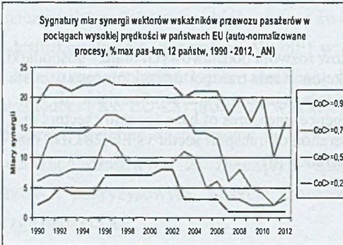
Rys. 4. Sygnatury miar synergii (zbieżności) wskaźników przewozów w modach transportu USA (a; b), UE-28 (c, d, e) i RF (f)
