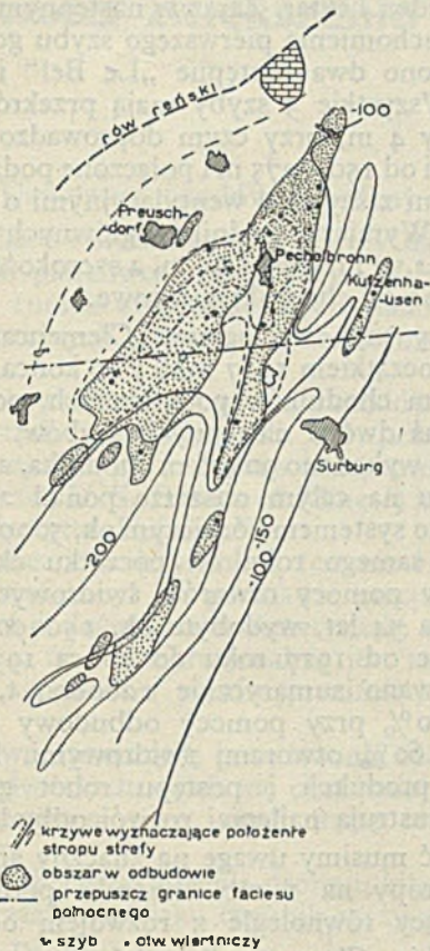
Rys. 1. Obszar Naftowy Alzacji Dolnej
