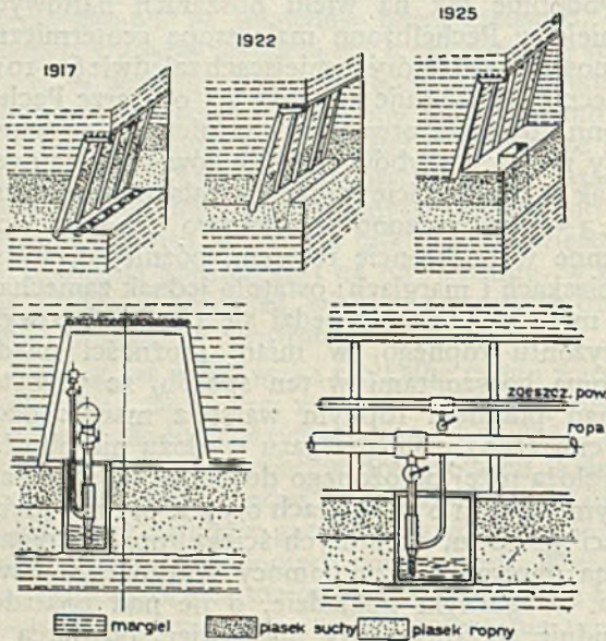
Rys. 3. Zmiany sposobu eksploatacji plasku roponośnego w Pechelbronn
