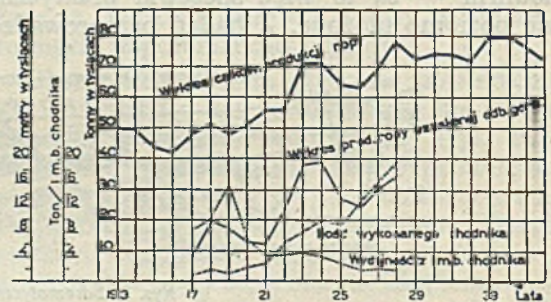
Rys. 4. Produkcja w Pechelbronn
