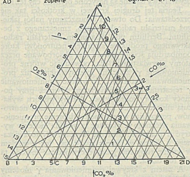
Rys. 2. Trójkąt Gibbs'a dla \text{CH}_4
