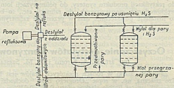
Rys. 2. Schemat włączenia filtrów z dolomitu
