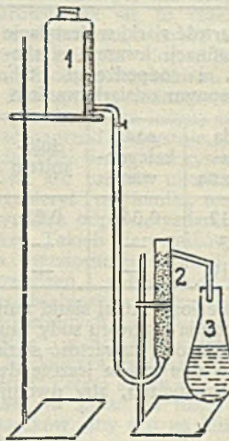
1. Słój, 2. Filtr dolomitowy, 3. Odbiernik benzyny Rys. 1
