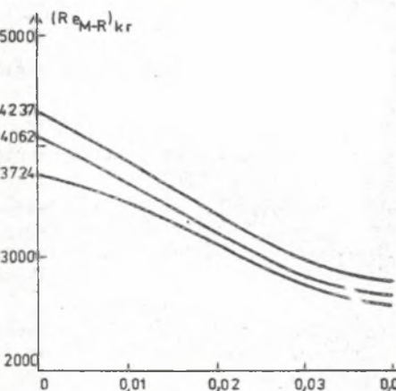
Rys.3 Zmiana (Re_{M-R})_{kr} w funkcji uogólnionej liczby Br
