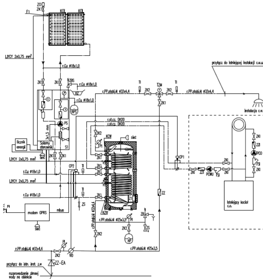
Rys.1.Schemat instalacji solarnej małej mocy [3].
