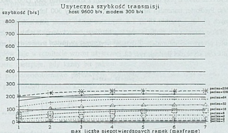
Rys. 11. Wpływ liczby potwierżeń na użyteczną szybkość transmisji (300 bd) Fig. 11. Acknowledgement number influence upon useful transmission speed (300 bd)
