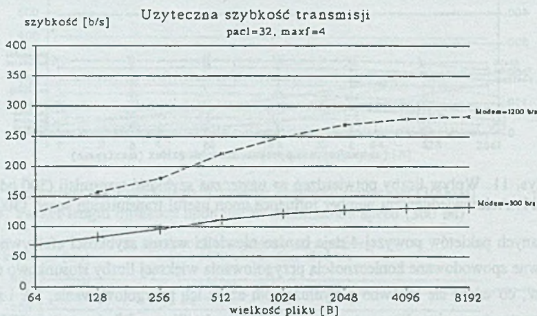
Rys. 12. Wpływ wielkości przesyłanej informacji na użyteczną szybkość transmisji Fig. 12. Transmitted information size influence upon useful transmission speed
