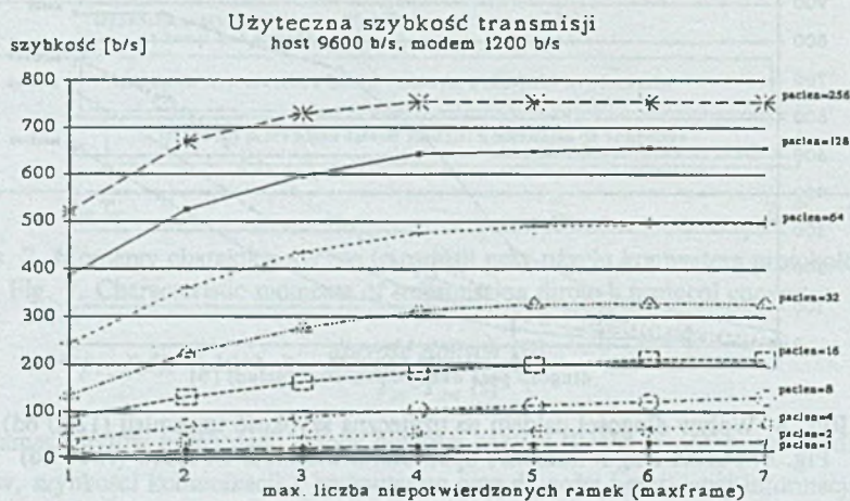
Rys. 10. Wpływ liczby potwierdzeń na użyteczną szybkość transmisji (1200 bd)
