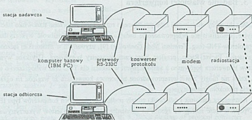
Rys. 6. Konfiguracja stanowiska badawczego Fig. 6. Research stand configuration
