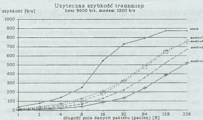
Rys. 8. Wpływ długości pakietu na użyteczną szybkość transmisji (1200 bd)
