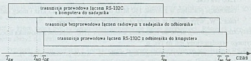
Rys. 7. Momenty charakterystyczne transmisji przy użyciu konwertera protokołów Fig. 7. Characteristic moments of transmission through protocol converter
