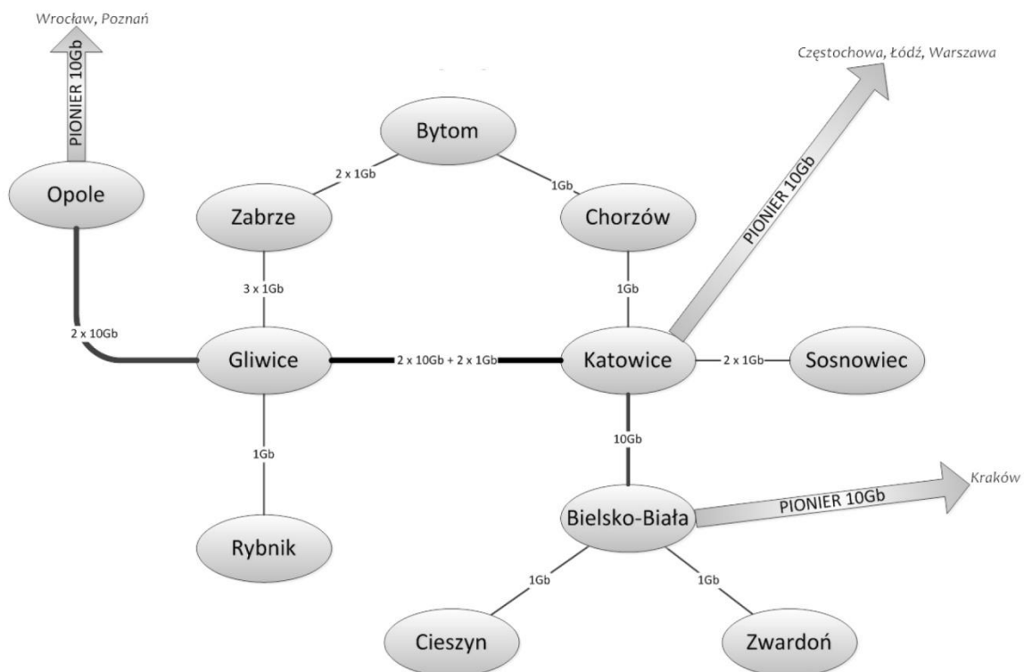
Rysunek 25. Struktura łączy światłowodowych szkieletu ŚASK
