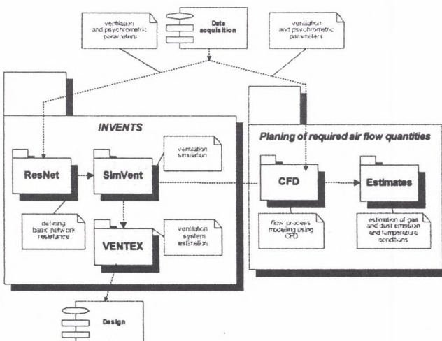
Fig.3. Architecture of the hybrid system INVENTS Rys.3. Schemat blokowy układu hybrydowego INVENTS
