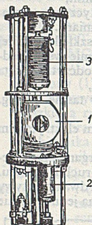
Rys. 9. Teleklinometr Schlumbergera
