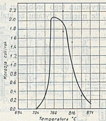
Rys. 11. Postęp korozji stali nierdzewnej 304 spowodowanej ciężką benzyną Refugio
