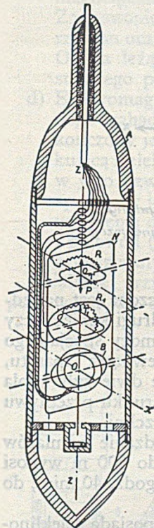
Rys. 7. Aparat Babukowa-Szczurowa
