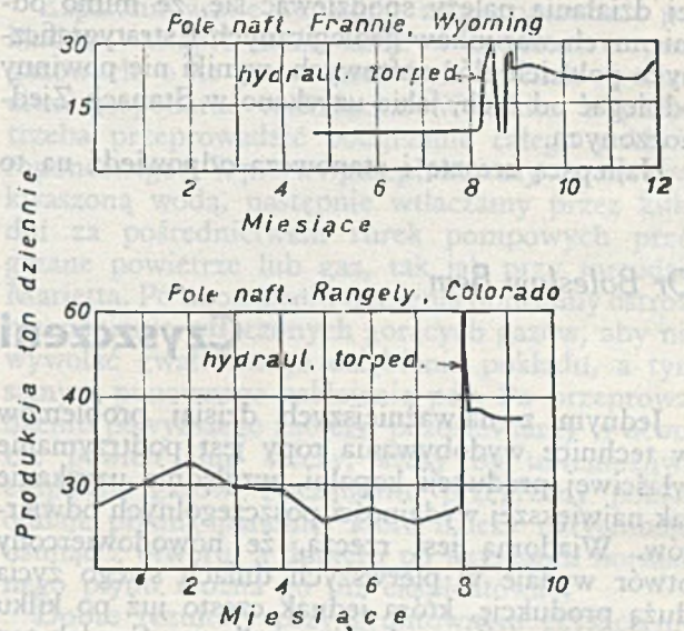
Rys. 4. Wykresy produkcji
