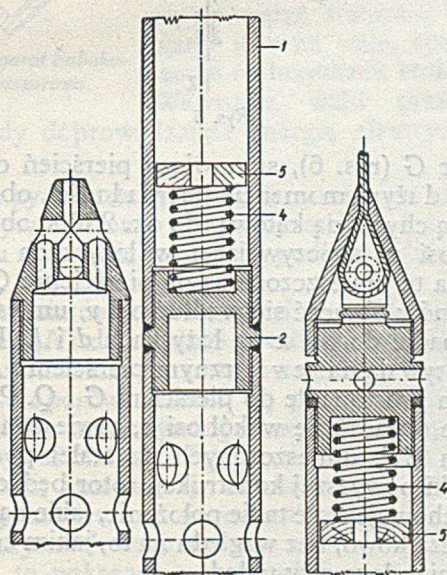
Rys. 2. Aparat Petrosiana - osłona
