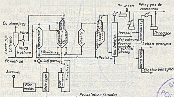
Rys. 8. Urządzenie krakingowe „Fluid Catalyst”
