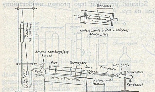
Rys. 10. Aparat do prób korozyjnych
