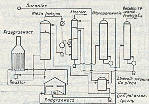
Rys. 9. Urządzenie do otrzymywania butadienu
