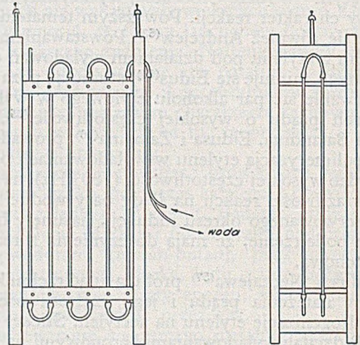
Rys. 3. Opornica wodna Mościckiego
