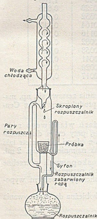
Rys. 2. Aparat Soxhleta
