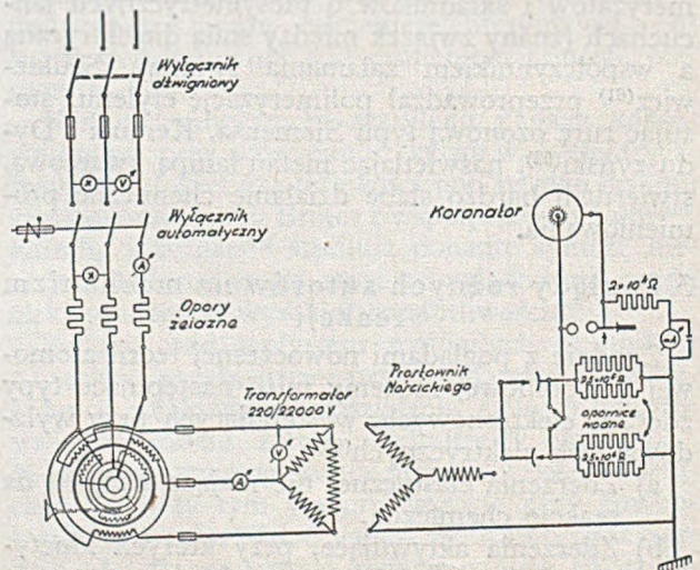
Rys. 4. Układ połączeń do wyładowań koronowych
