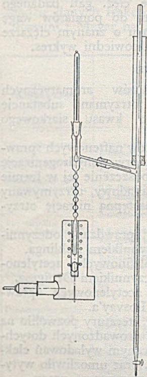
Rys. 10. Aparat do pół-mikro destylacji
