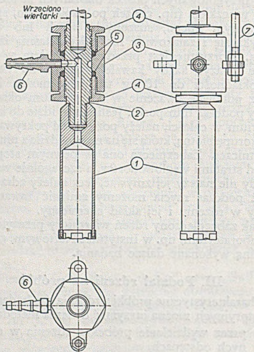
1-wiertło diamentowe, 2-przedłużenie wrzeczona, 3-łożysko dławikowe, 4-śruby dławikowe, 5-uszczelki, 6-końcówka do węża gumowego, 8-pretły usztywniające
