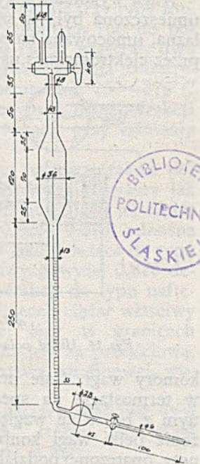
Rys. 12. Zmodyfikowana biureta Bunte'go
