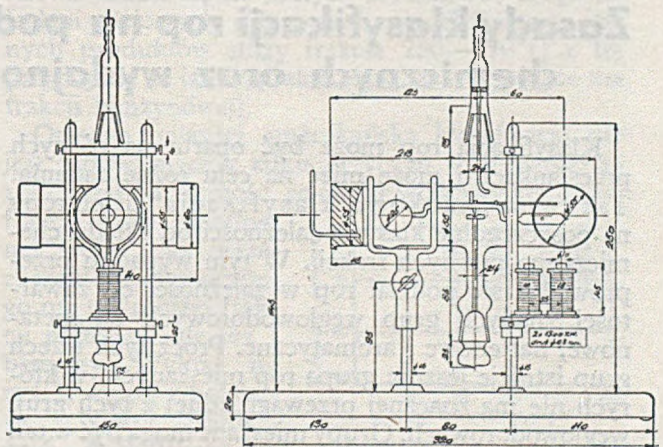
Rys. 13. Elektromagnetyczna waga gazowa
