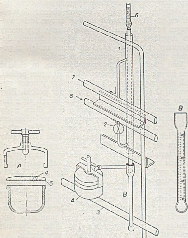
A—retorta, B—menzurka, 1—kondensator, 2—zawór do regul. przepływu wody chłodzącej, 3—doprowadzenie gazu do palnika Bunsena, 4—wkręt dla rurki, 5—płaszczyna styku, 6—chloroform, 7—wypływ wody chłodzącej, 8—wplyw wody chłodzącej
