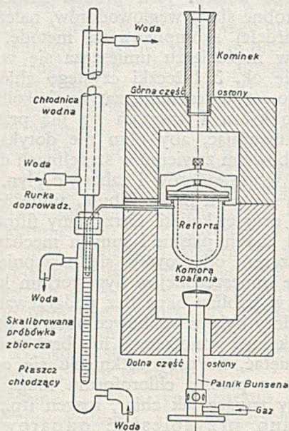
Rys. 4. Aparatura destylacyjna dla określenia zawartości plynów w badanej próbce
